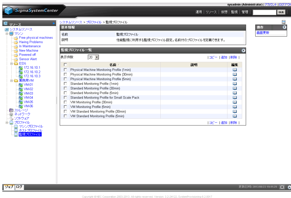
図 52 監視プロファイル一覧
