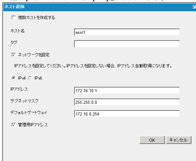
図 29 ホスト追加
