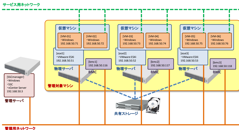
図 2 今回構築するシステムの構成
