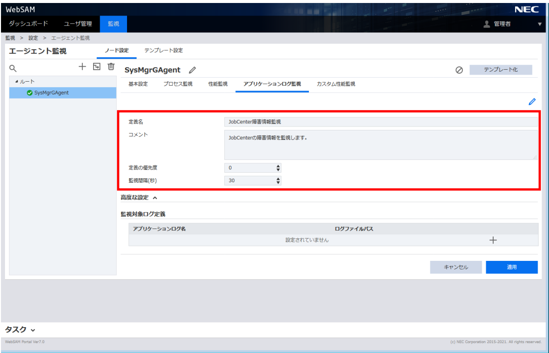
図23.5 アプリケーションログ監視の編集画面
