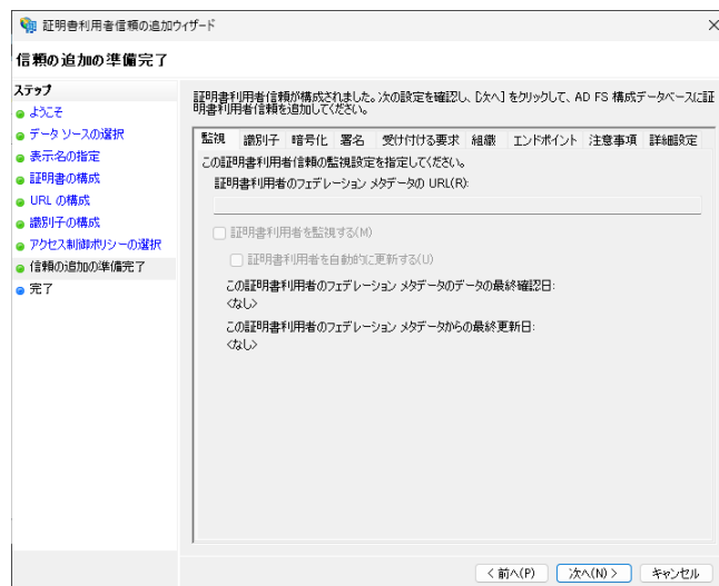
図14.12 証明書利用者信頼の追加ウィザード [信頼の追加の準備完了]画面
