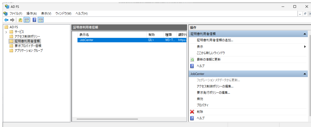
図14.14 ADFS の証明書利用者信頼画面
