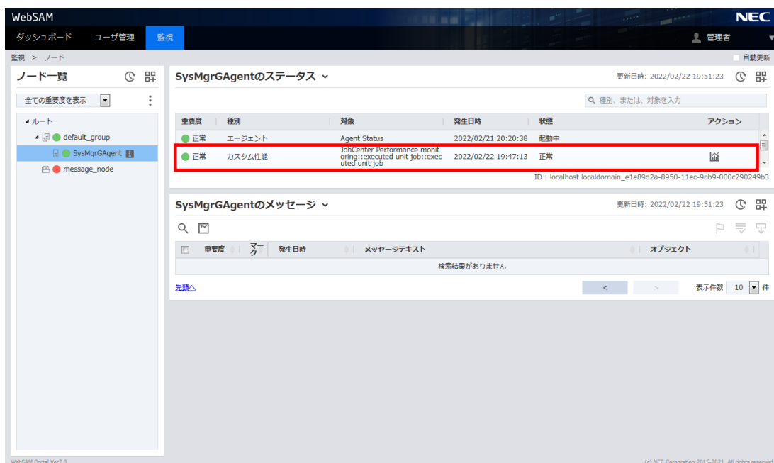
図24.12 SystemManagerGのカスタム性能監視(正常時)
