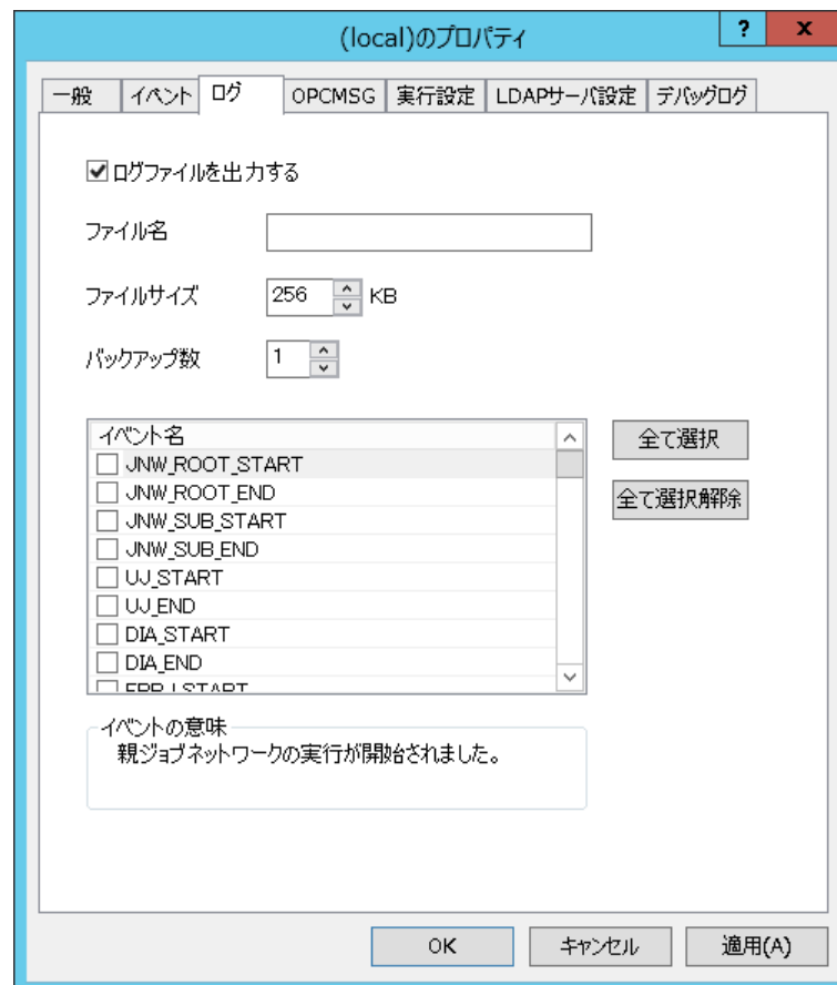
図15.3 ログタブ画面例
