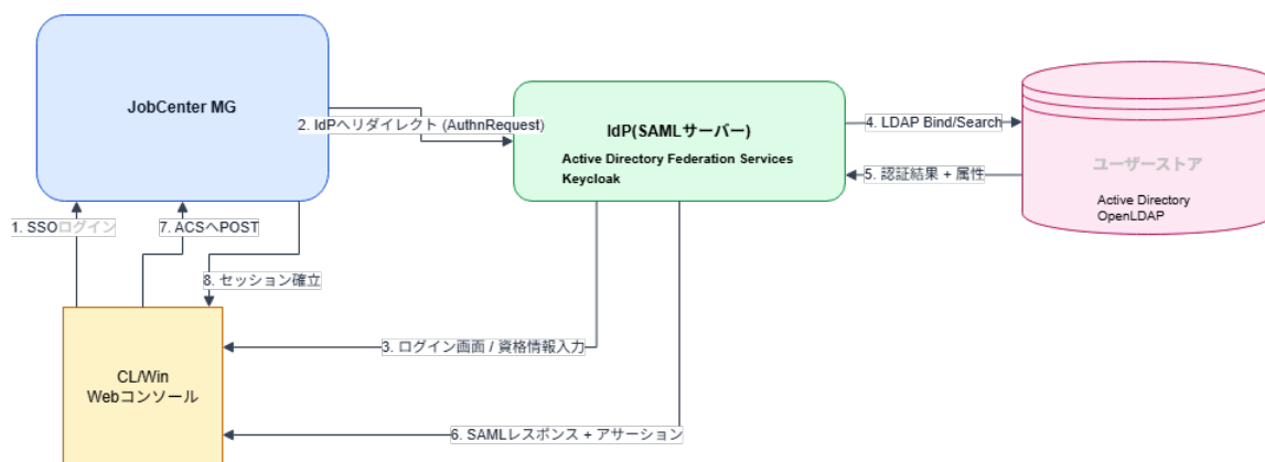
図14.1 LDAP 連携の概要
