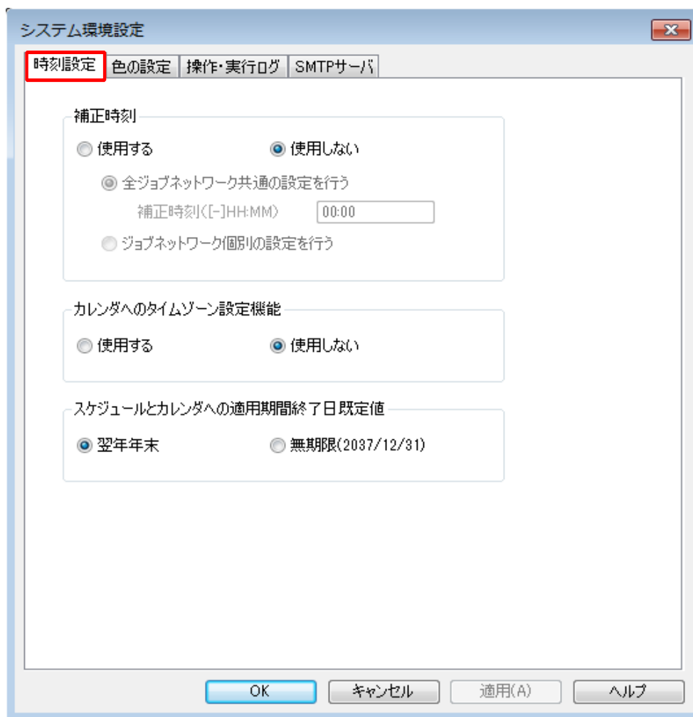
図9.10 〔システム環境設定〕画面例
