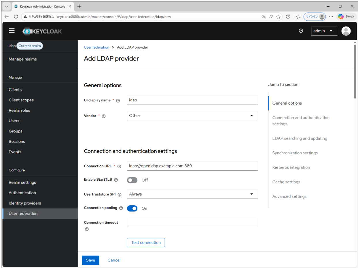
図14.22 Keycloak の Add LDAP provider 画面
