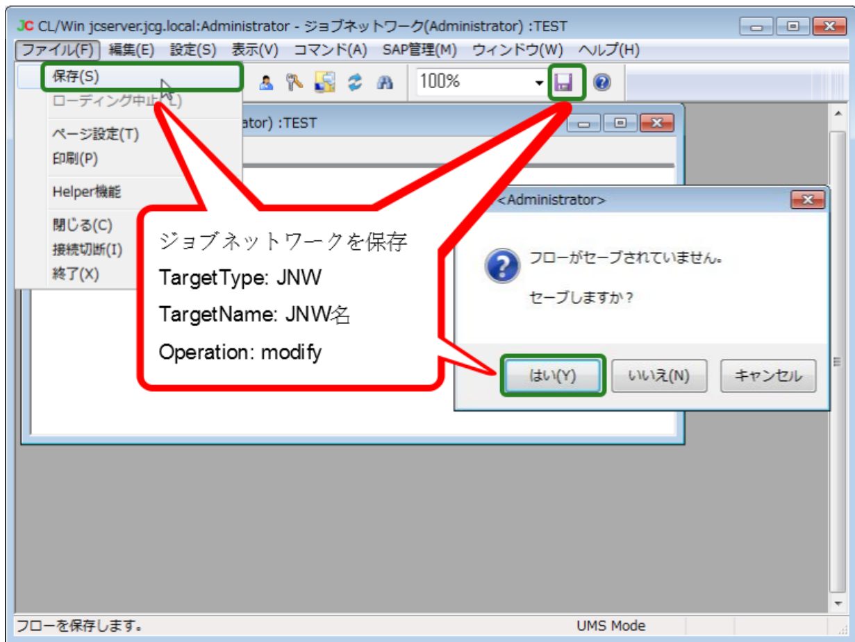
図7.32 ジョブネットワークフローに対する操作
