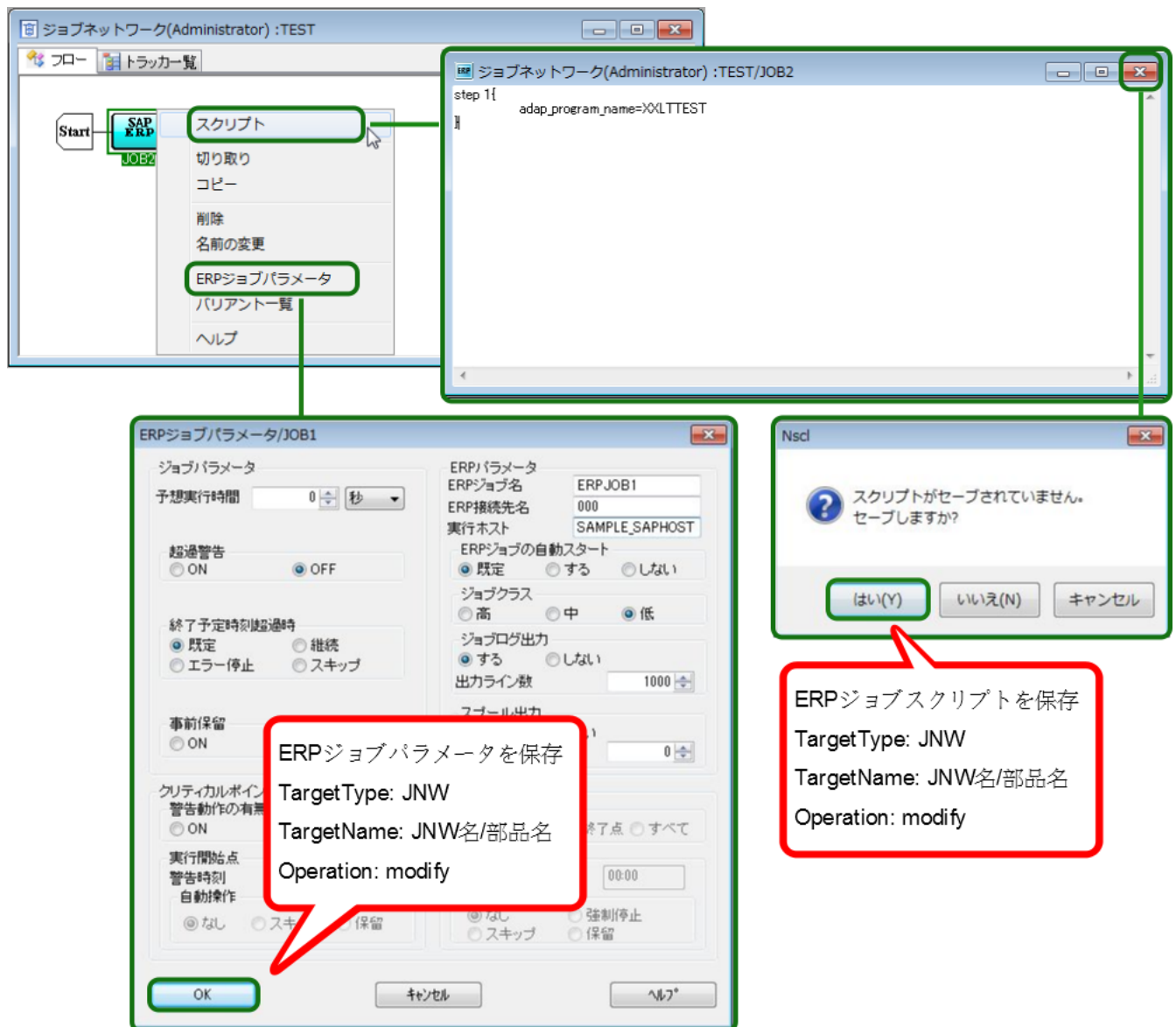
図7.34 ERPジョブに対する操作
