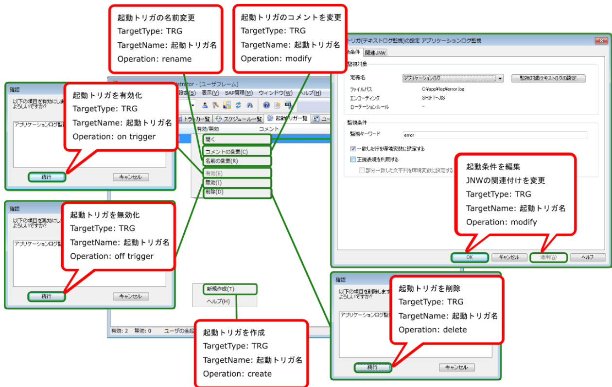
図7.25 起動トリガに対する操作
