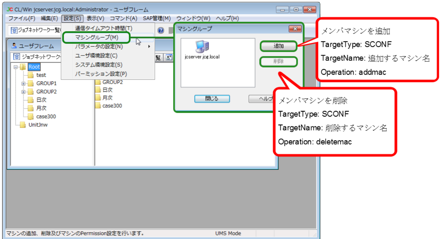
図7.47 マシングループに対する操作
