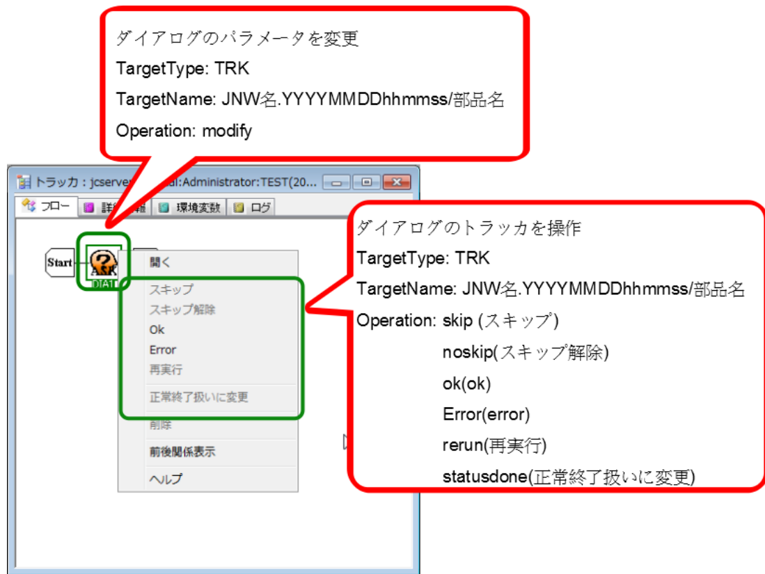
図7.14 ダイアログ部品トラックに対する操作
