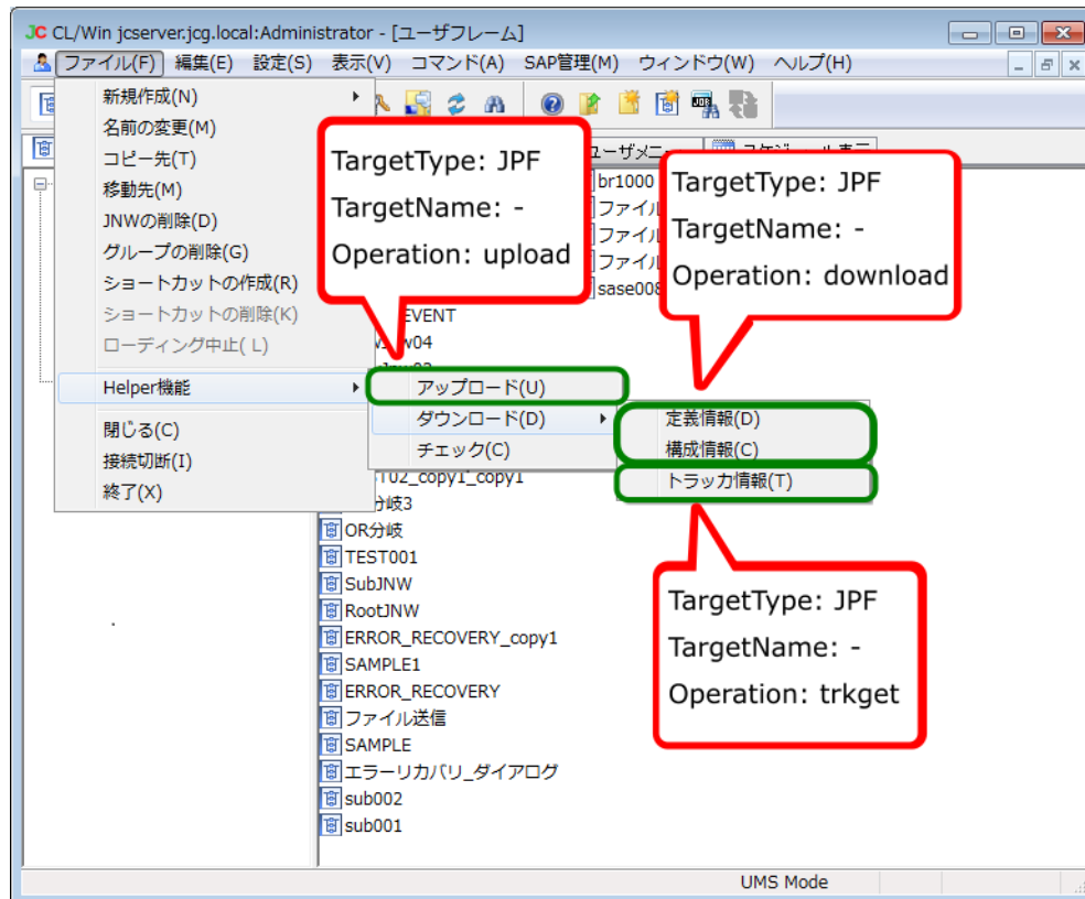
図7.48 JPFのアップロード・ダウンロード
