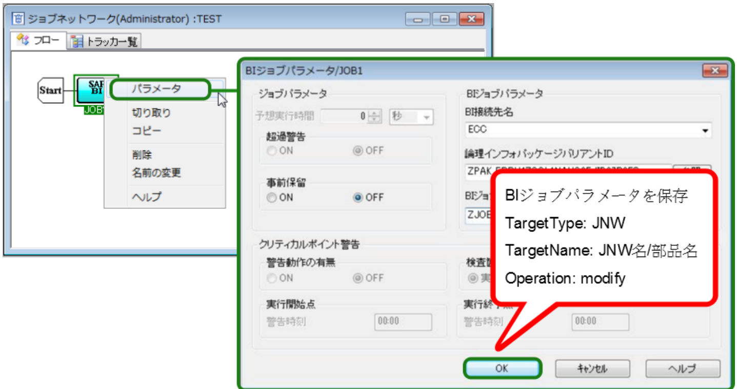
図7.35 BIジョブに対する操作
