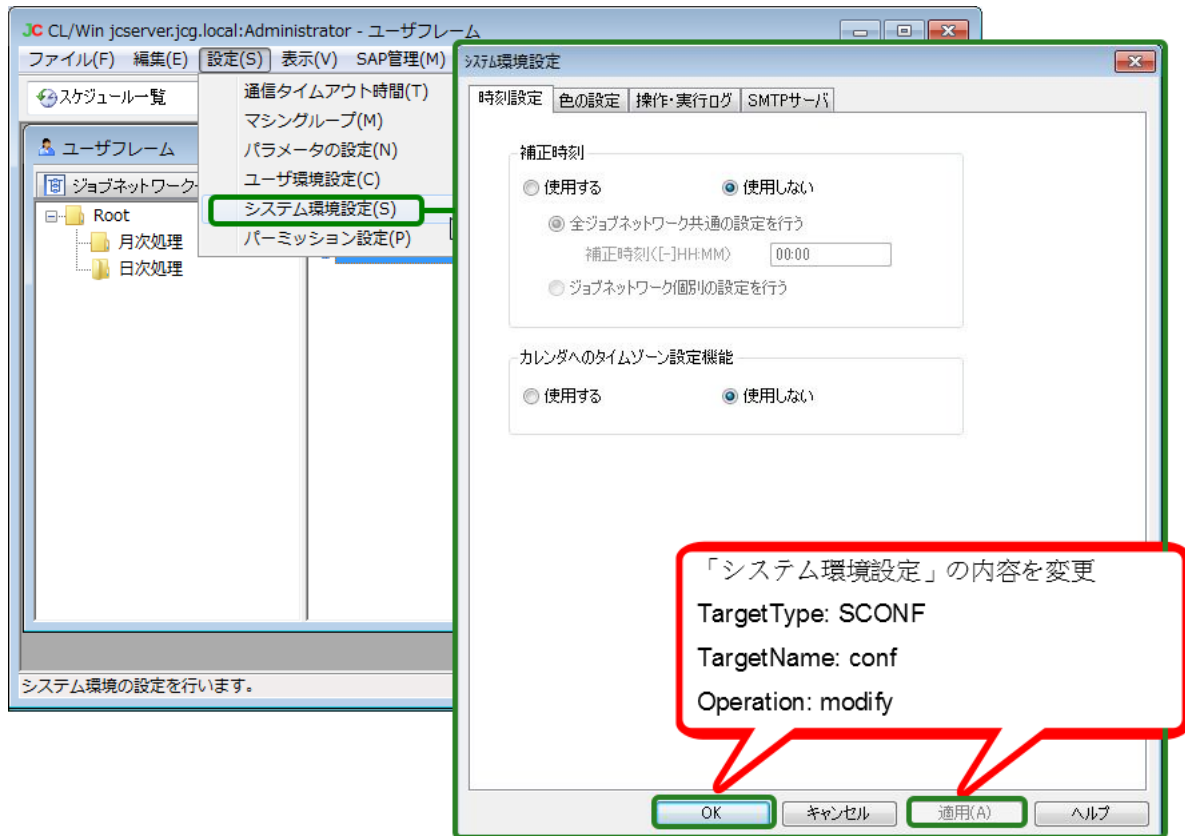
図7.30 システム環境設定に対する操作
