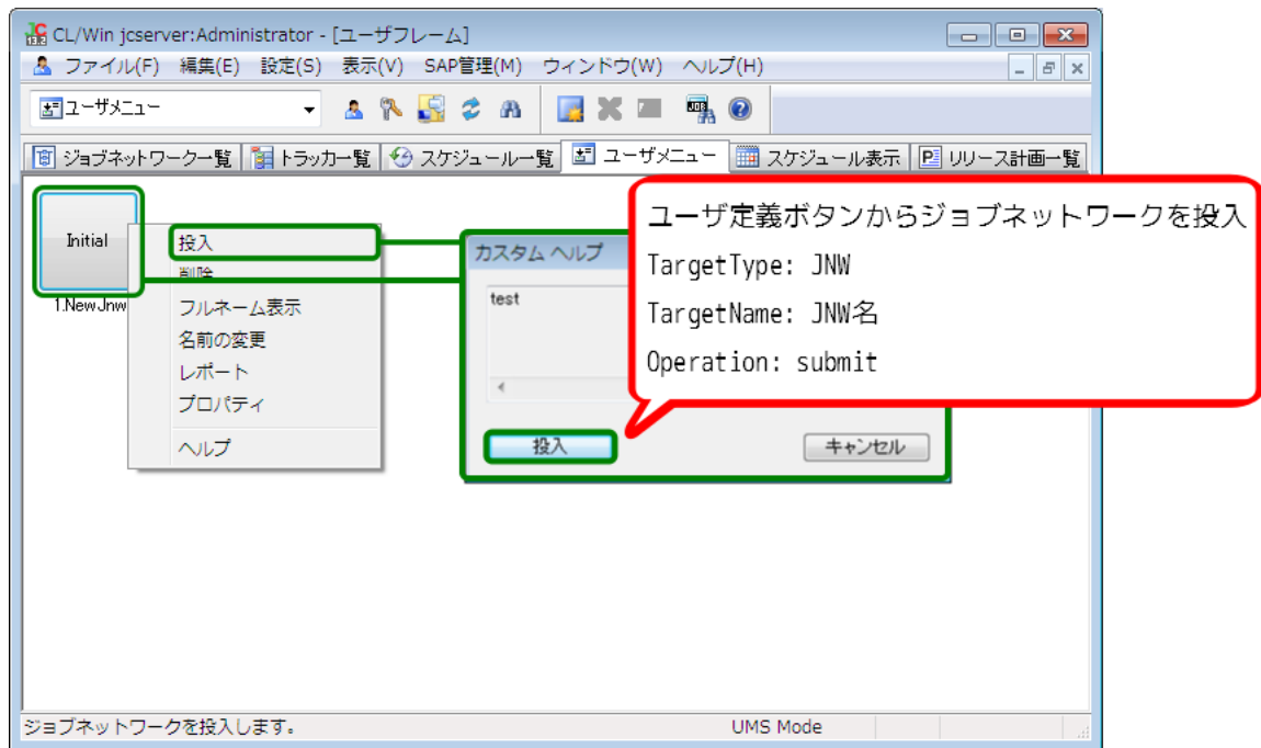
図7.27 ユーザメニューの操作
