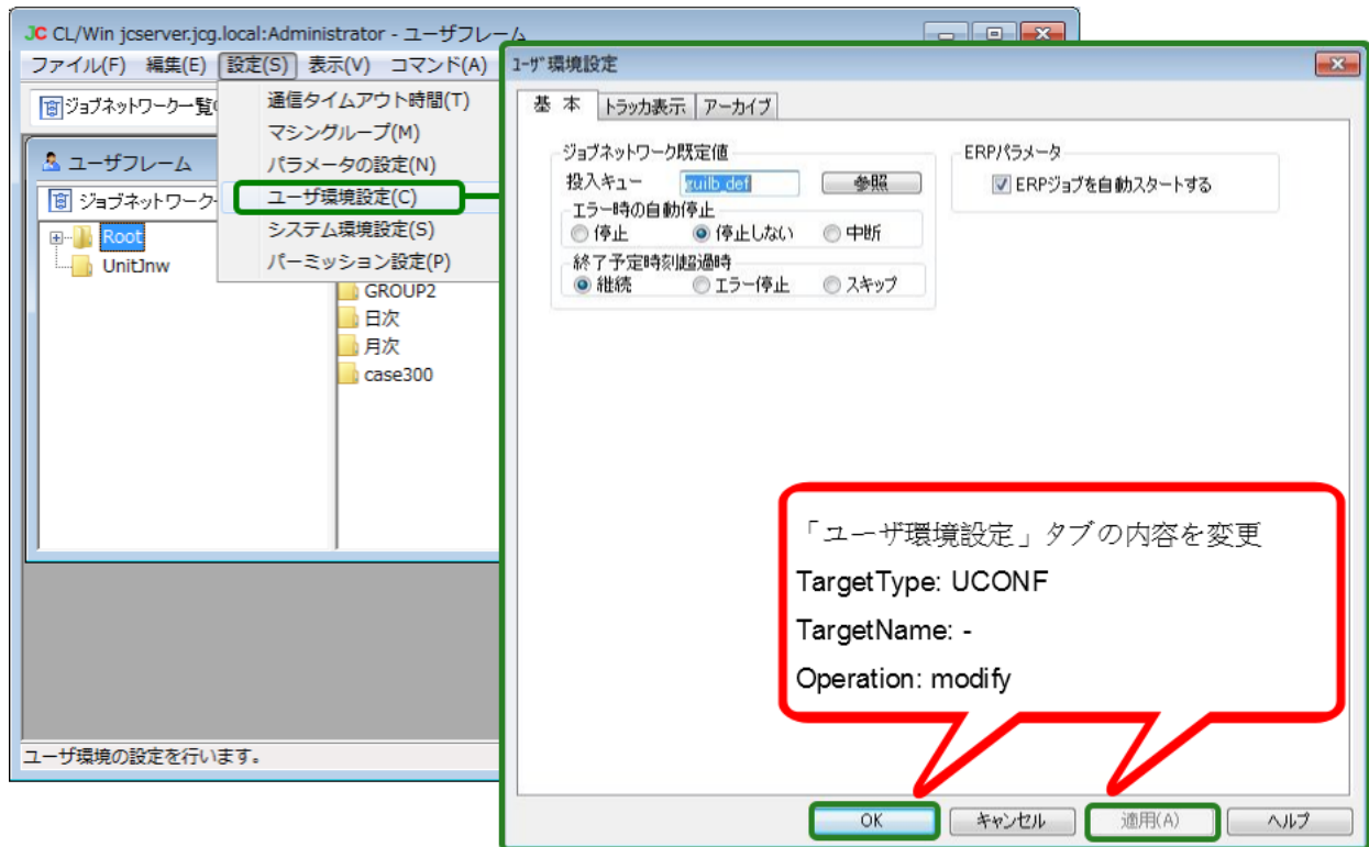
図7.31 ユーザ環境設定に対する操作
