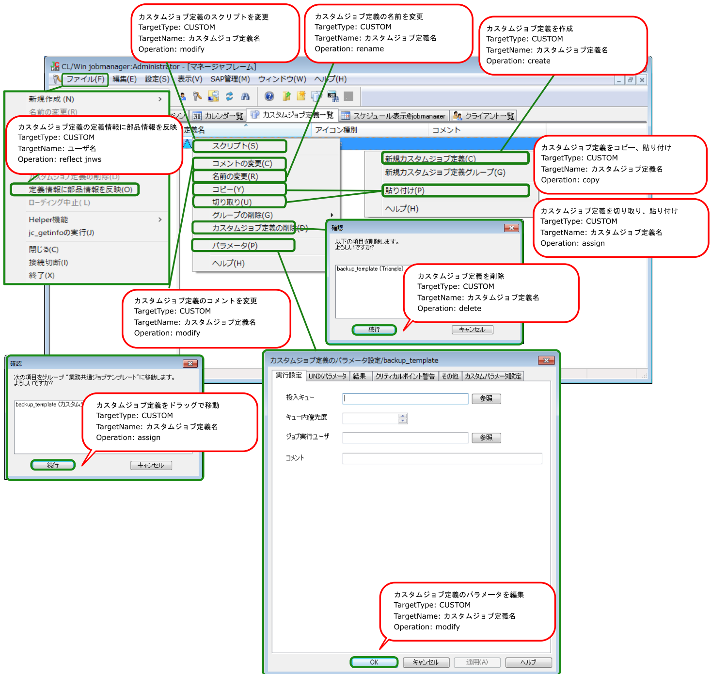
図7.43 カスタムジョブ定義に対する操作
