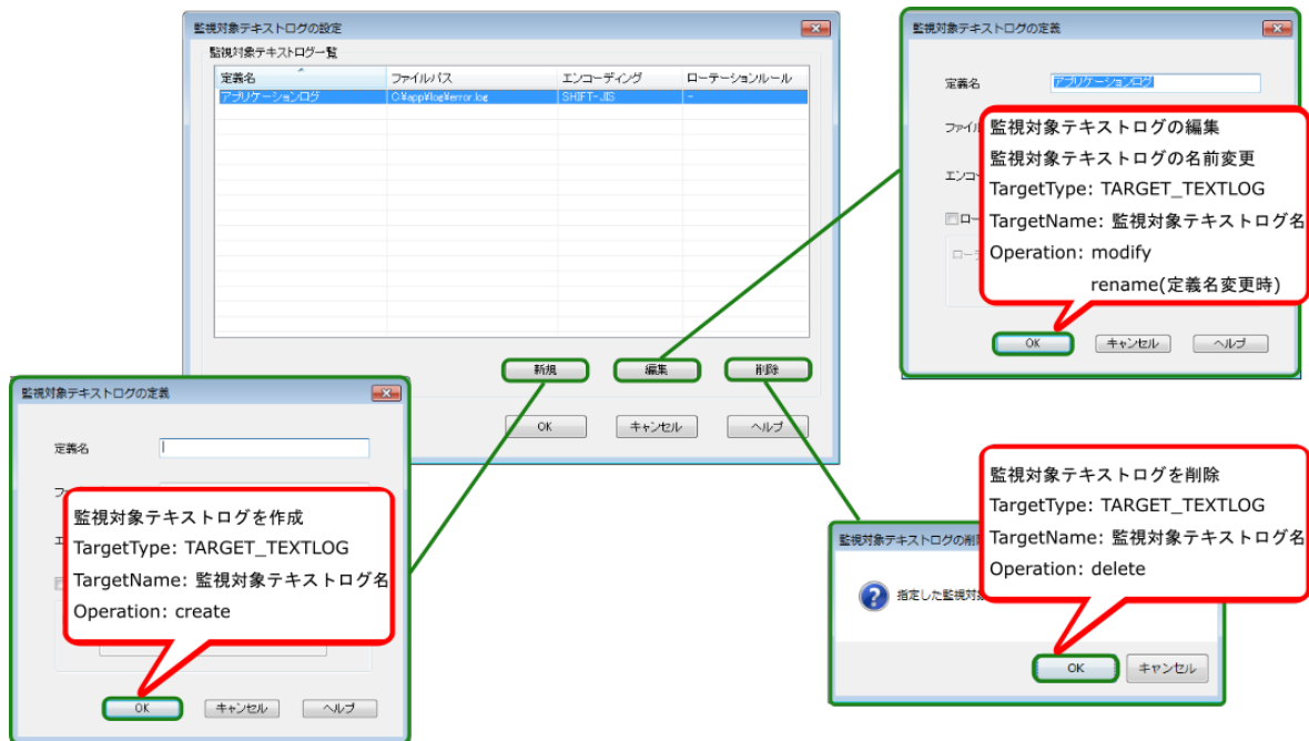
図7.26 監視対象テキストログに対する操作
