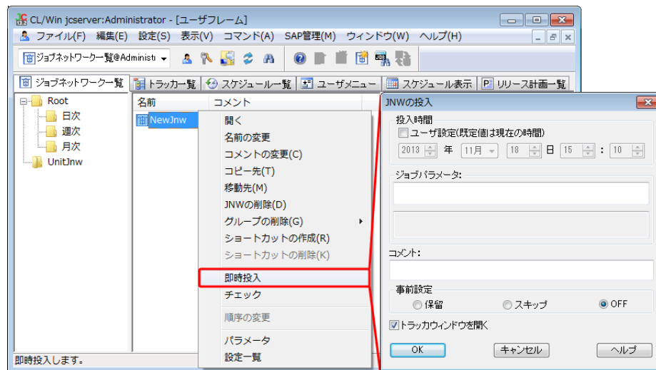
図3.3 即時投入画面例
