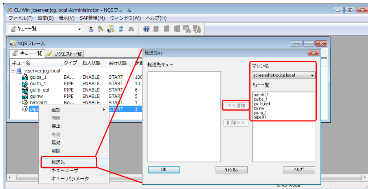
図6.13 転送先キューの指定画面例
