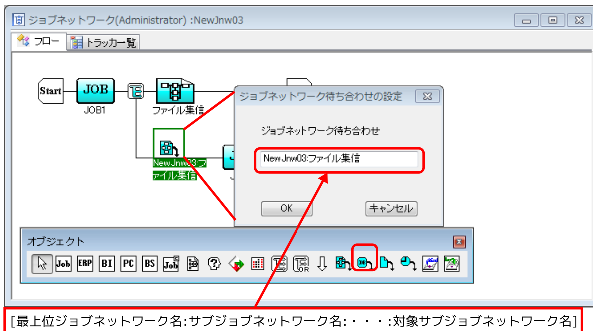
図4.20 ジョブネットワーク待ち合わせの設定例
