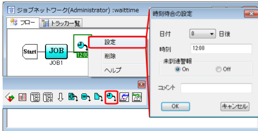
図4.22 時刻待ち合わせの設定画面例
