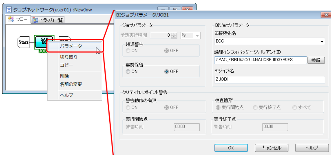
図4.5 BIジョブパラメータの画面例
