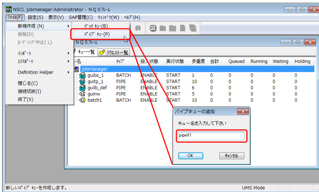
図6.11 パイプキューの追加画面例
