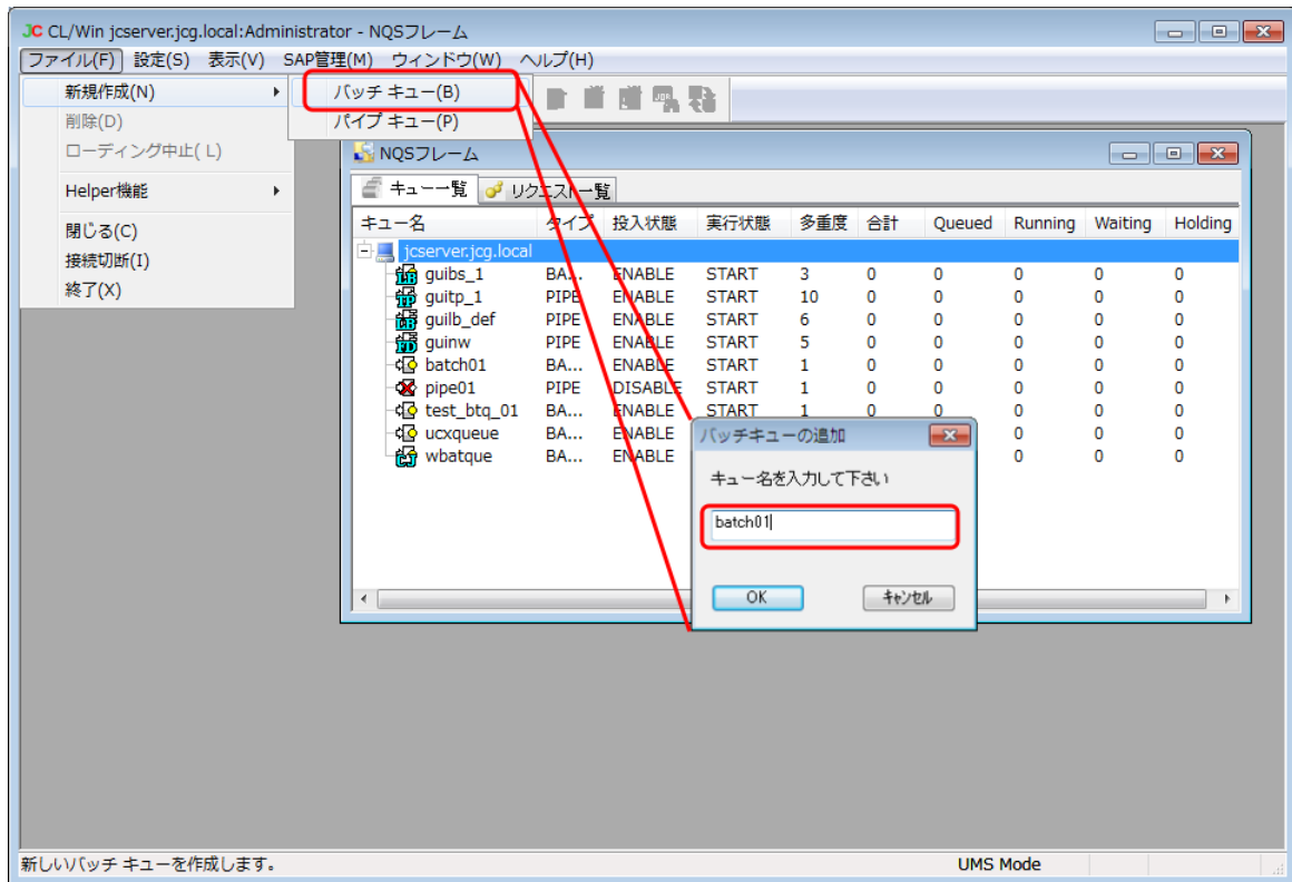
図6.9 バッチキューの作成画面例
