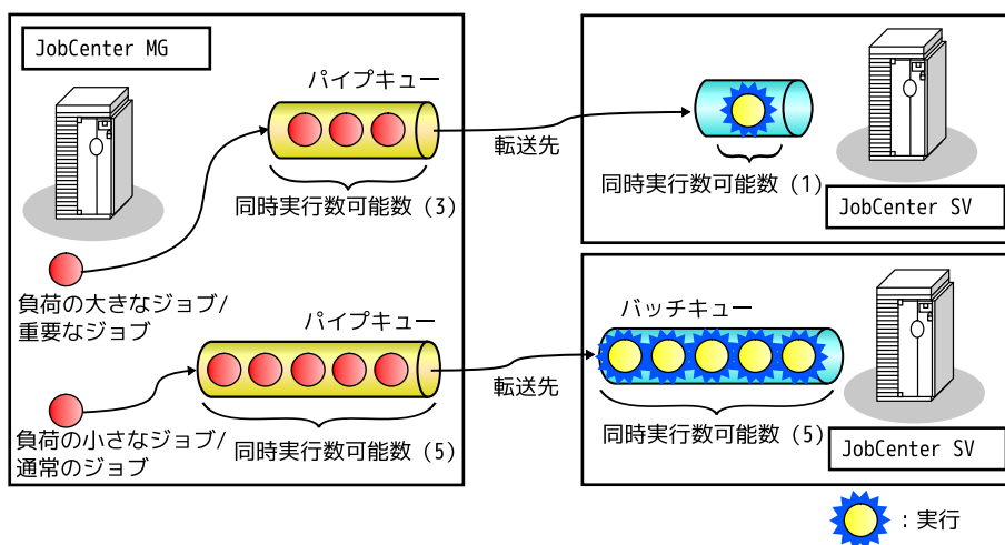
図6.5 ジョブ同時実行制限のイメージ
