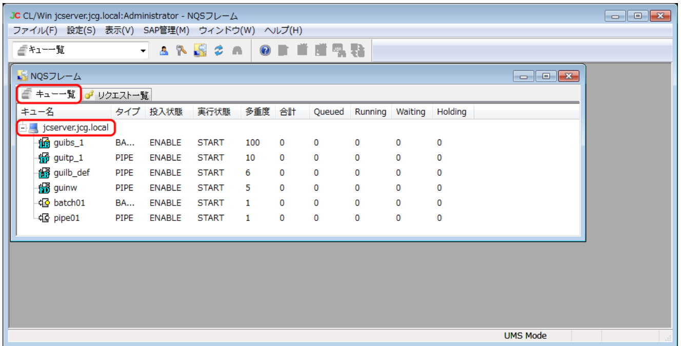
図6.8 [NQSフレーム] - [キュー一覧] 画面例
