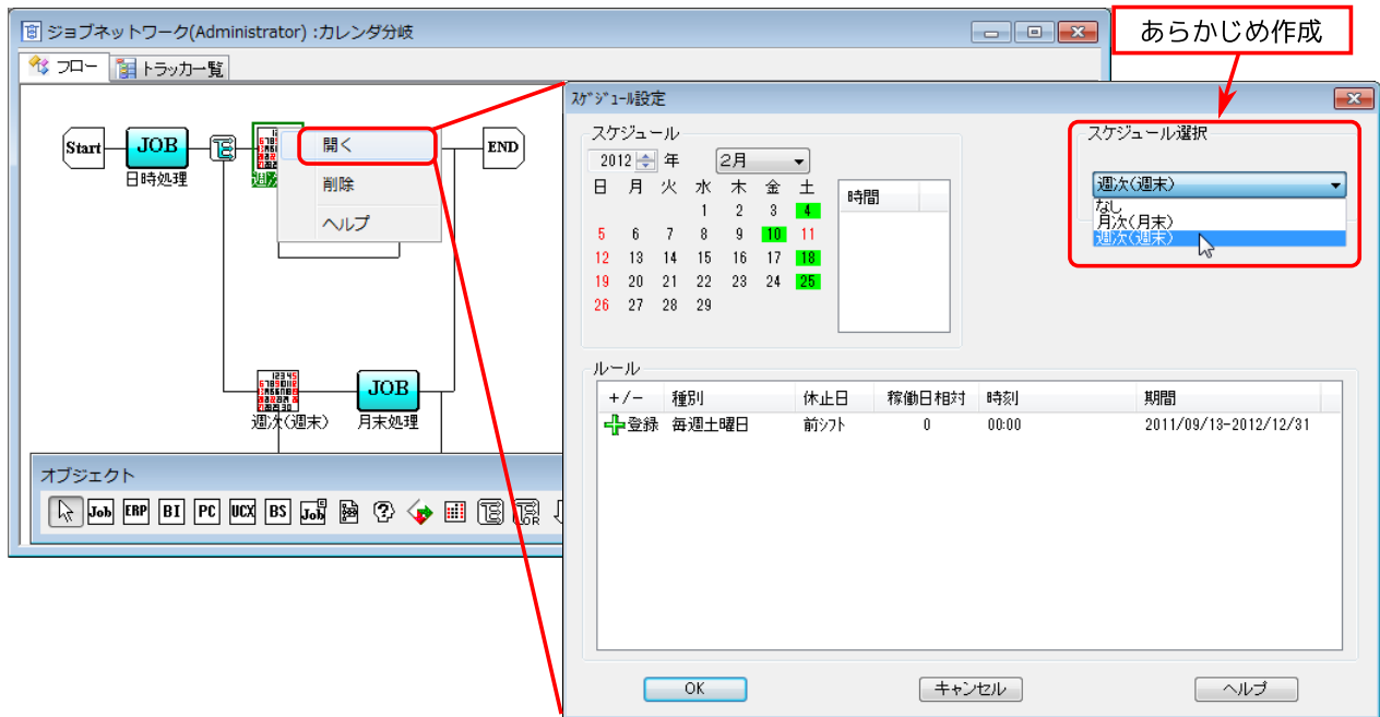
図4.16 スケジュール設定画面例
