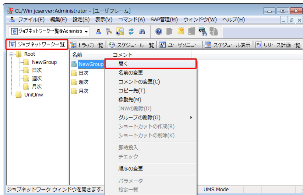
図3.8 グループ内への移動
