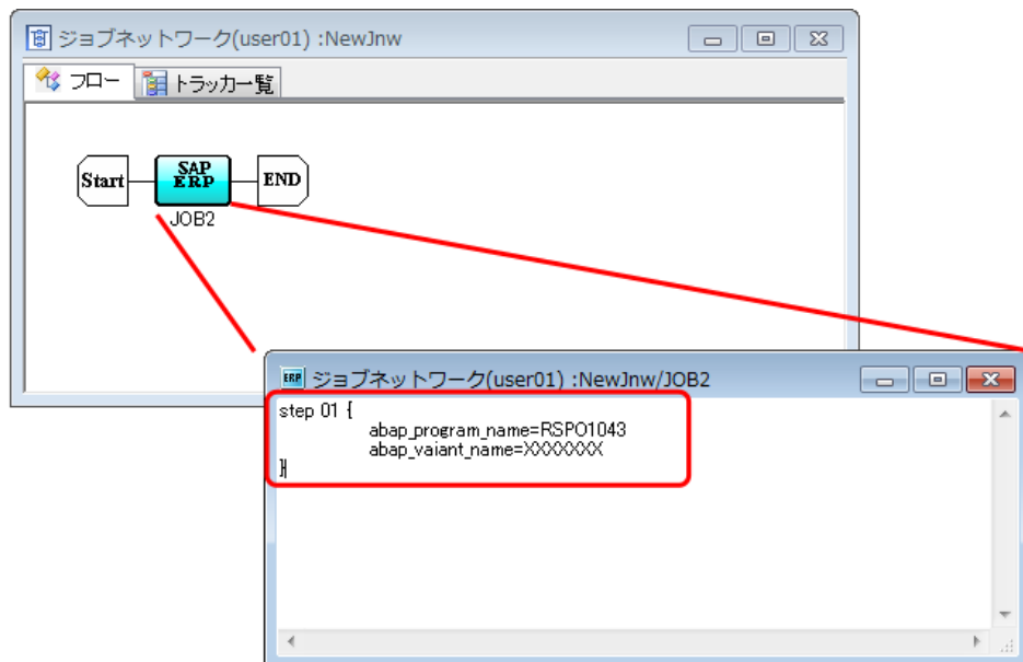
図4.3 ERPジョブのバッチファイル（Windows）の例
