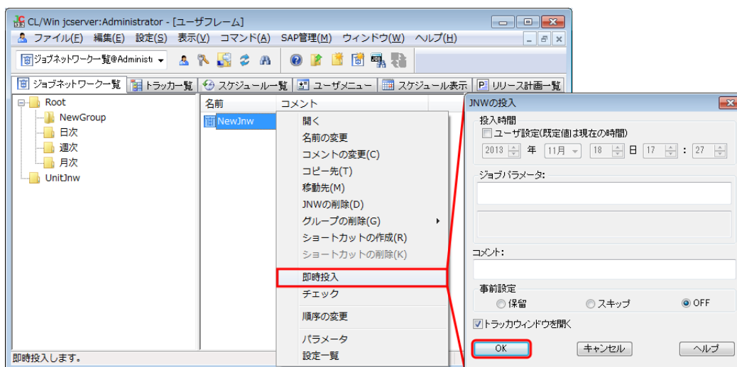
図3.18 即時投入の実行例
