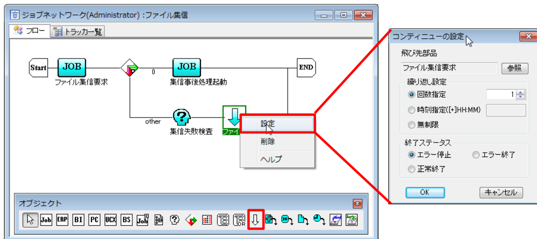
図4.17 コンティニュー部品の設定画面例
