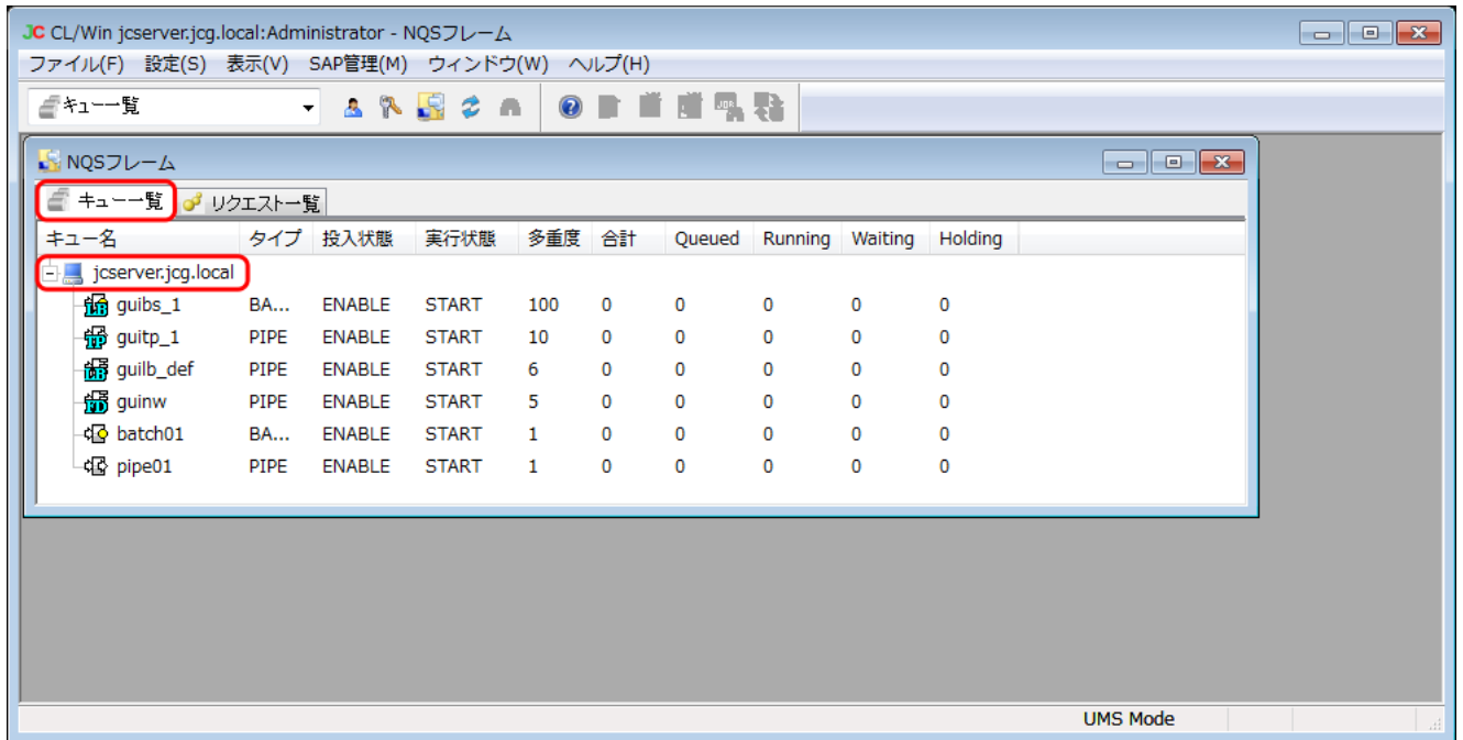
図7.1 [NQSフレーム] – [キュー一覧] 画面例
