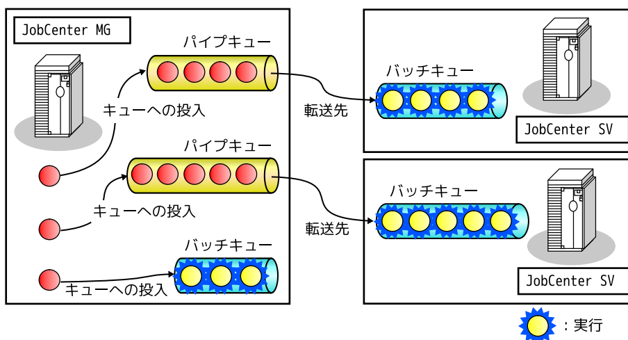
図6.4 ジョブ転送のイメージ
