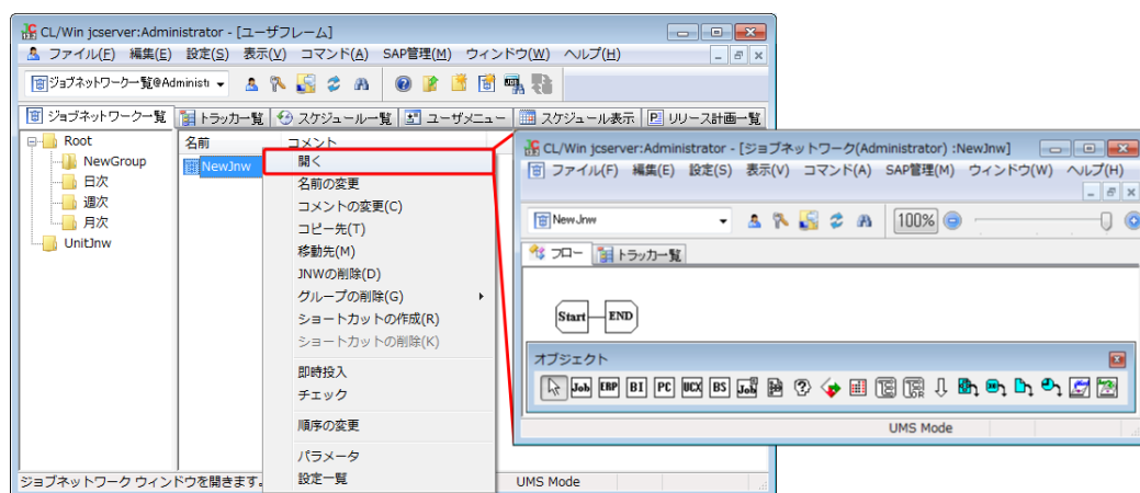
図3.10 ジョブネットワークの表示
