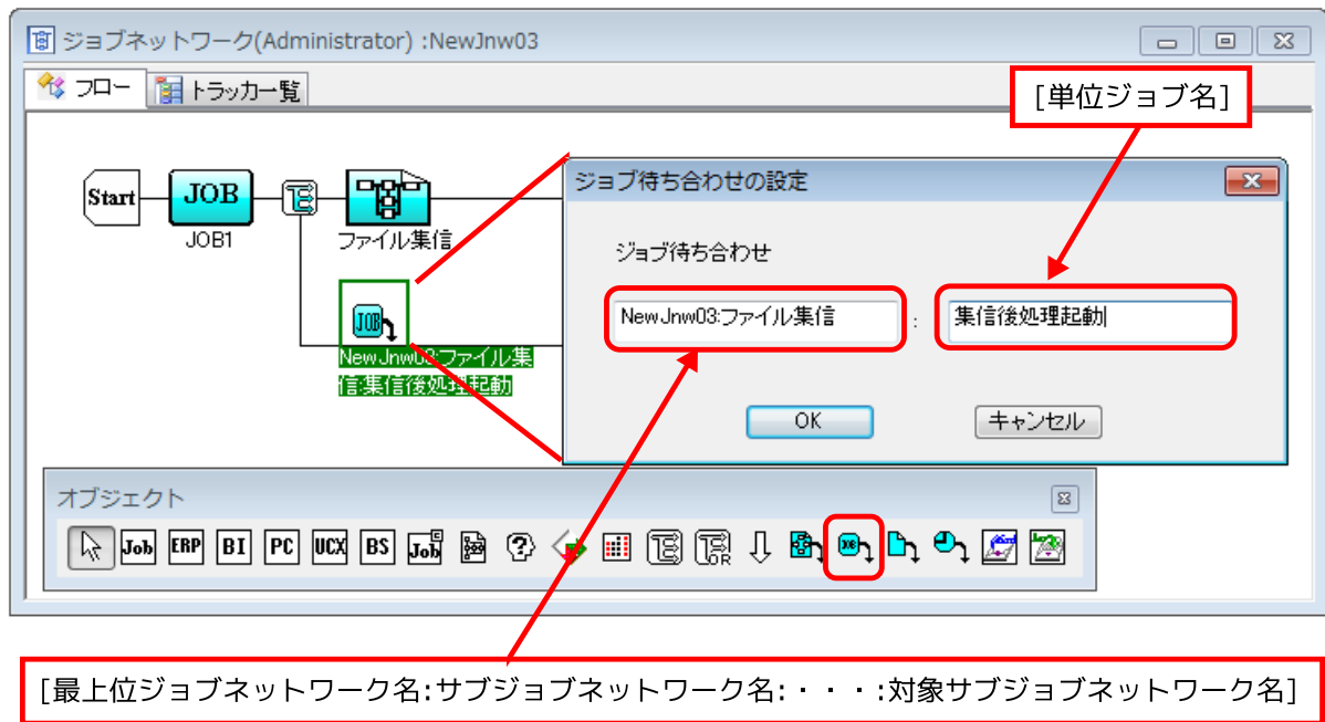
図4.19 ジョブ待ち合わせの設定例
