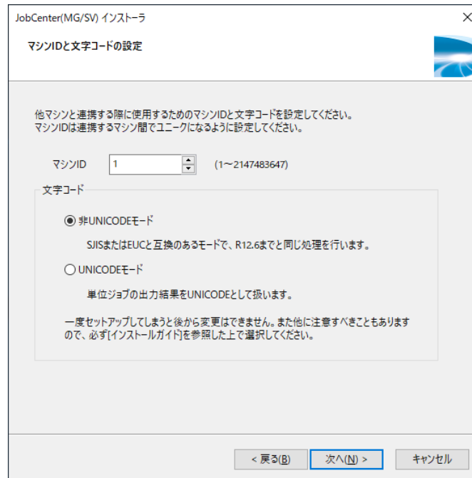
図2.19 マシンIDと文字コードの設定画面
