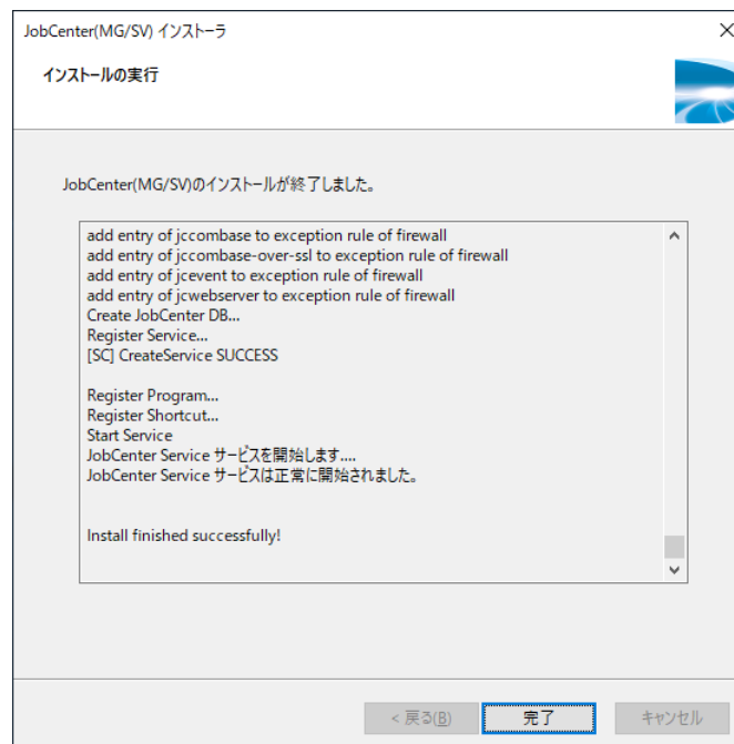
図2.21 インストールの実行画面
