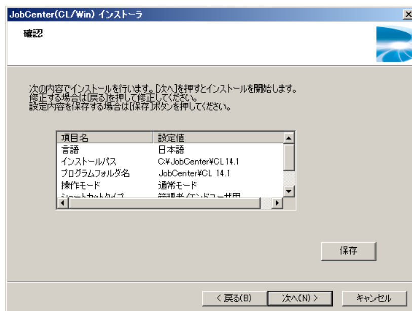
図2.29 確認画面
