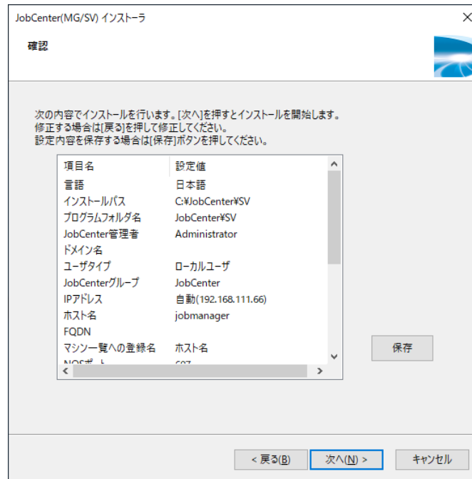
図2.20 確認画面
