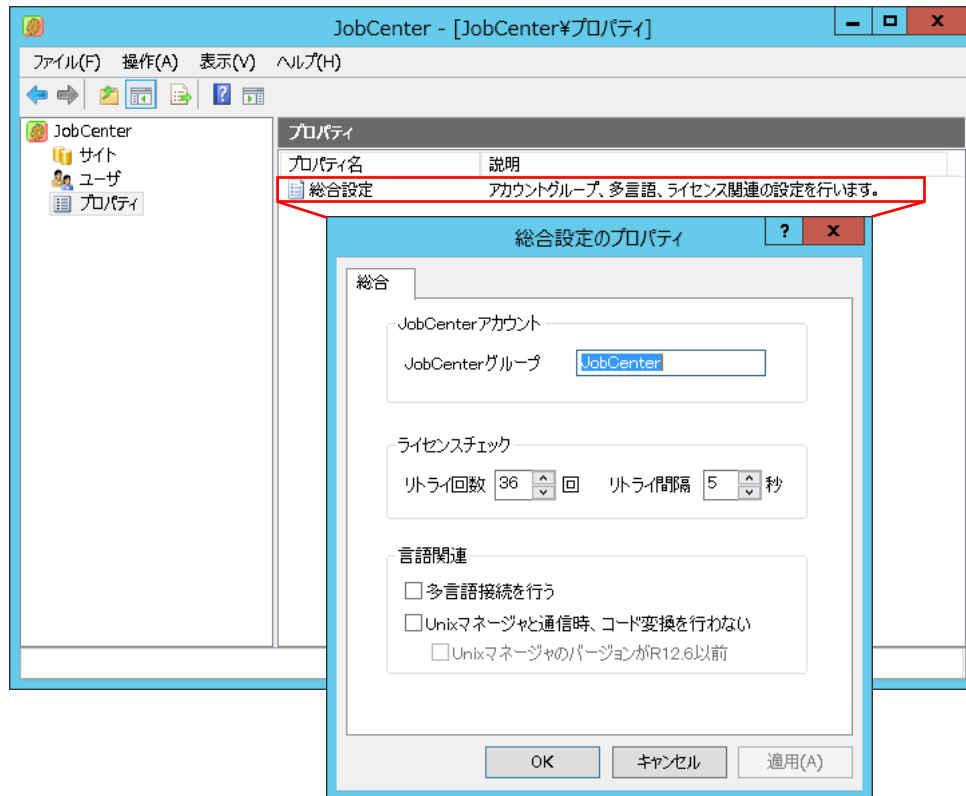
図16.23 総合設定のプロパティ画面例
