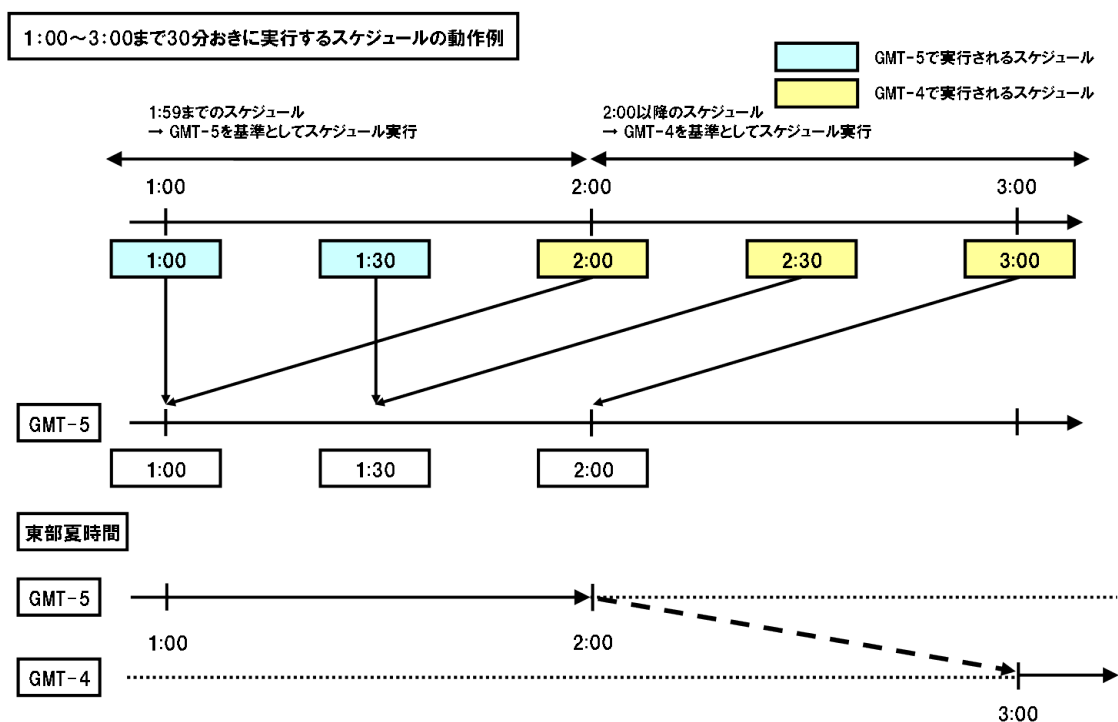
図19.7 夏時間開始時刻周辺での動作例
