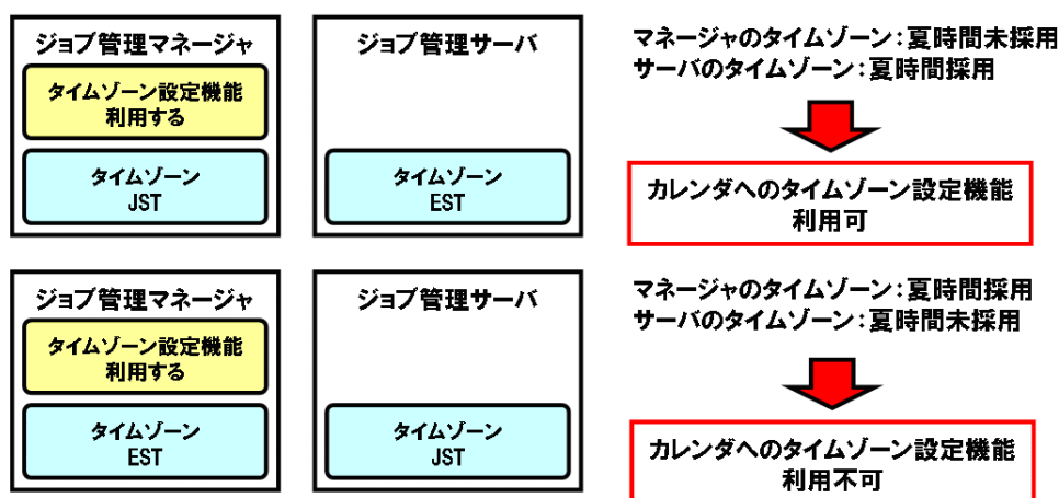
図19.1 カレンダーへのタイムゾーン設定機能の利用条件例
