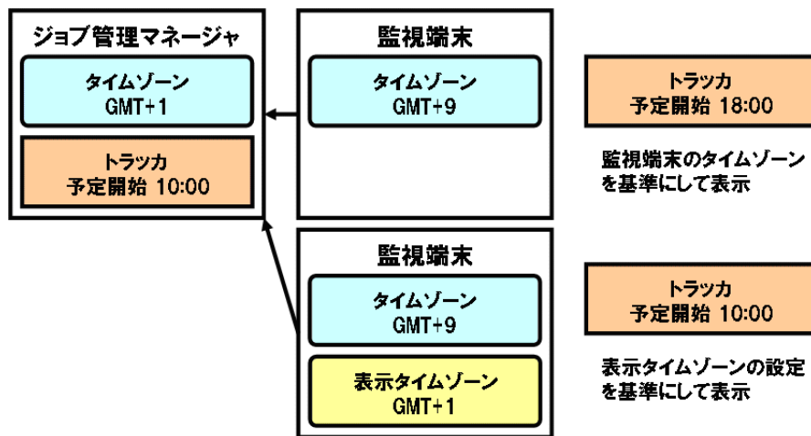
図19.9 表示タイムゾーン変更機能の利用例
