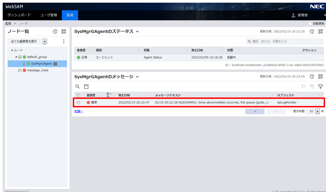
図24.11 SystemManagerGのメッセージ監視
