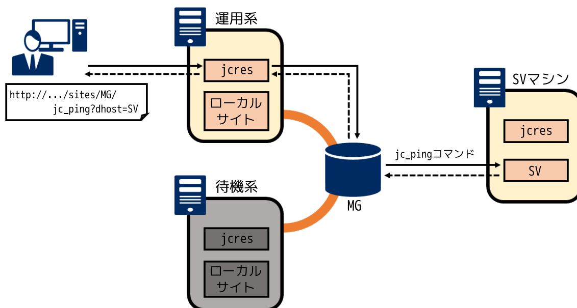
図21.1 MGからSVに対する疎通確認の構成図
