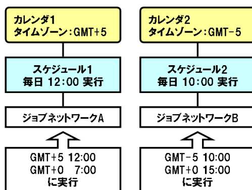
図19.2 カレンダーへのタイムゾーン設定機能の動作イメージ
