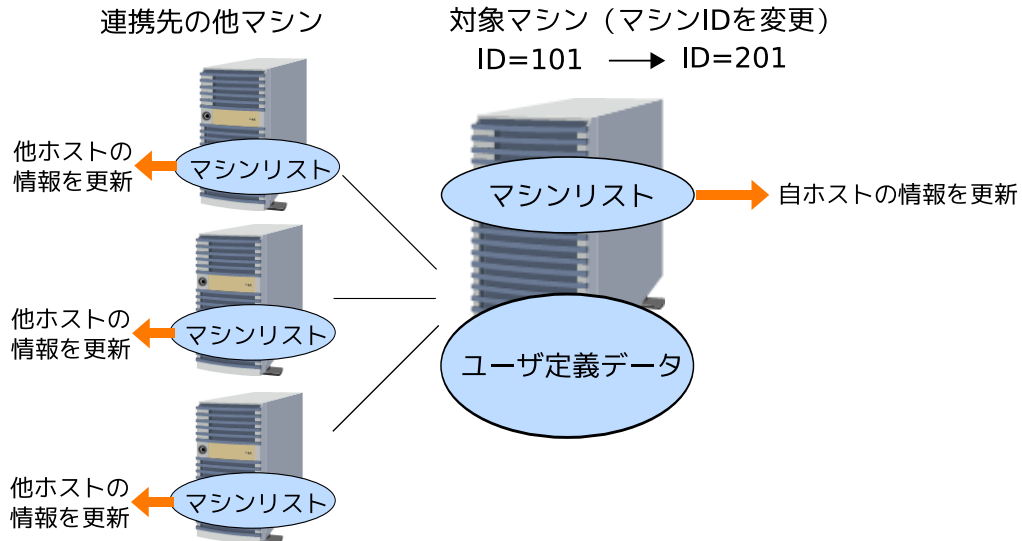
図17.5 マシンIDの変更
