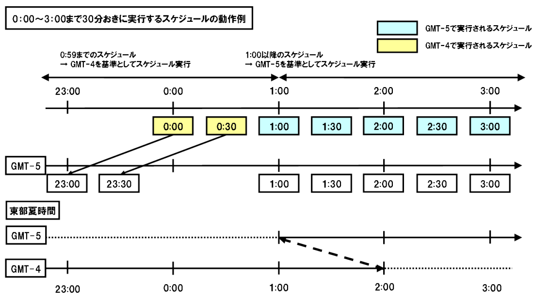
図19.8 夏時間終了時刻での動作例
