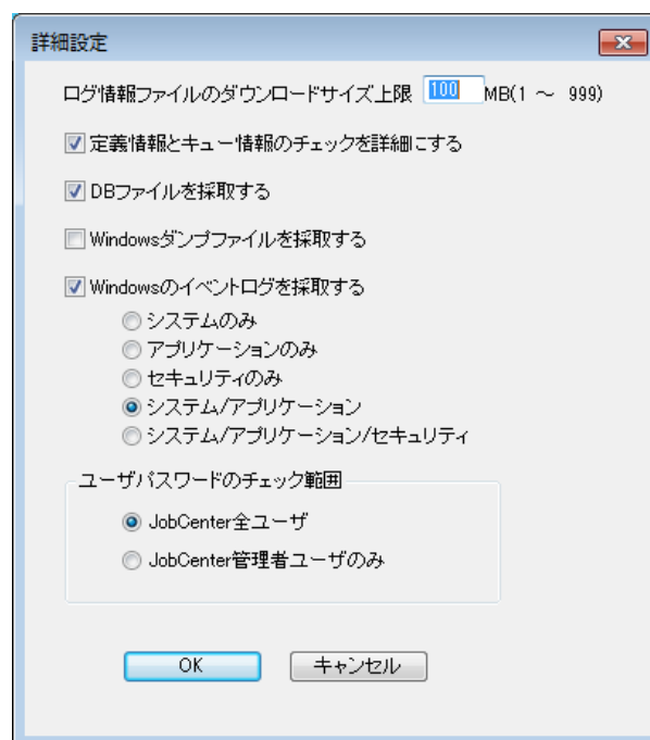
図28.6 jc_getinfoの詳細設定画面 (Windows版JobCenter MG/SV の場合)
