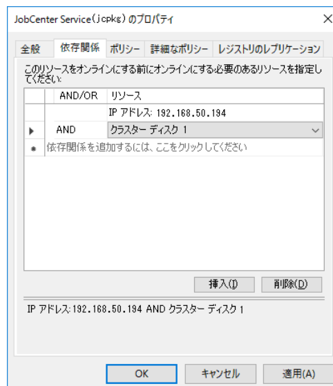
図5.8 依存関係設定画面例
