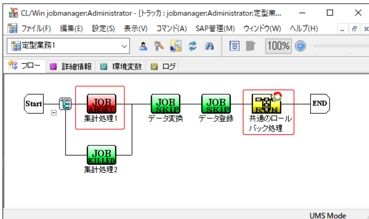
図16.23 並列分岐部品上で中断が発生した場合のジョブネットワーク
