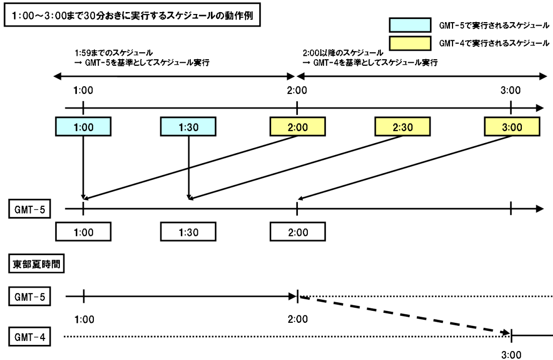
図17.7 夏時間開始時刻周辺での動作例
