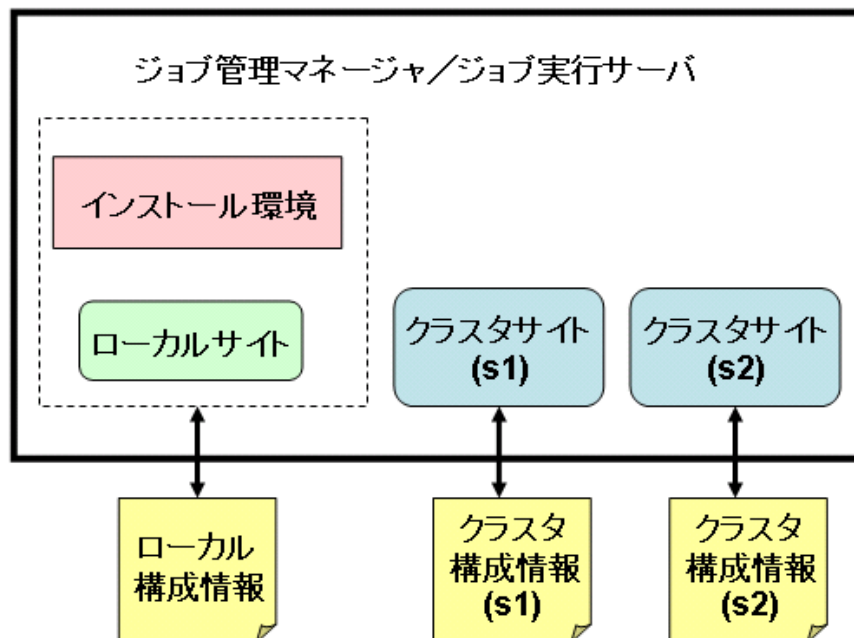
図18.1 構成情報のバックアップ・復元機能の動作イメージ
