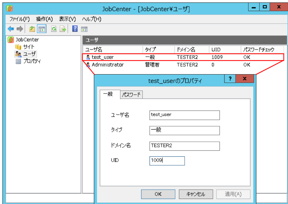
図14.16 ユーザのプロパティ画面例
