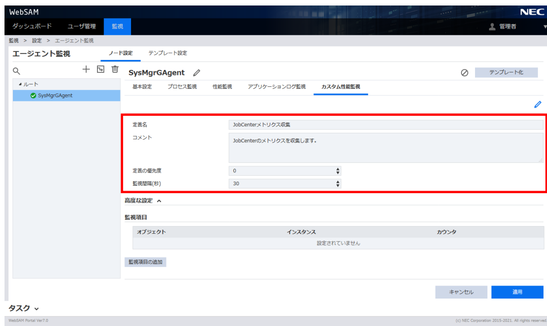
図23.5 カスタム性能監視の編集画面
