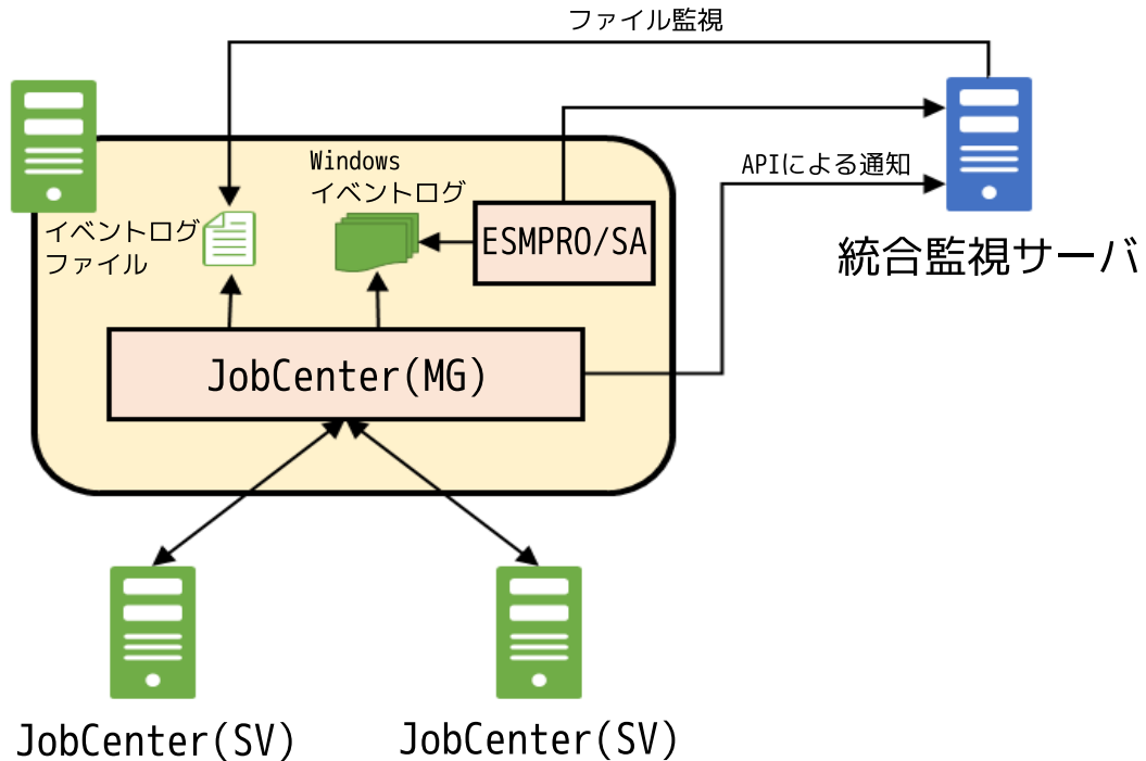
図13.2 Windows版のイベント連携のイメージ
