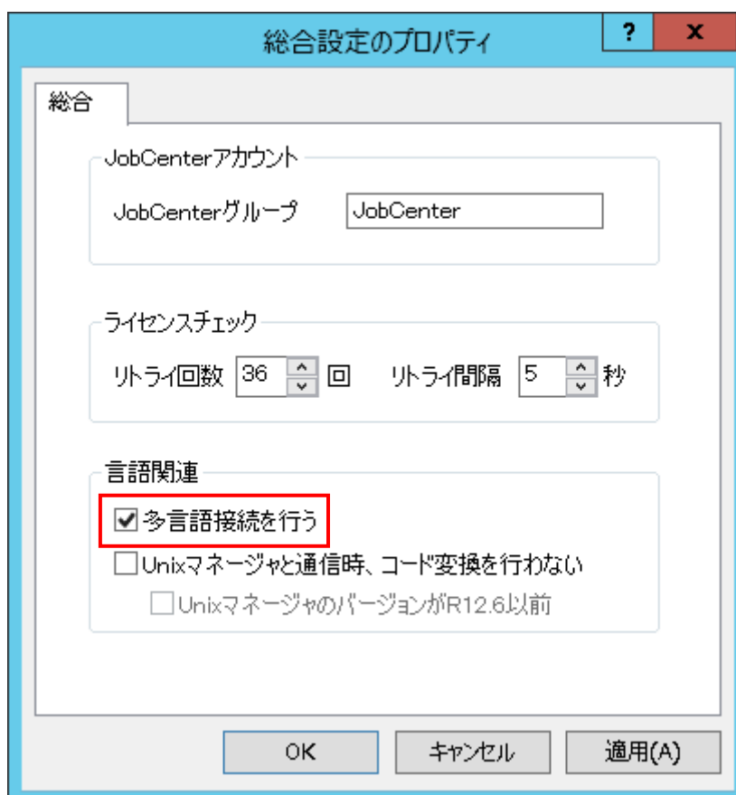
図9.1 総合設定のプロパティ画面例
