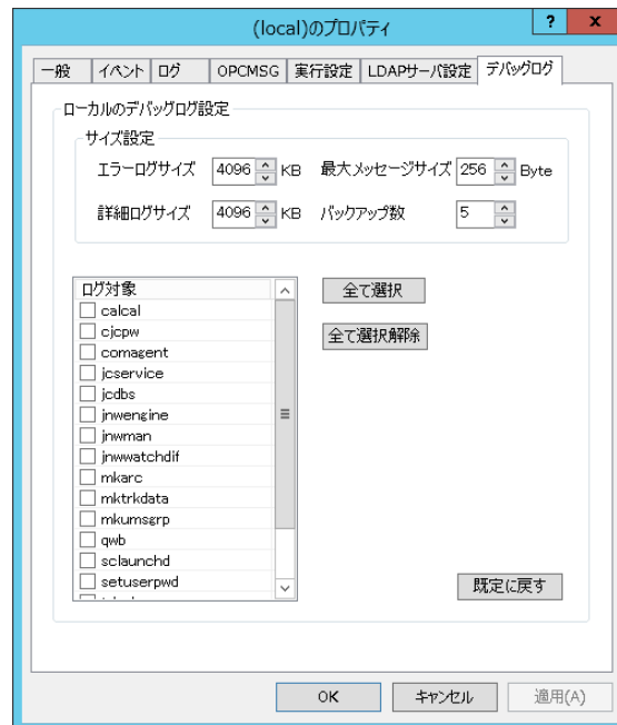
図14.11 デバッグログタブの画面例
