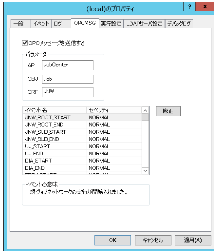
図13.20 [詳細設定] ダイアログ [OPCMSG] 画面例
