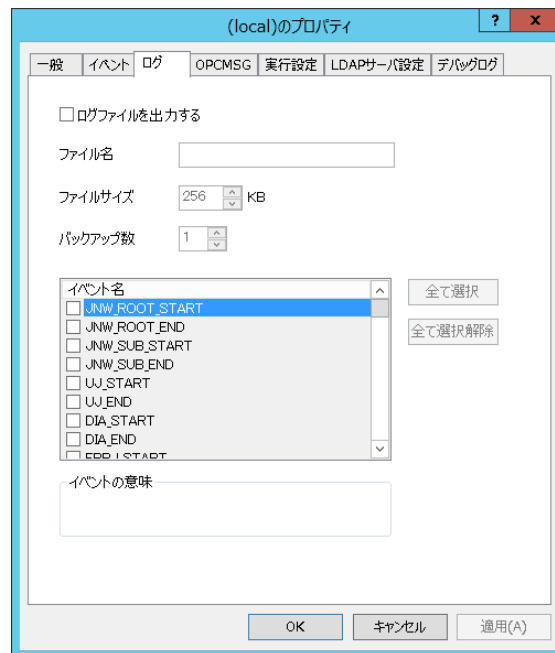
図14.7 ログタブの画面例
