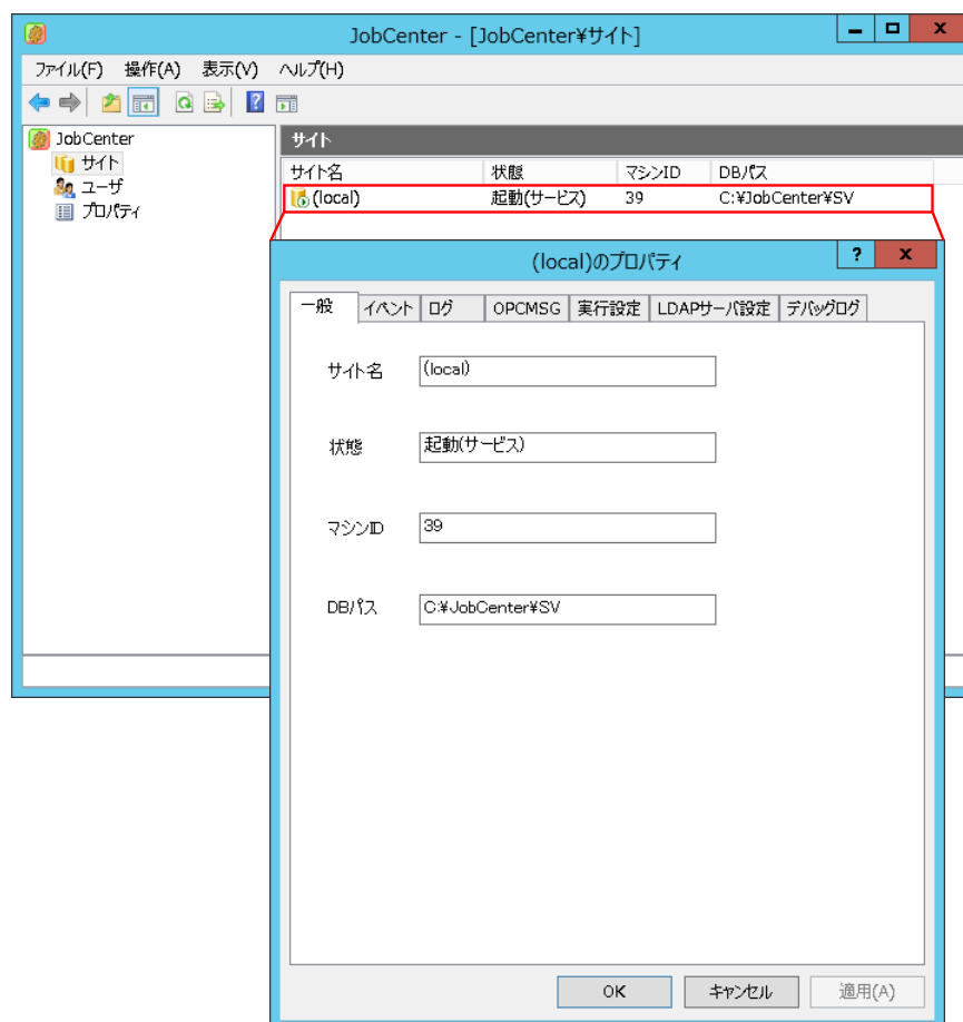
図14.4 サイトのプロパティ画面例
