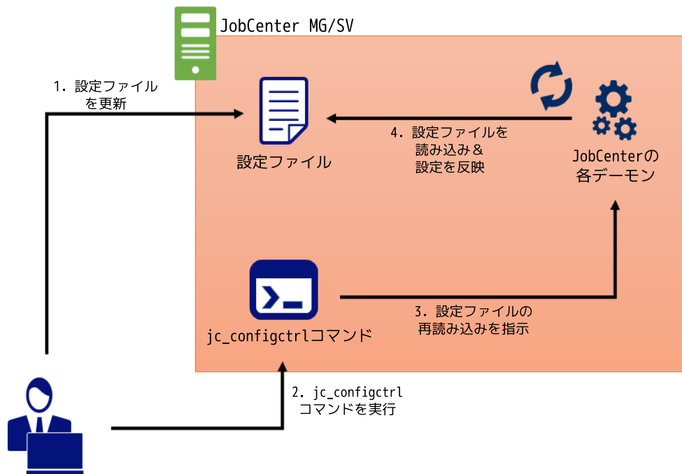
図6.1 設定ファイルの再読み込みの動作イメージ
