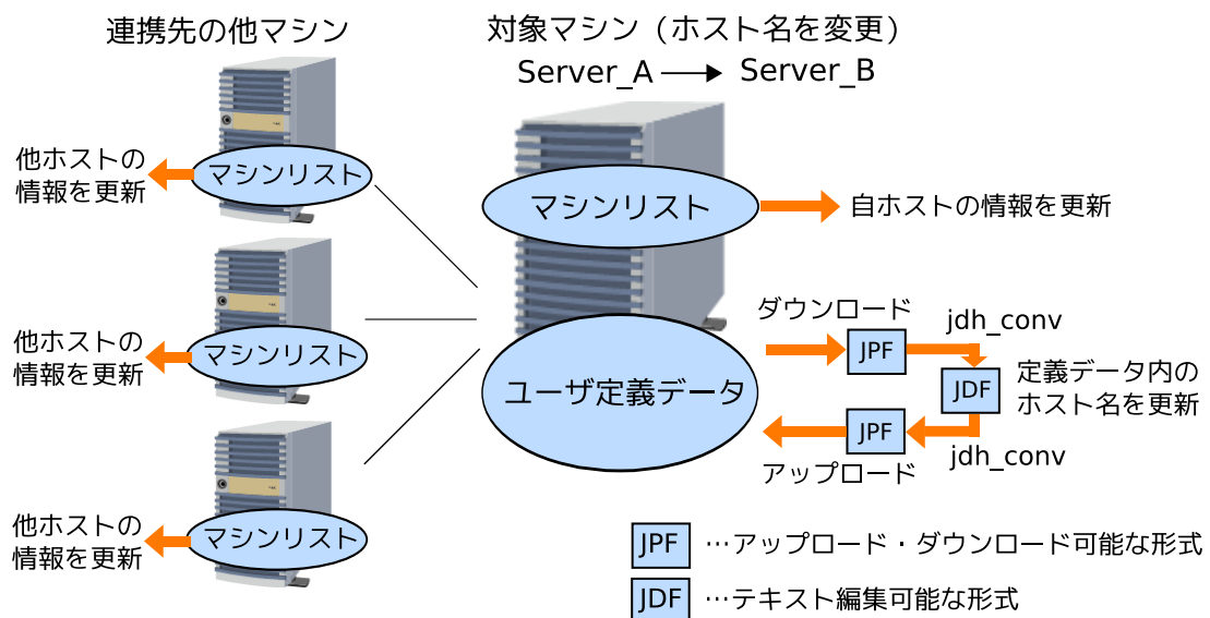
図15.4 ホスト名の変更
