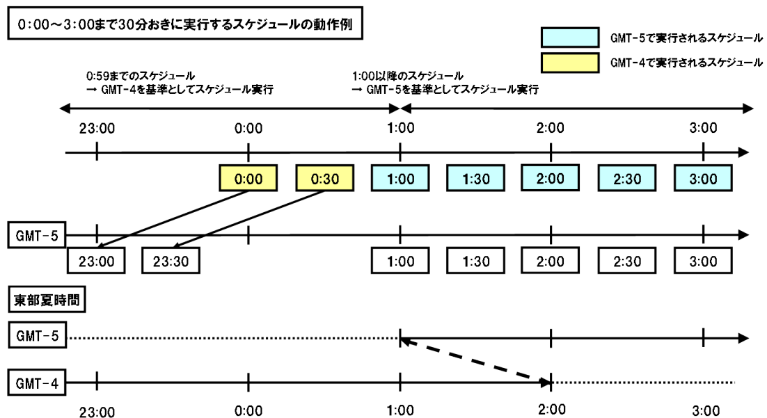
図17.8 夏時間終了時刻での動作例
