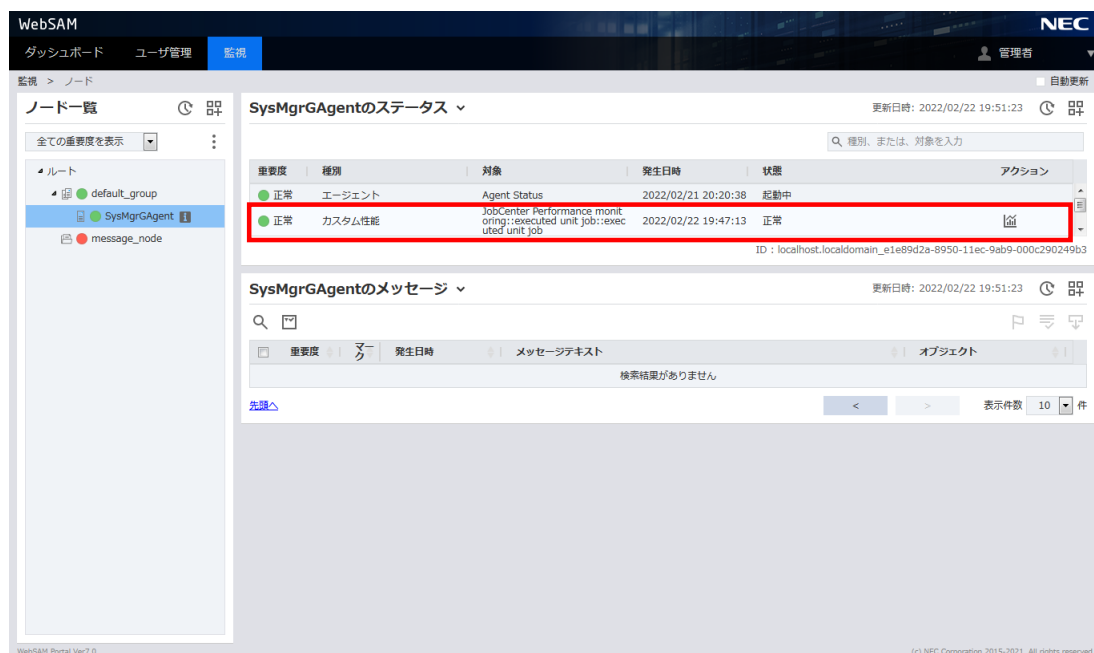
図23.12 SystemManagerGのカスタム性能監視(正常時)
