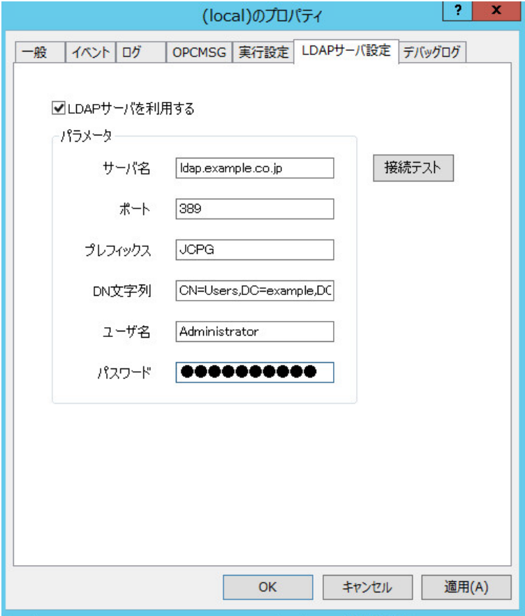
図12.3 JobCenter側のLDAPサーバ設定例
