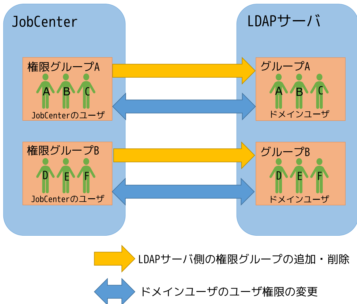
図12.1 LDAPサーバ連携機能の概要
