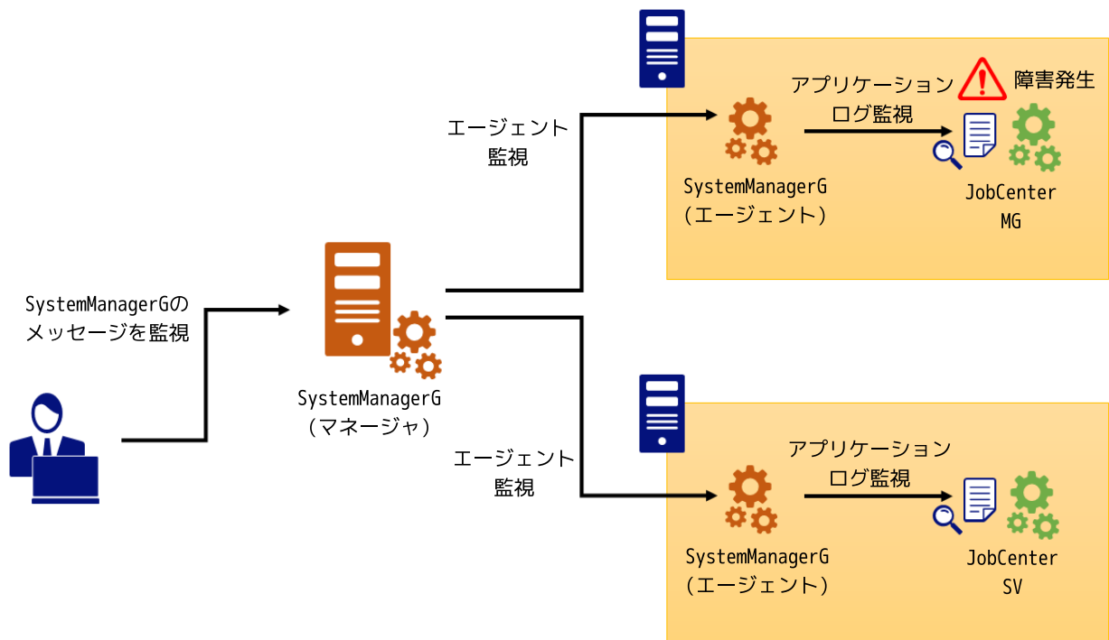
図22.1 JobCenterの障害情報監視イメージ
