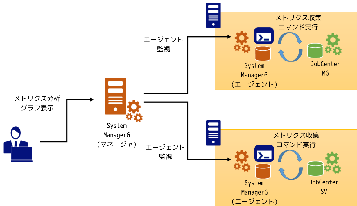
図23.1 JobCenterのメトリクス収集イメージ
