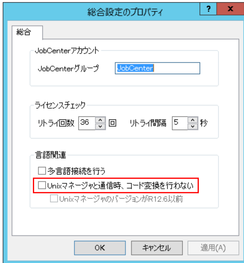
図10.1 総合設定のプロパティダイアログ画面例
