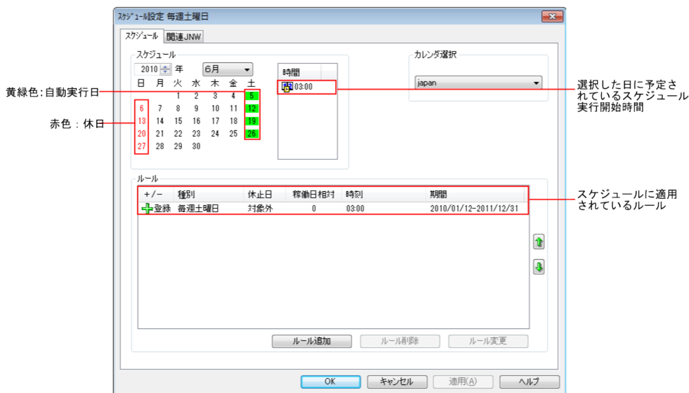
図8.1 「スケジュール設定」画面例
