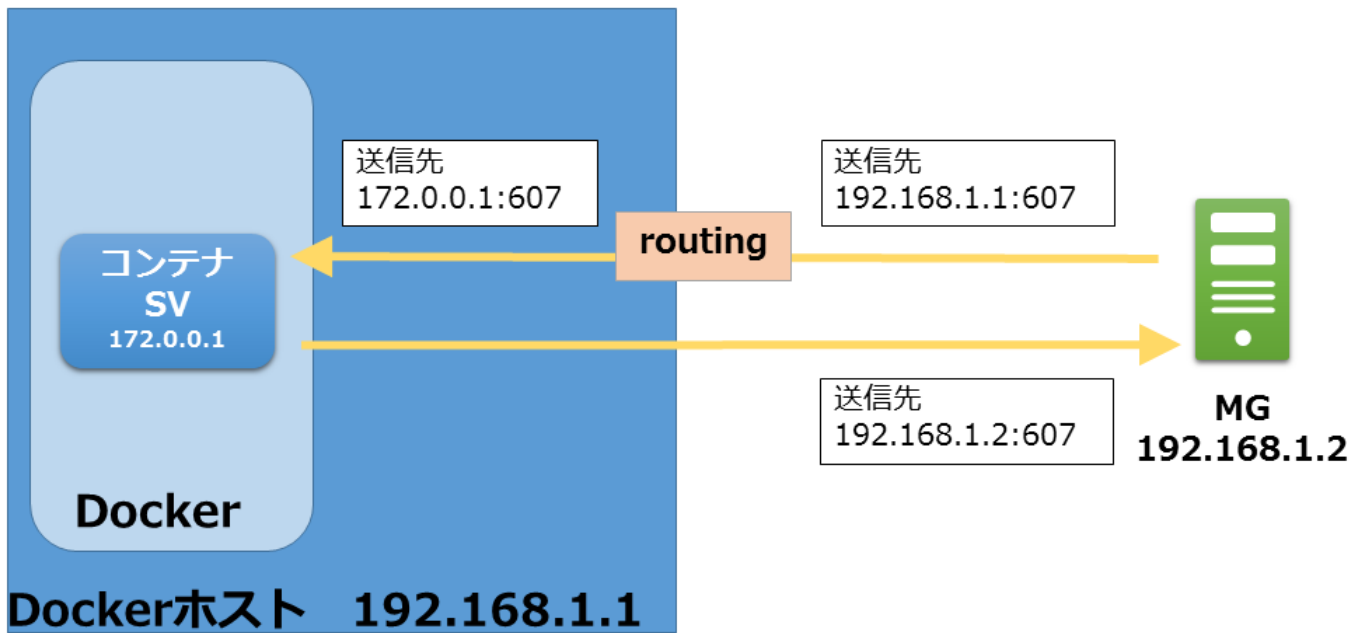
図2.8 Docker外部との通信
