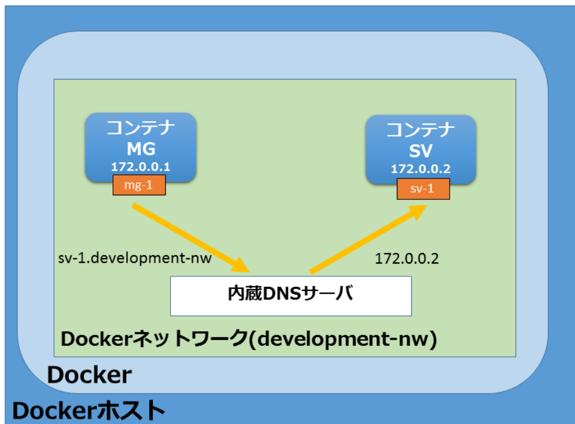
図2.7 Docker内部での通信
