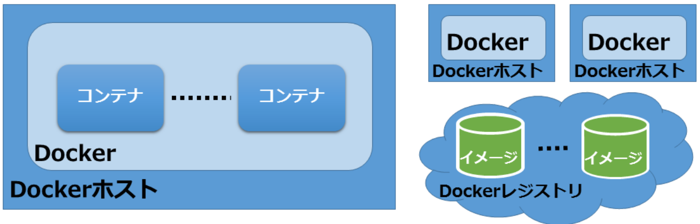
図2.1 Docker環境
