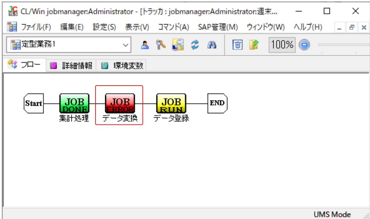
図16.65 エラーが発生したサブジョブネットワーク
