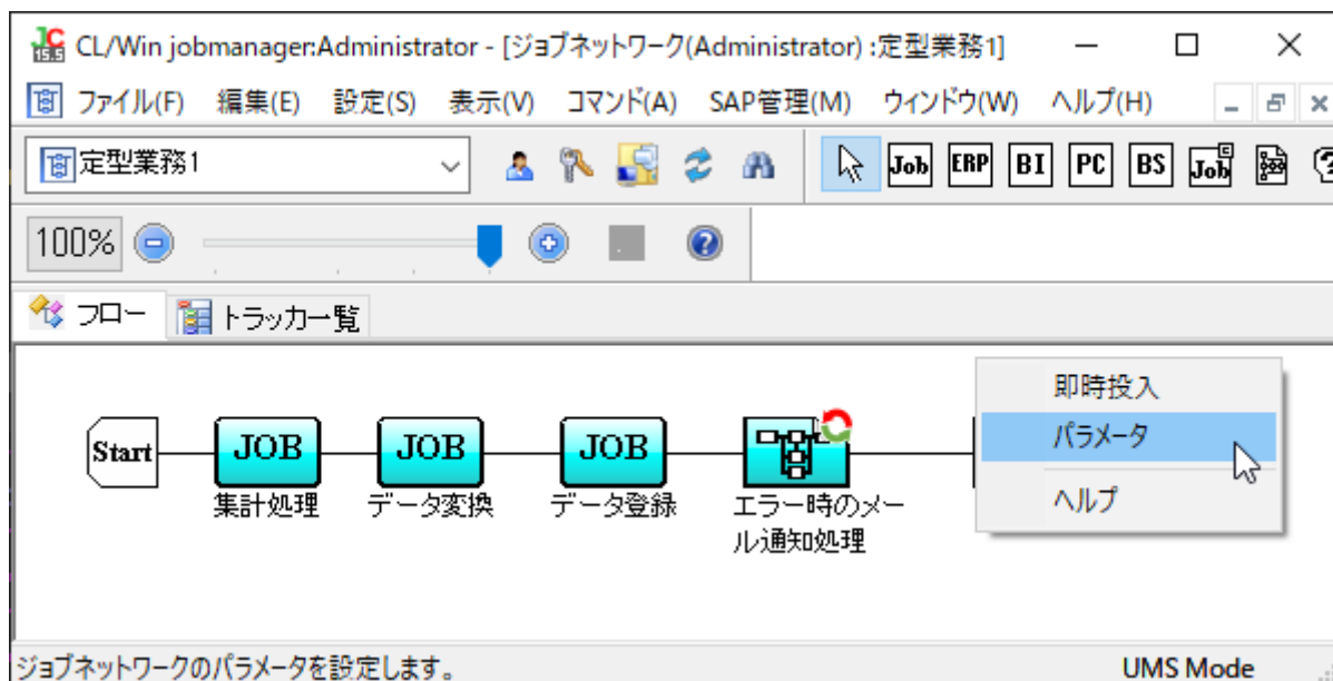
図16.7 ジョブネットワークのパラメータの表示
