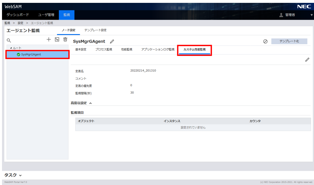
図21.3 カスタム性能監視の設定画面の表示方法
