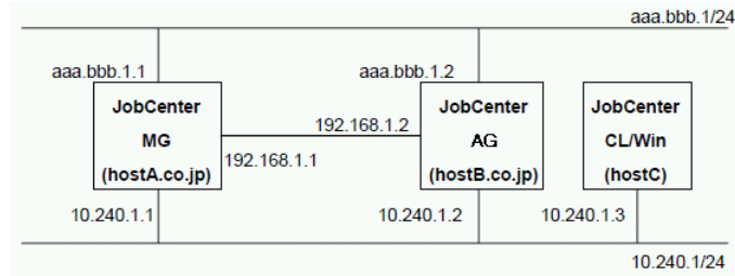
図3.1 IPアドレスの指定例
