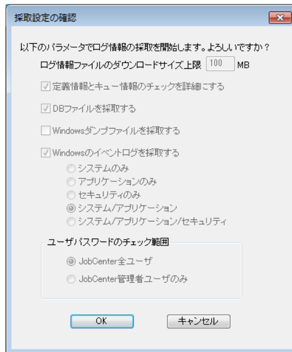
図24.8 [採取設定の確認]画面
