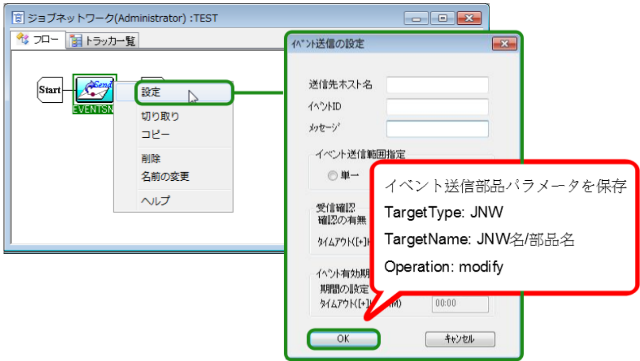
図7.39 イベント送信部品に対する操作
