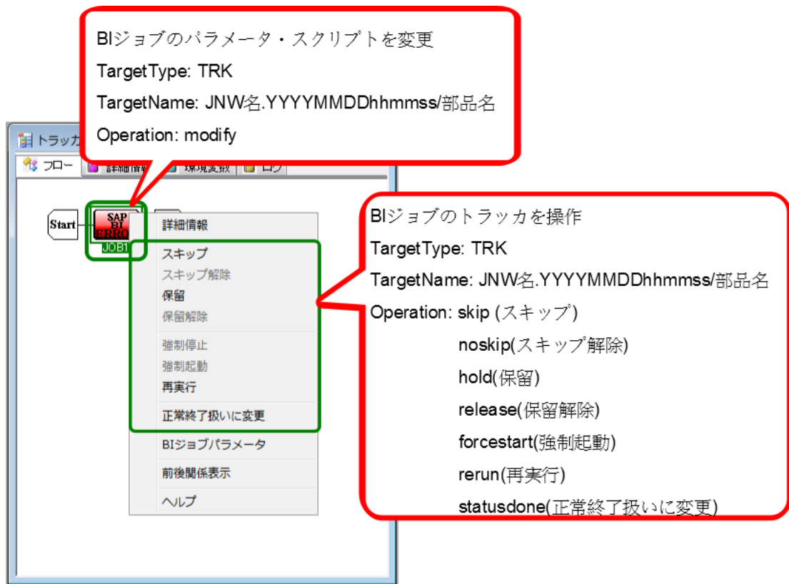
図7.12 BIジョブトラッカに対する操作
