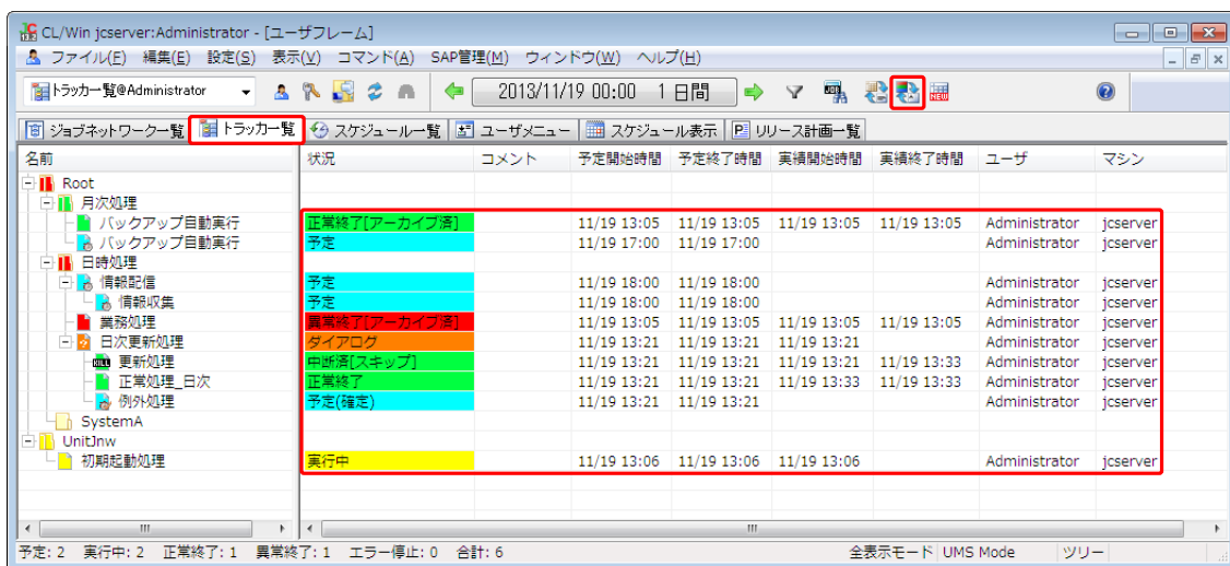
図5.5 ユーザフレームのトラッカー一覧（テキストモード）画面例
