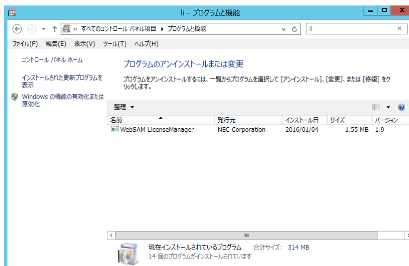
図2.6 画面例
