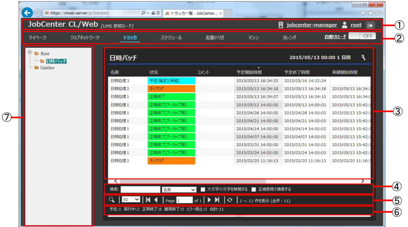
図5.1 CL/Web画面
