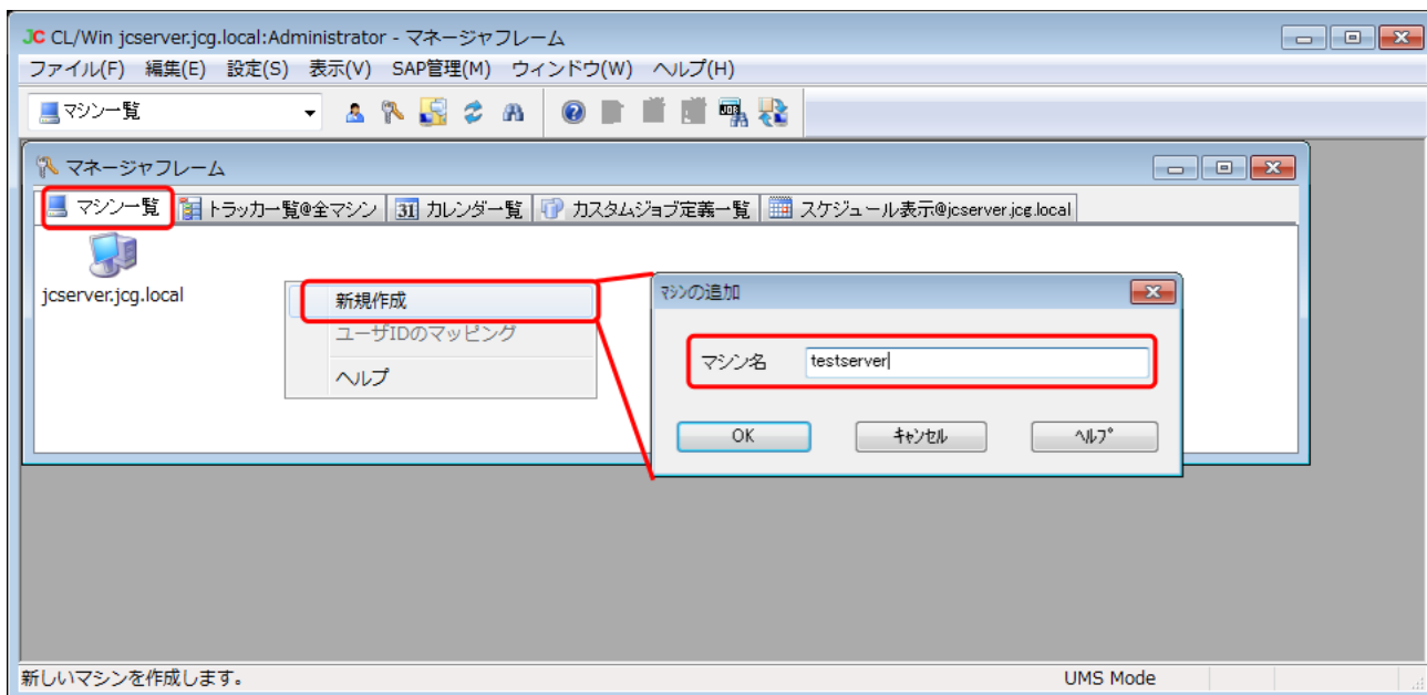
図6.2 マシーナ一覧へのマシン追加画面例（簡易リモートマシン構成機能）
