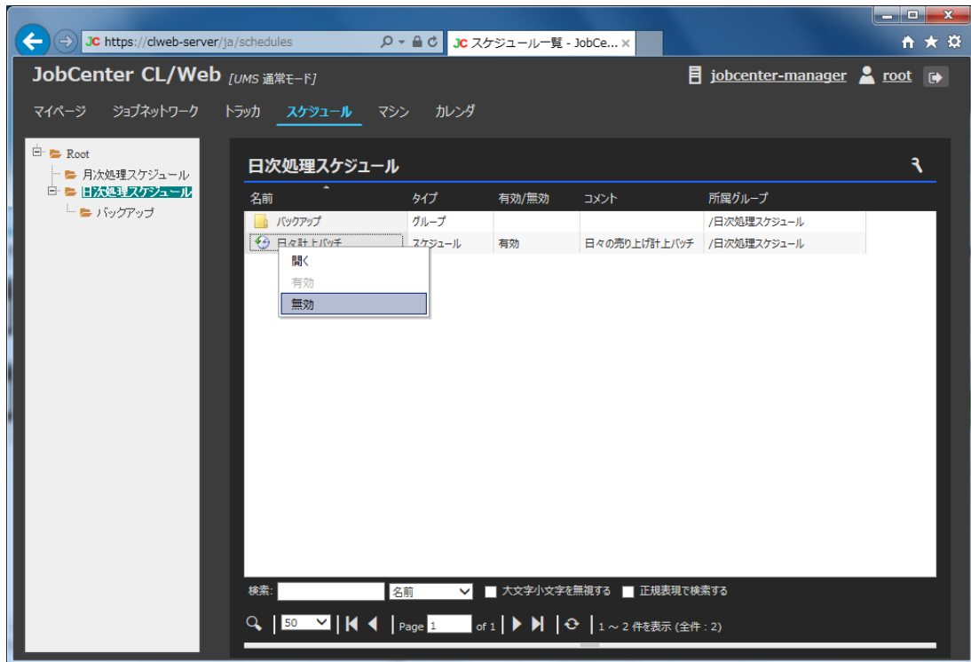
図5.46 スケジュールの無効化選択
