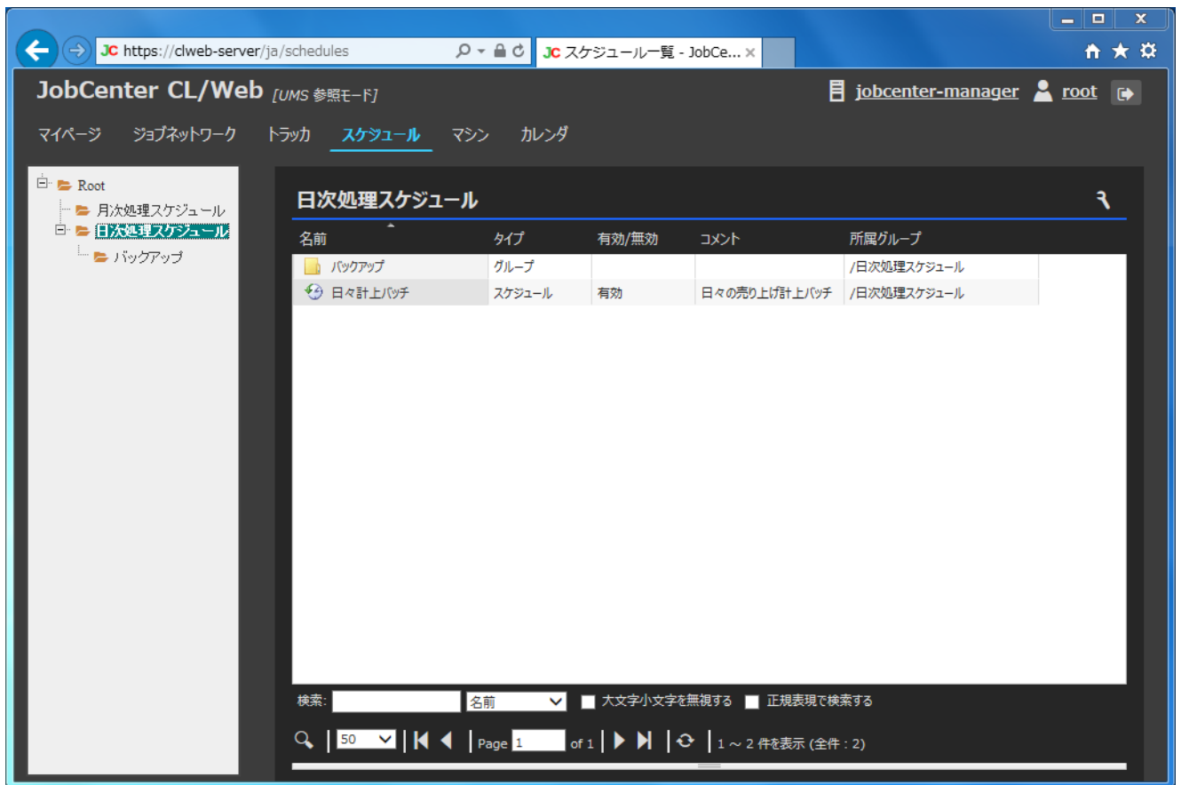
図5.42 スケジュールグループ選択画面
