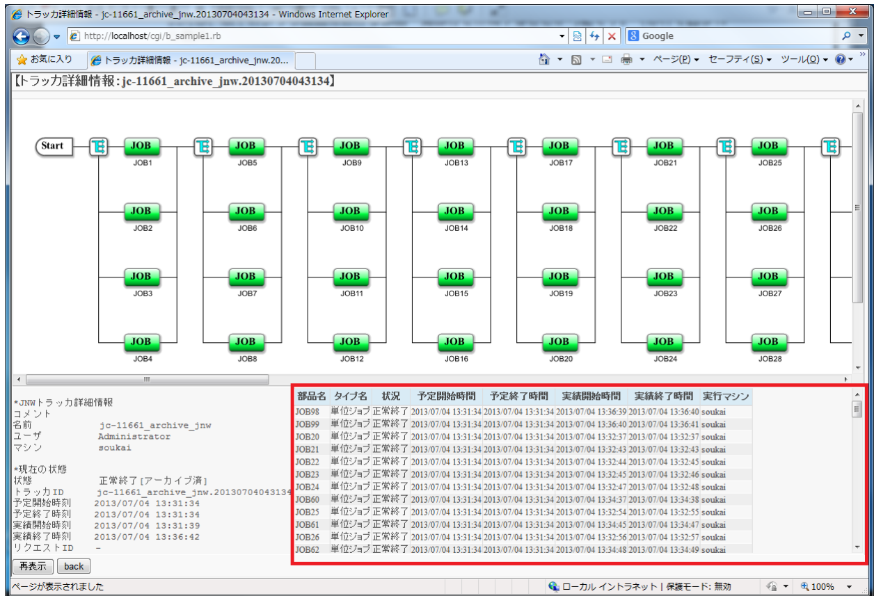
図6.10 トラッカ詳細表示例
