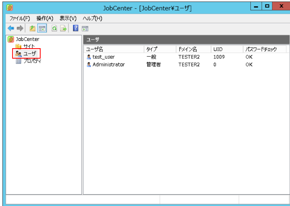
図13.15 ユーザ画面例
