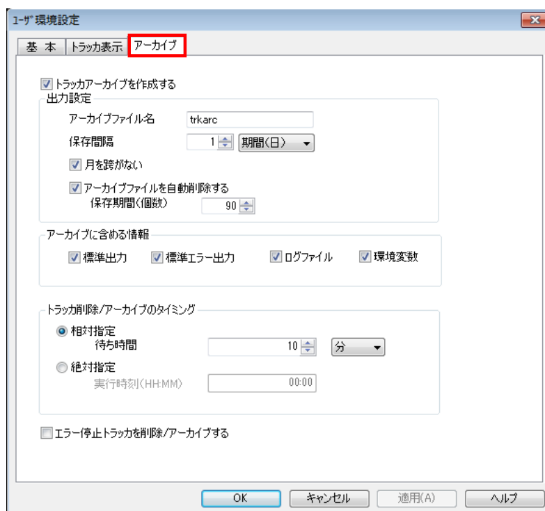
図8.57 [ユーザ環境設定] ダイアログの [アーカイブ] タブの画面例
