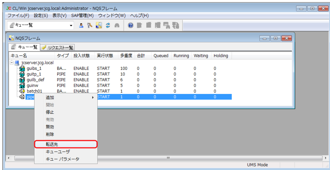
図10.19 転送先キューの指定画面例
