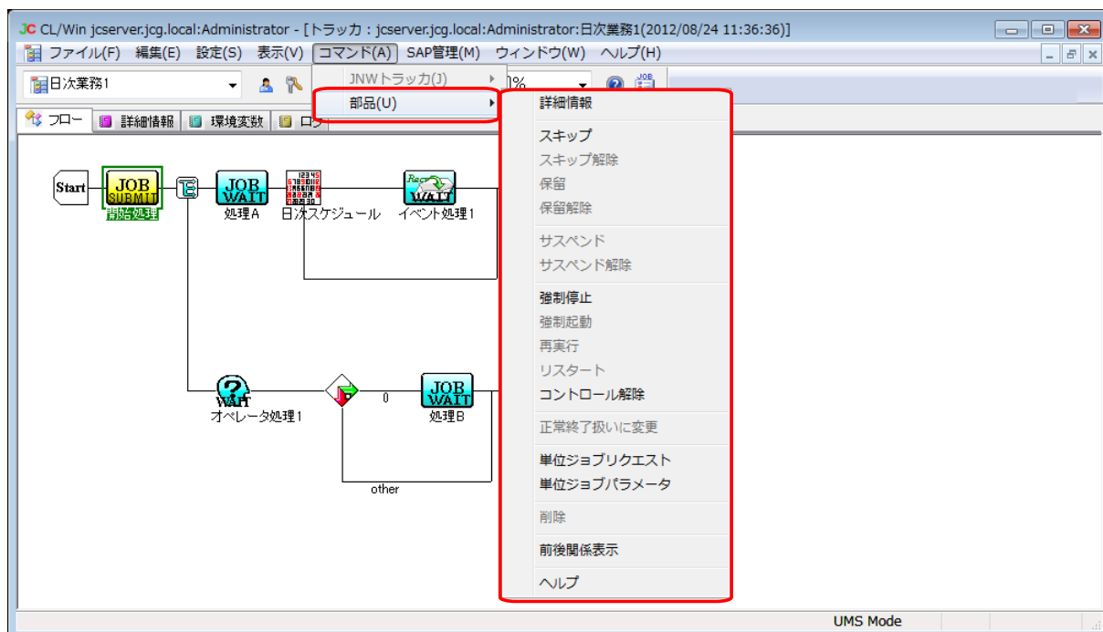
図8.49 [ジョブネットワークトラッカ] ウィンドウのフロー上で部品を選択している場合のメニュー [コマンド] - [部品] の画面例
