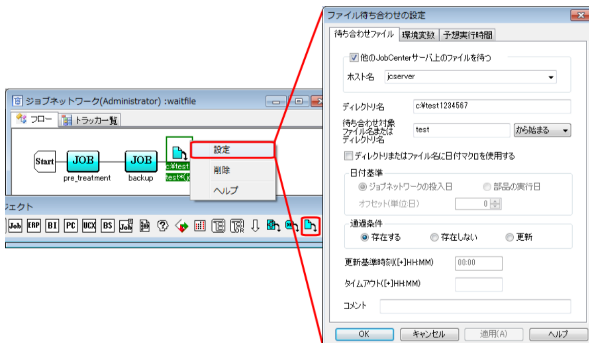
図4.21 ファイル待ち合わせ設定画面例
