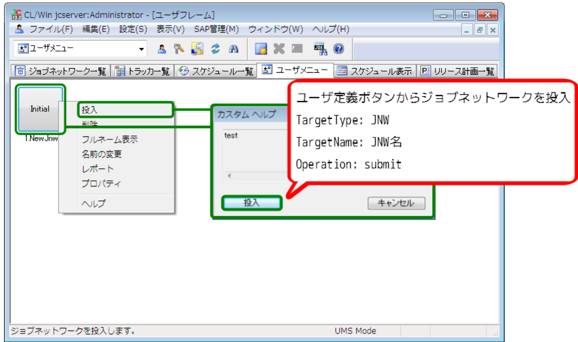
図7.25 ユーザメニューの操作
