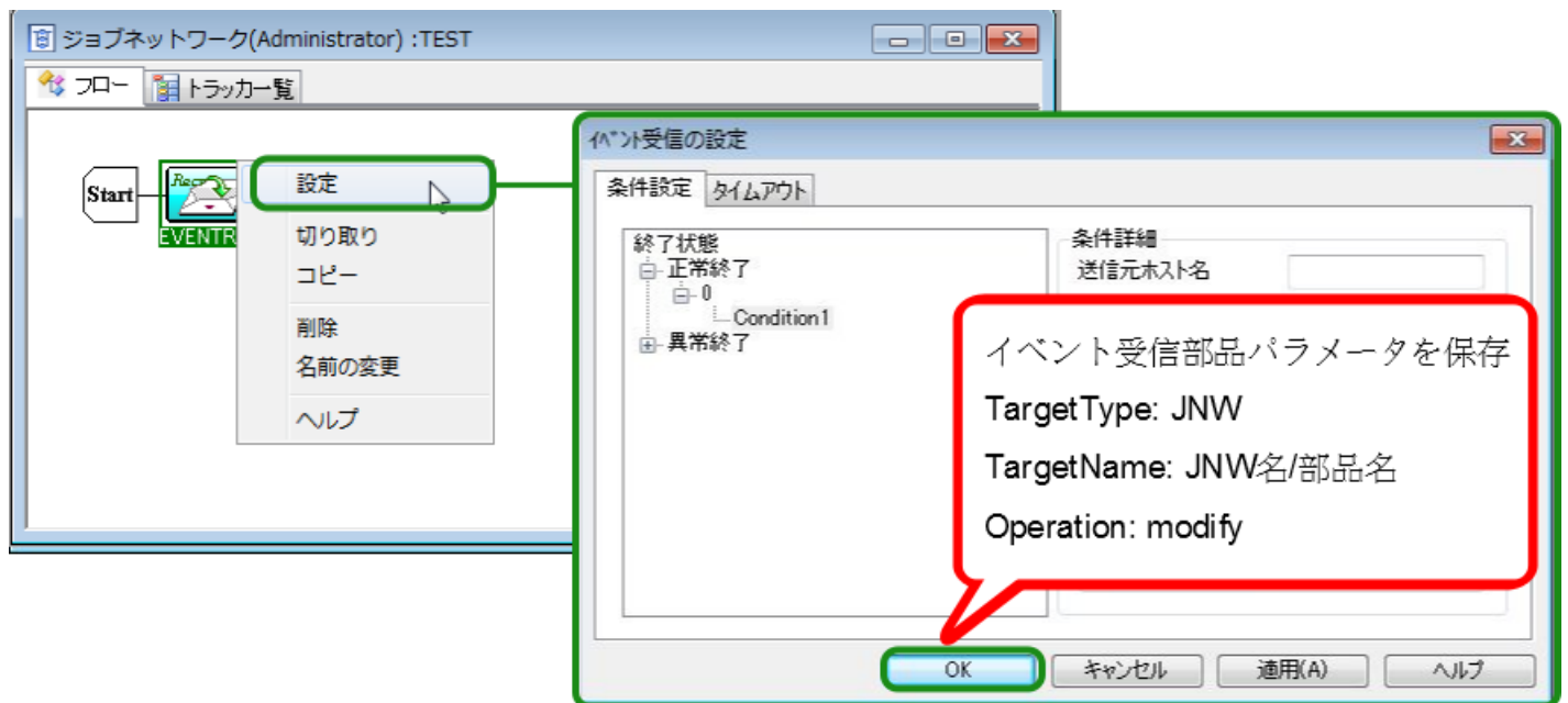
図7.36 イベント受信部品に対する操作
