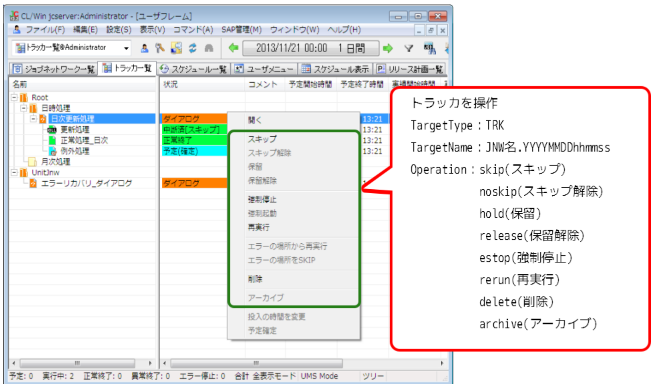
図7.6 トラッカに対する操作（共通）
