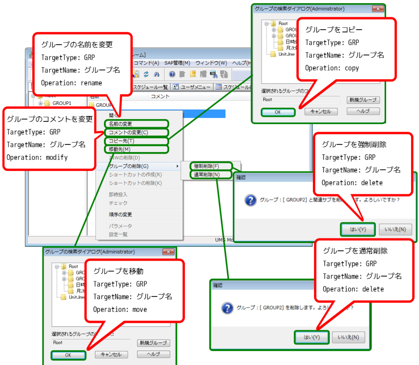
図7.1 グループに対する操作
