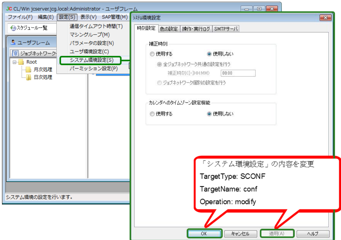
図7.26 システム環境設定に対する操作
