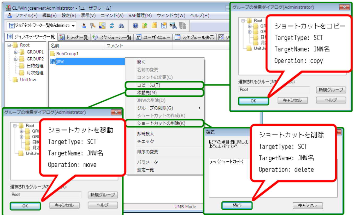
図7.5 ショートカットに対する操作
