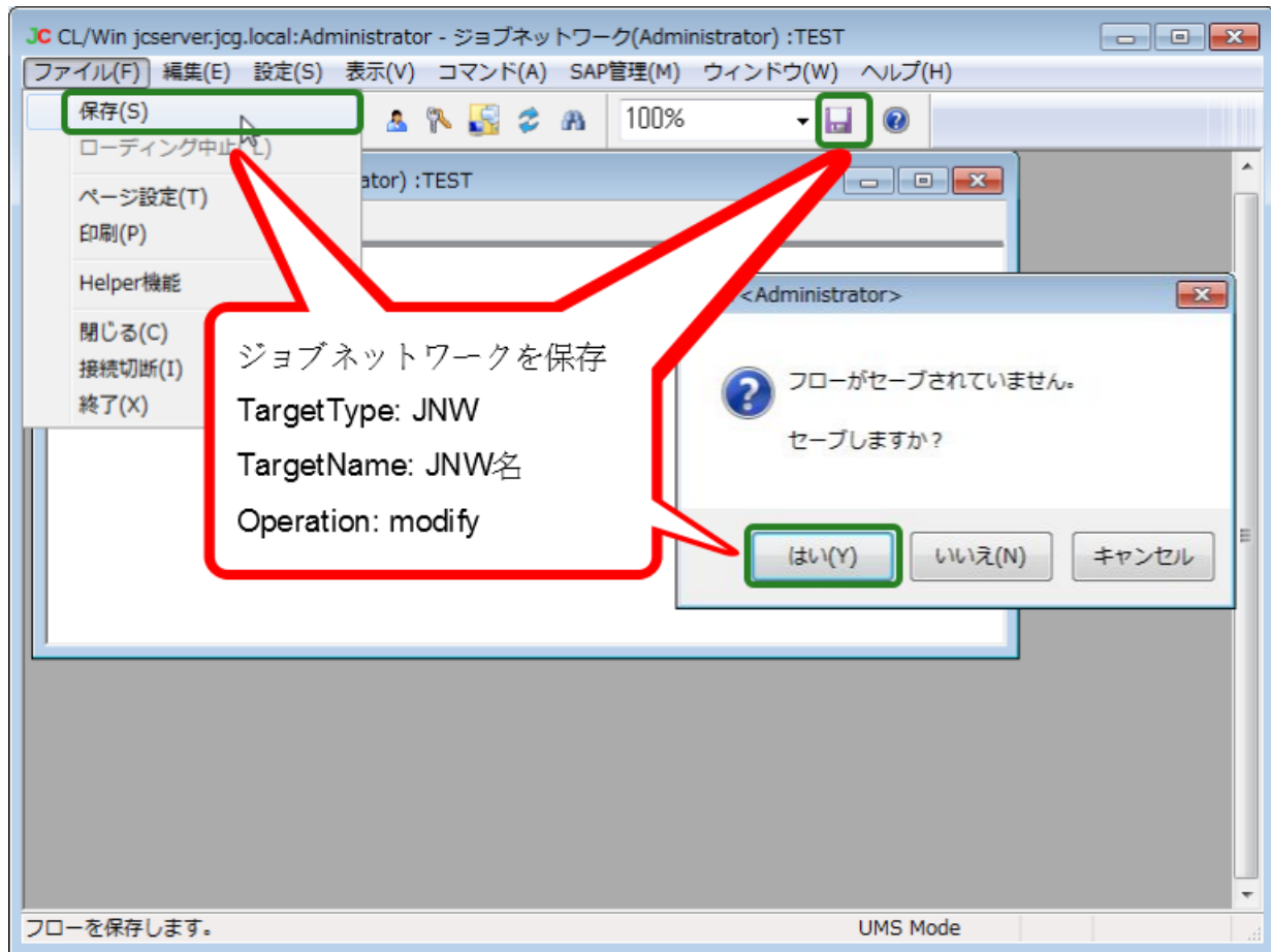
図7.28 ジョブネットワークフローに対する操作
