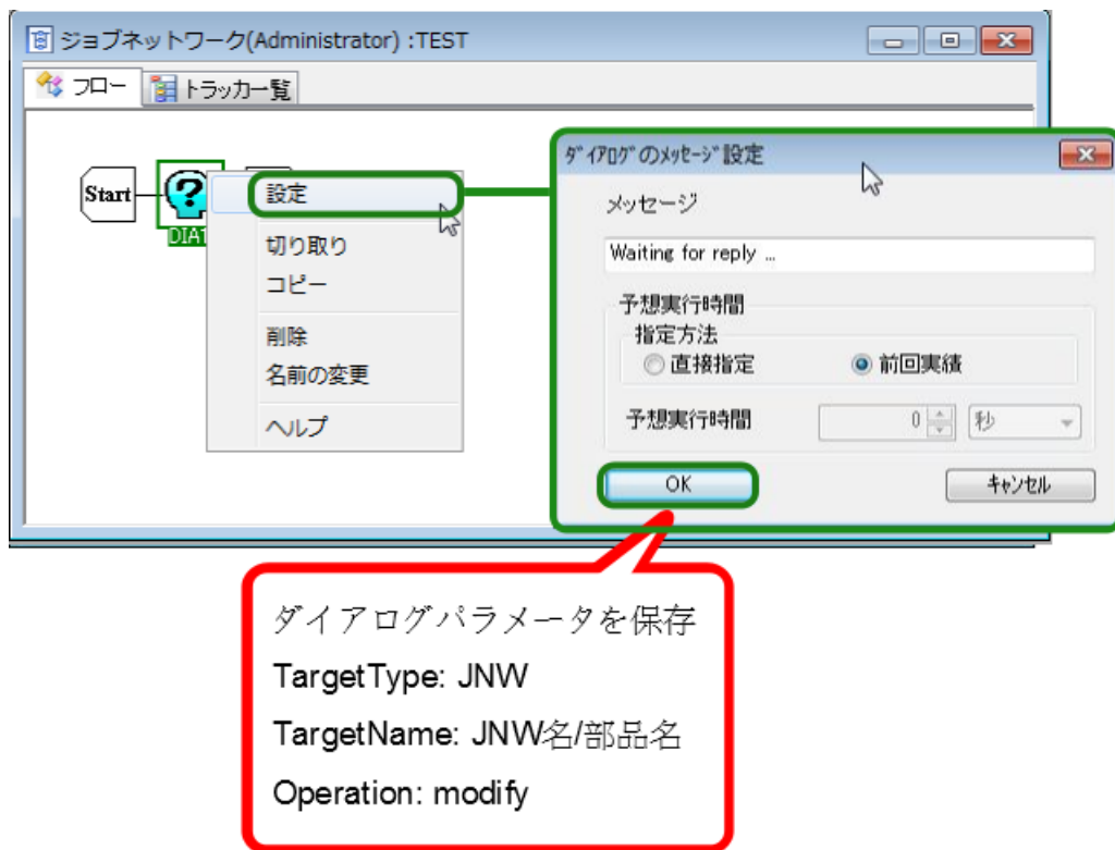
図7.33 ダイアログ部品に対する操作
