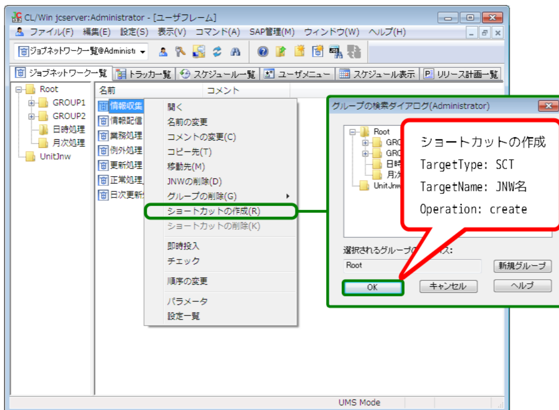
図7.4 ショートカットに対する操作
