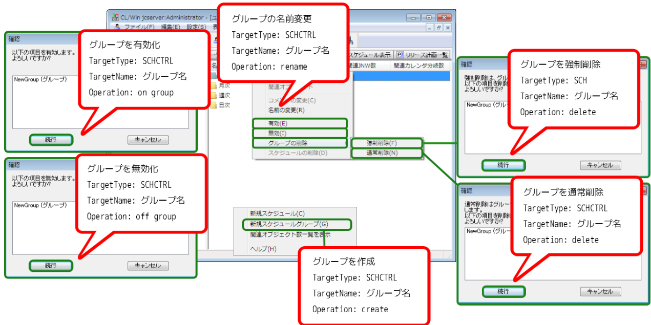
図7.23 スケジュールグループに対する操作
