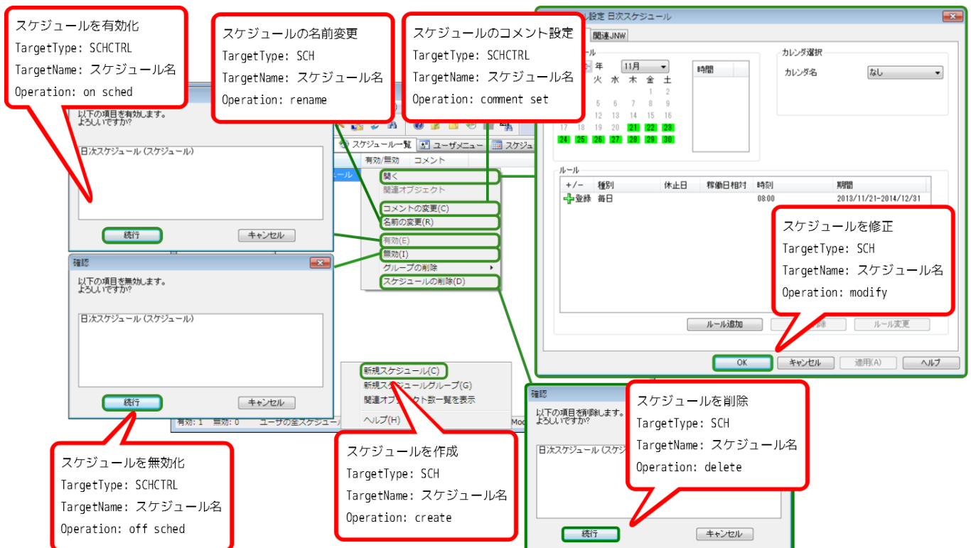
図7.24 スケジュールに対する操作
