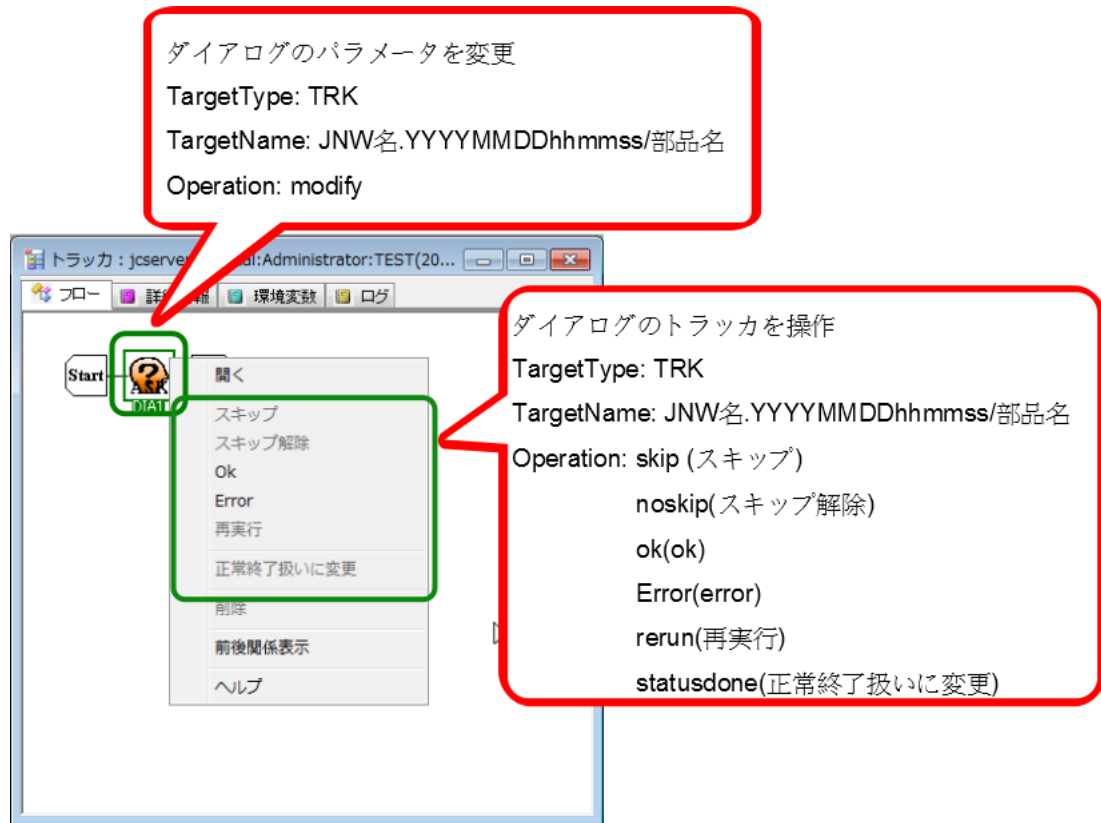
図7.14 ダイアログ部品トラッカに対する操作
