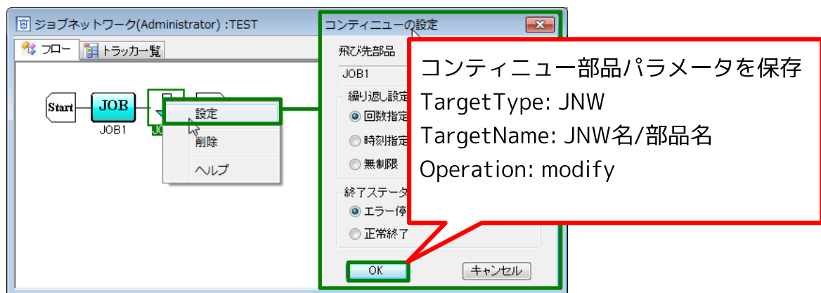
図7.34 コンティニュー部品に対する操作
