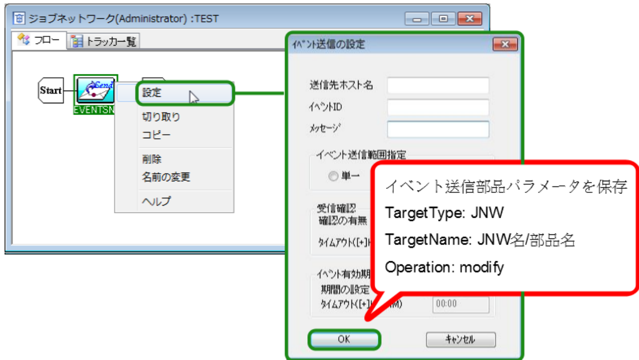
図7.35 イベント送信部品に対する操作
