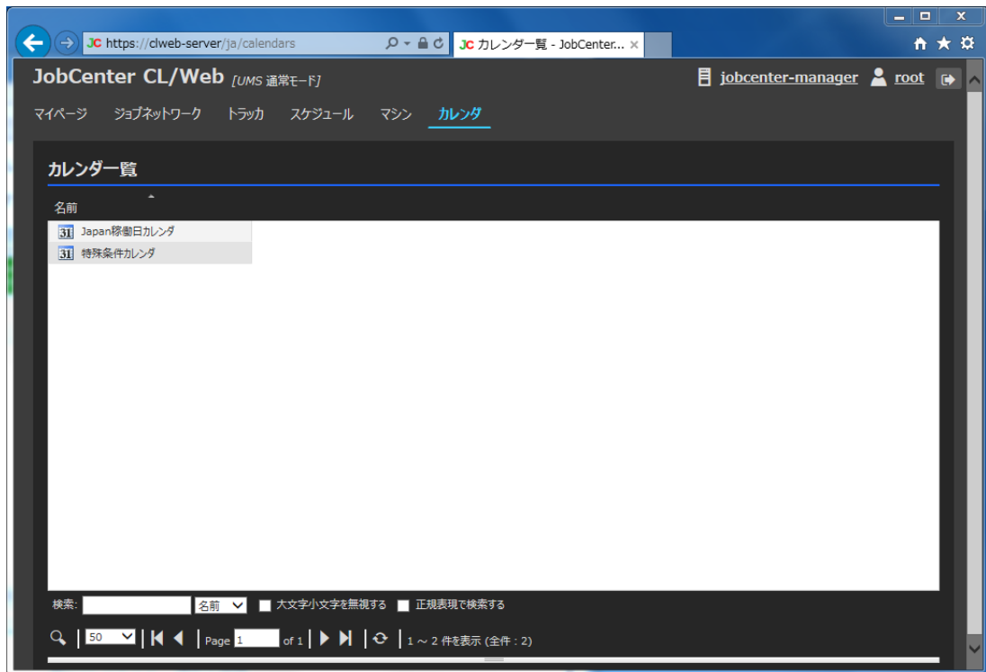
図5.59 カレンダー一覧表示画面
