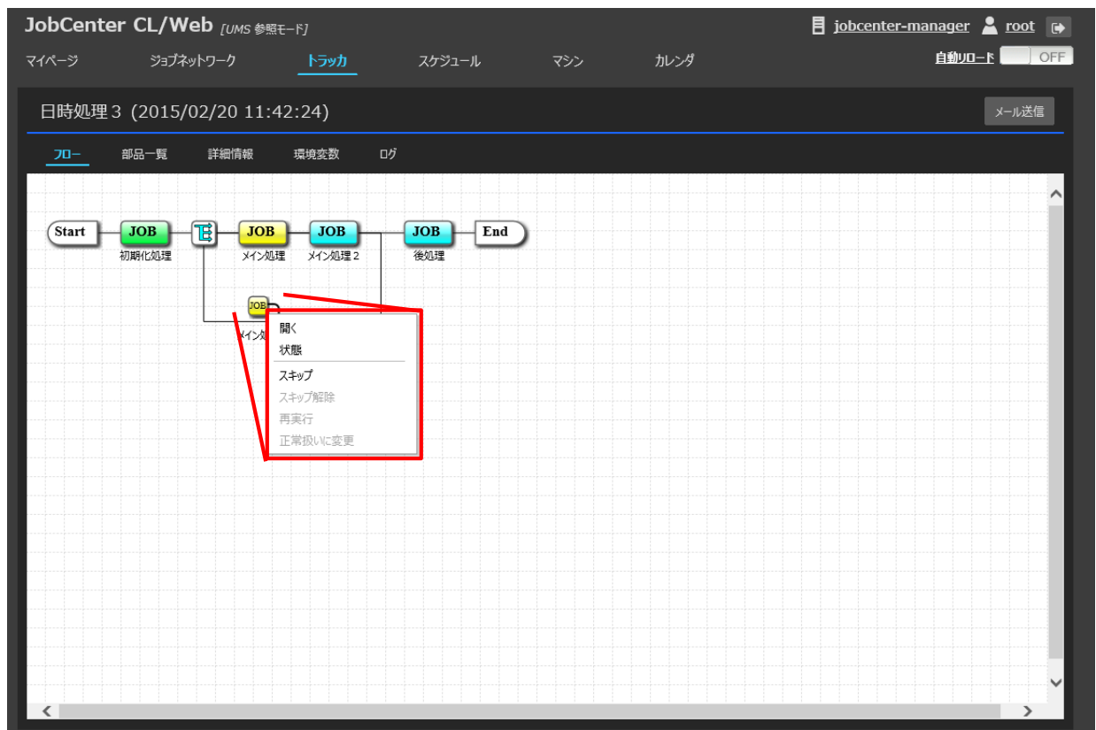
図5.35 ジョブ待ち合わせ部品の詳細画面
