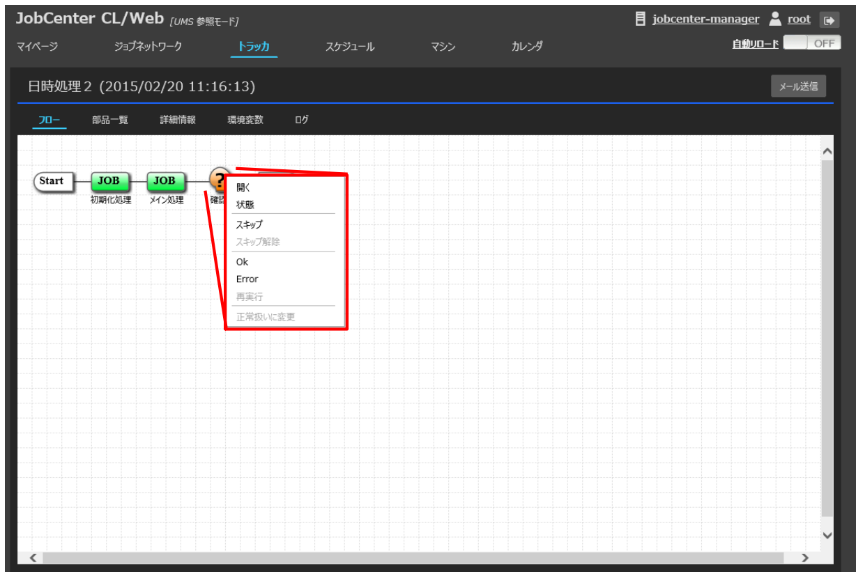
図5.34 ダイアログトラック部品の詳細画面
