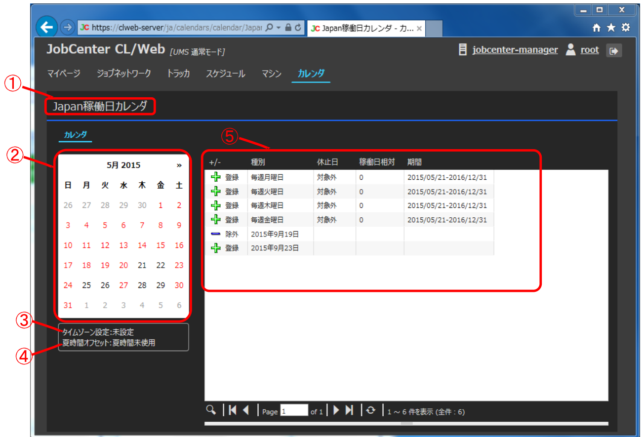
図5.61 カレンダー定義情報表示画面
