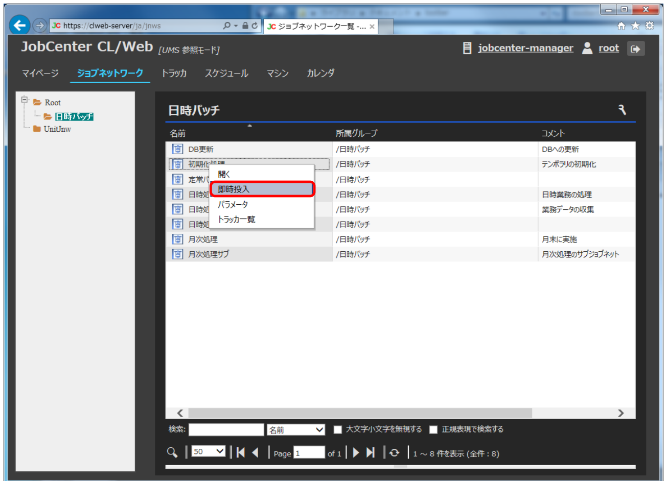
図5.17 ジョブネットワーク表示テーブルでの[即時投入]の選択画面
