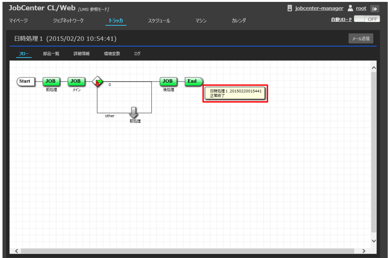
図5.26 ジョブフロー表示画面
