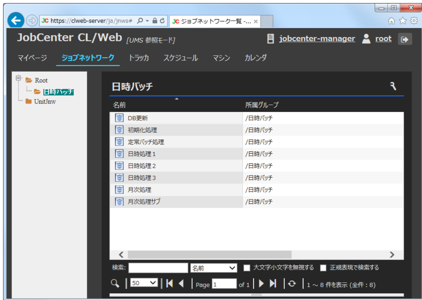
図1.1 JobCenter CL/Web画面イメージ
