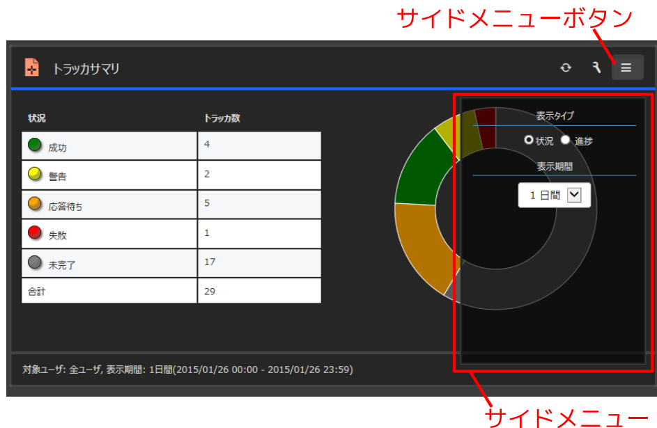
図5.77 サイドメニュー表示
