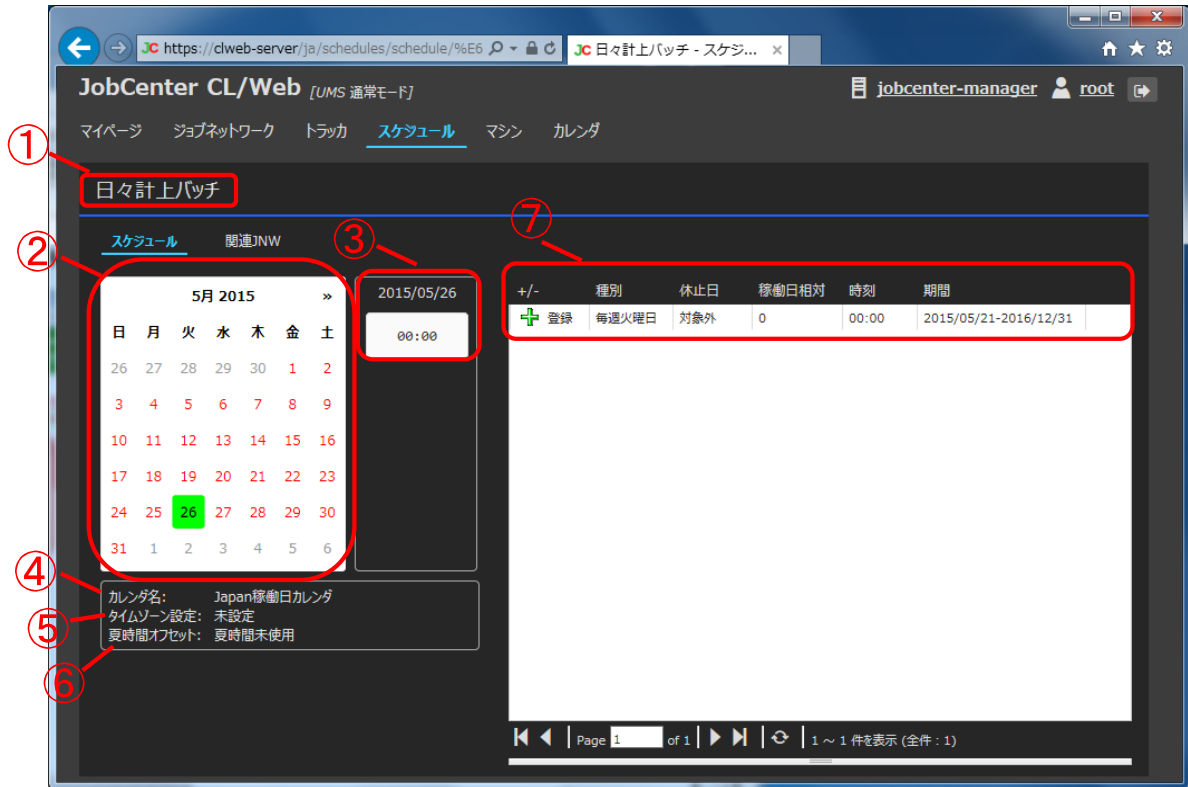
図5.42 スケジュール定義参照画面
