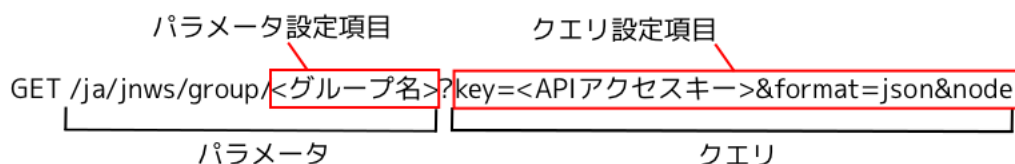
図6.15 GETメソッド設定項目
