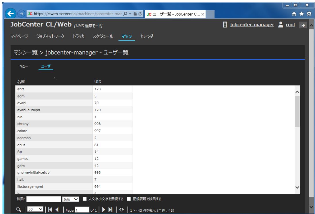
図5.58 ユーザタブ選択画面
