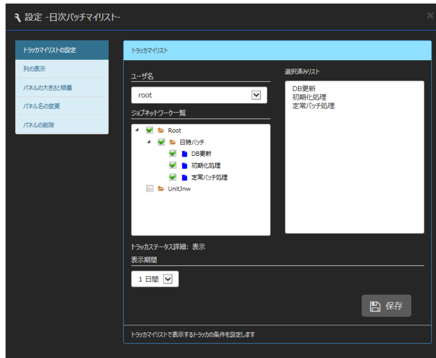
図5.82 トラッカマイリスト設定ダイアログ（ジョブネットワーク選択）
