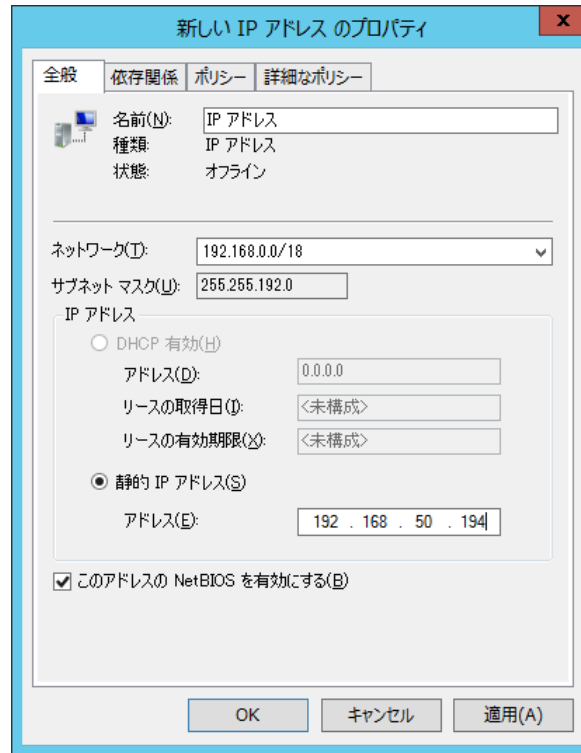
図6.12 IP アドレスの追加画面例
