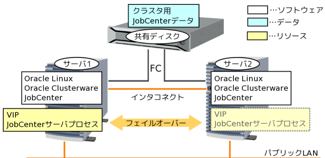
図7.1 構成例
