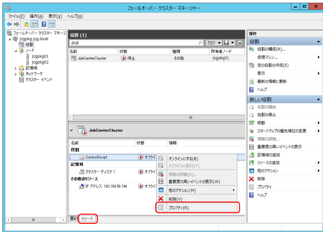
図6.15 クラスタサービスの概要画面例
