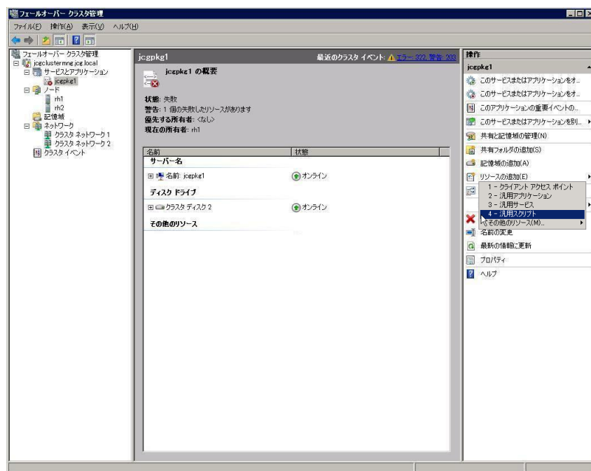
図6.6 リソースタイプの追加画面例
