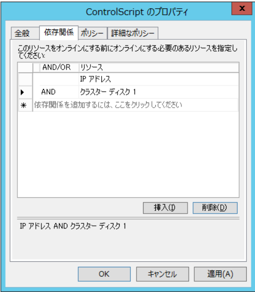
図6.16 依存関係設定画面例
