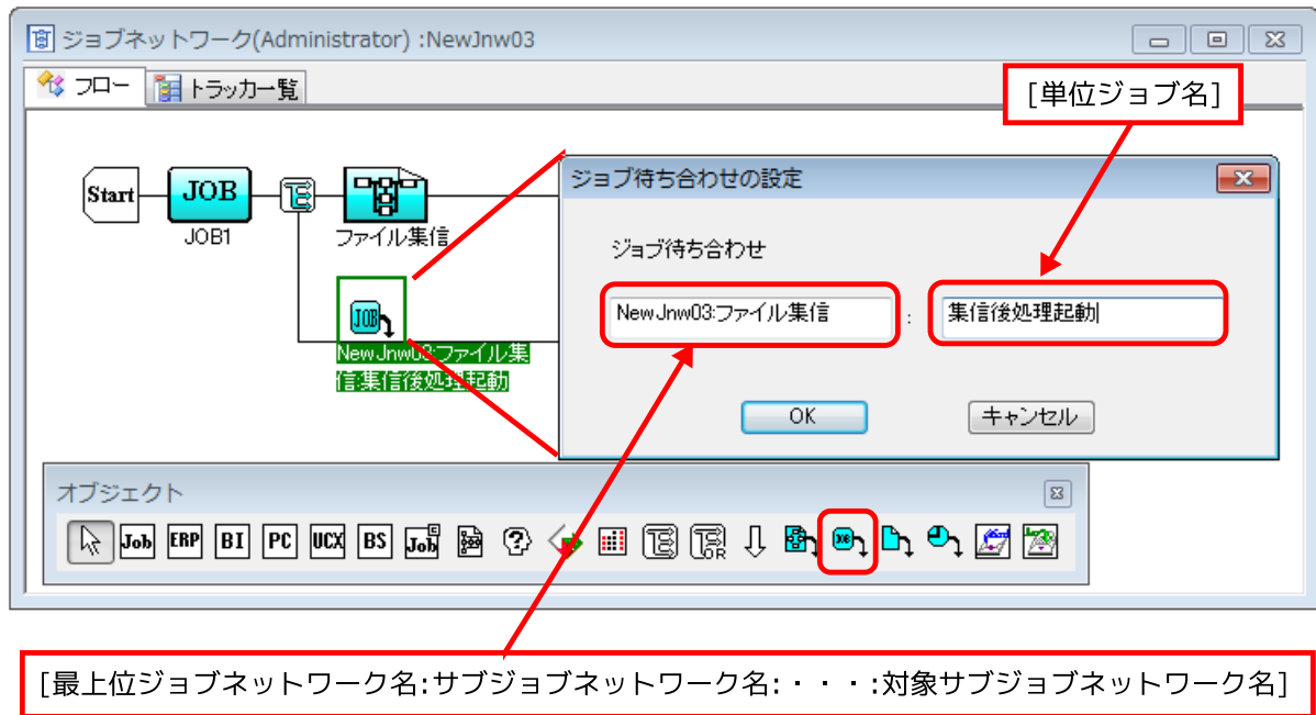
図4.20 ジョブ待ち合わせの設定例
