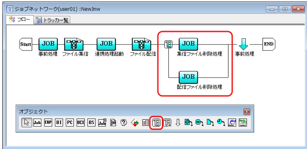
図4.11 並列分岐オブジェクト配置例
