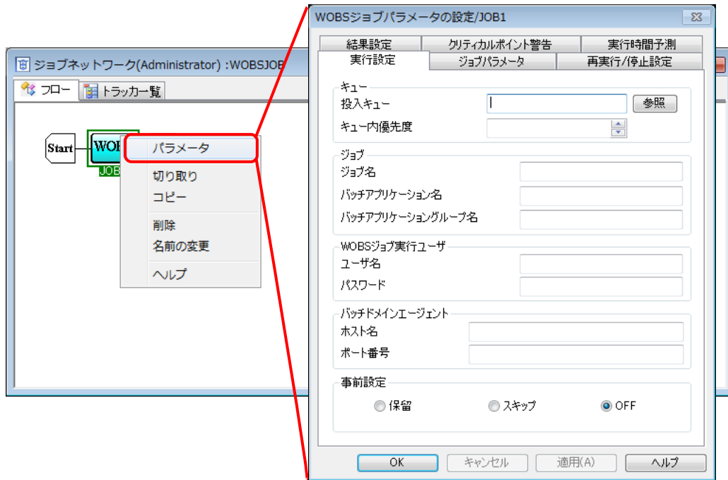
図4.8 WOBSジョブパラメータの設定画面
