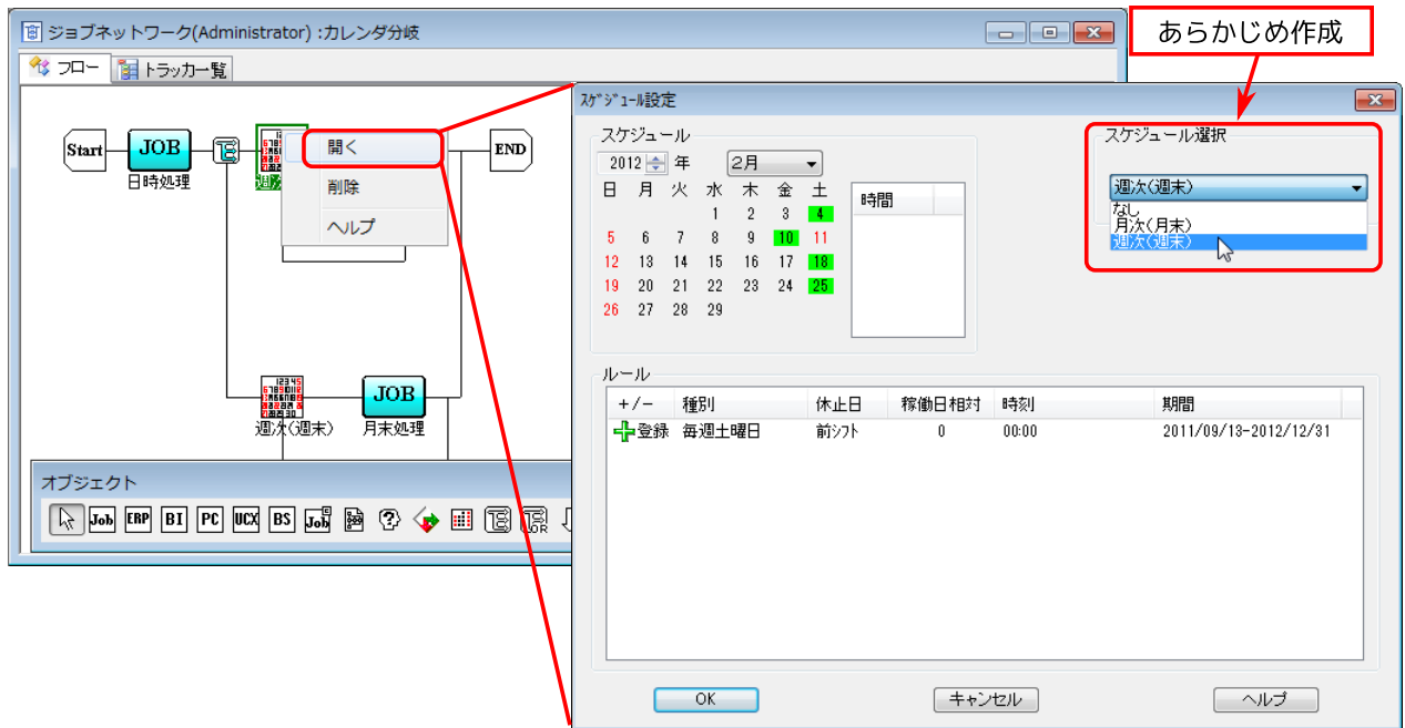
図4.17 スケジュール設定画面例
