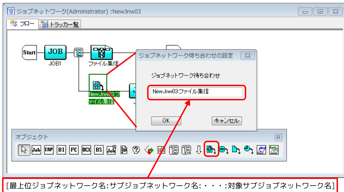
図4.21 ジョブネットワーク待ち合わせの設定例
