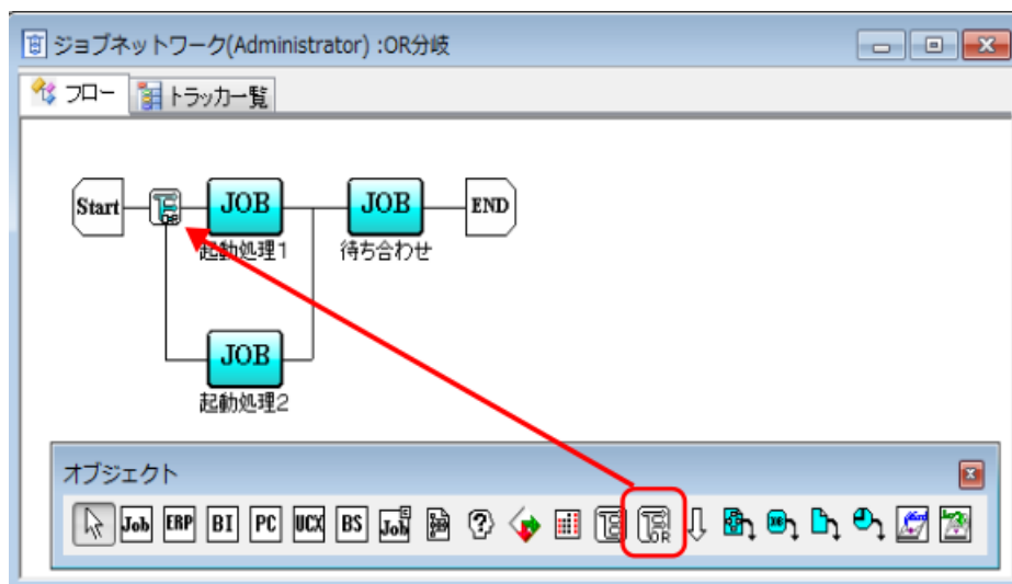
図4.13 OR分岐フローの追加と削除
