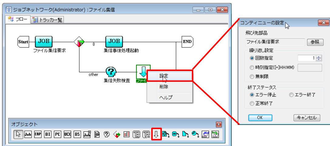
図4.18 コンティニュー部品の設定画面例
