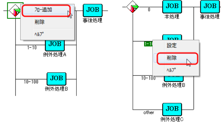
図4.15 条件分岐フローの追加と削除
