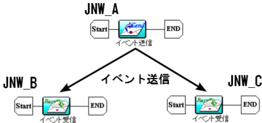
図4.25 スター型連携モデル例
