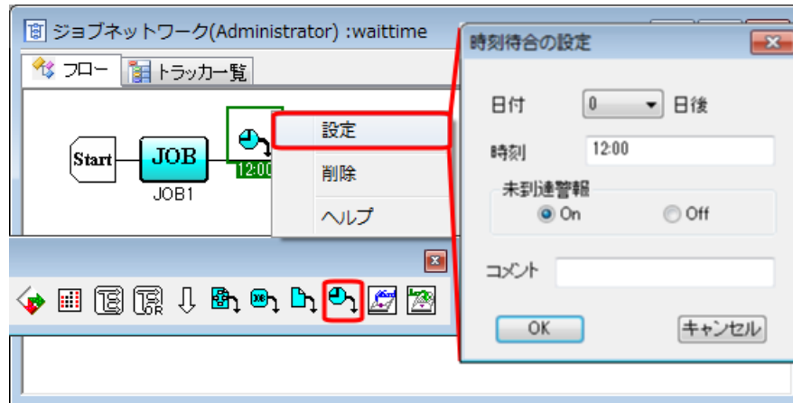
図4.23 時刻待ち合わせの設定画面例
