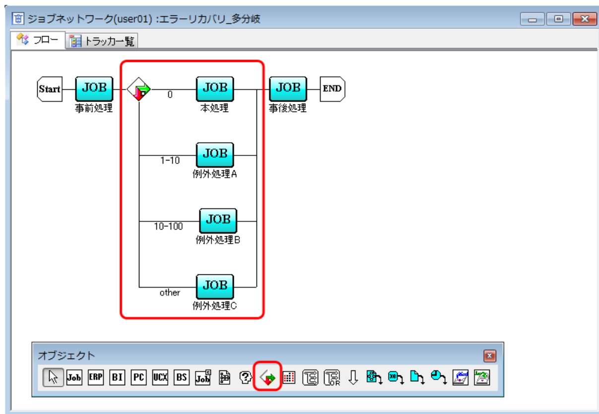
図4.14 条件分岐の配置画面例
