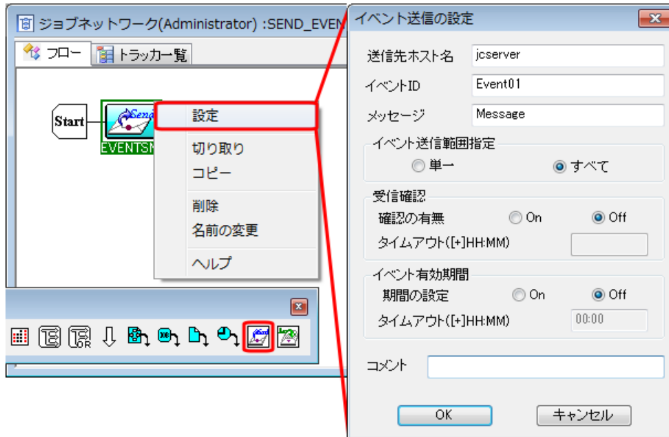
図4.27 イベント送信の設定画面例
