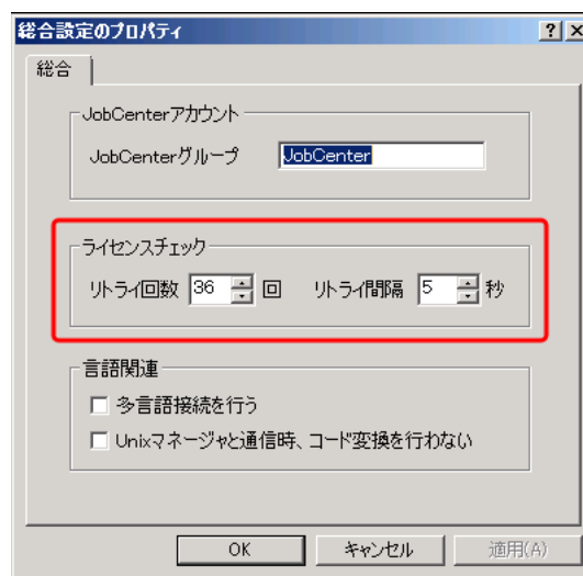
図5.2 ライセンスチェック設定画面
