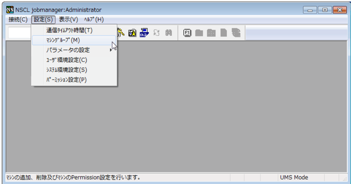
図3.4 メニューバー「設定」－「マシングループ」選択画面例
