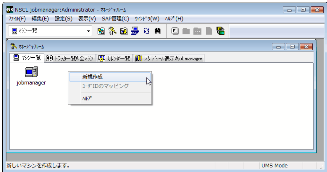
図3.1 マシン一覧へのマシン追加画面例（標準リモートマシン構成機能）
