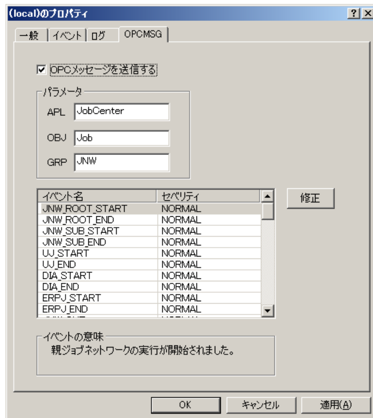
図11.20 [詳細設定] ダイアログ [OPCMMSG] 画面例
