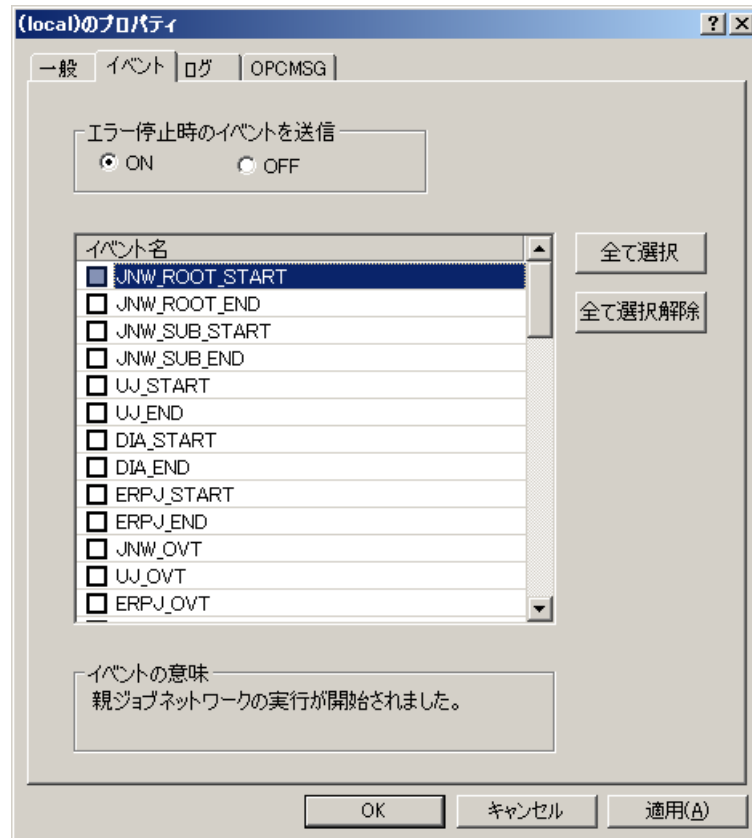
図11.15 イベントタブの画面例
