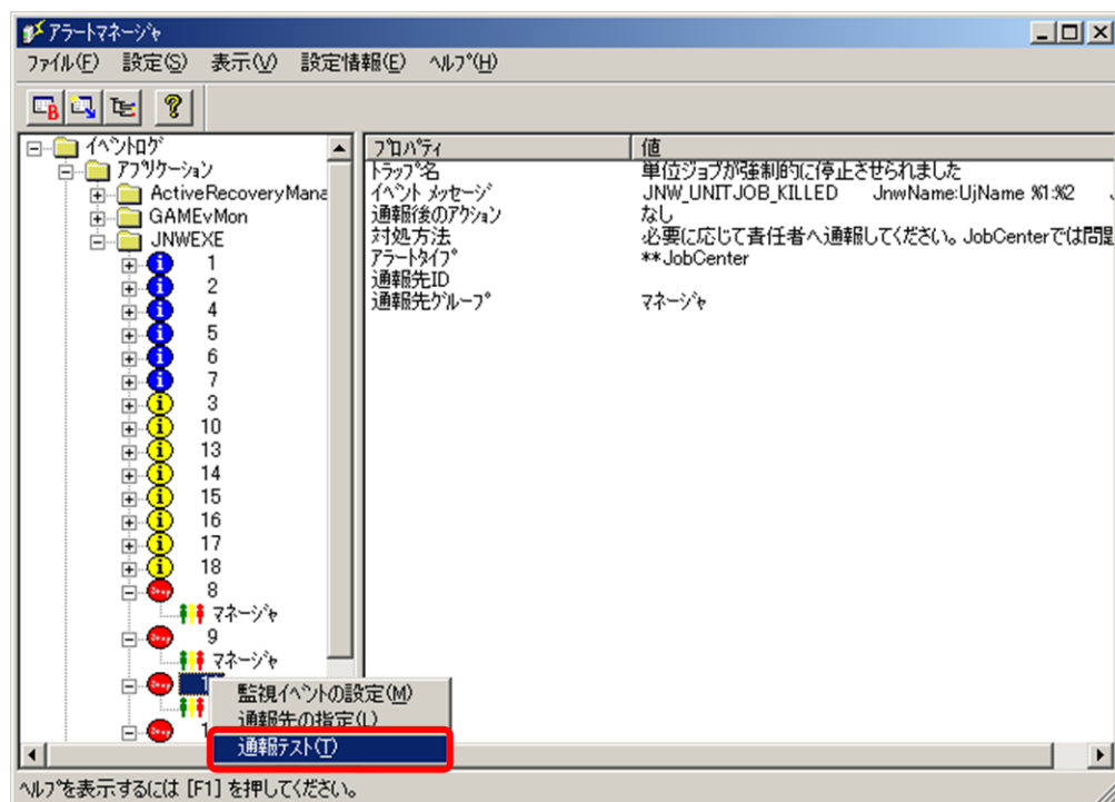
図11.11 [アラートマネージャ] ウィンドウ画面例
