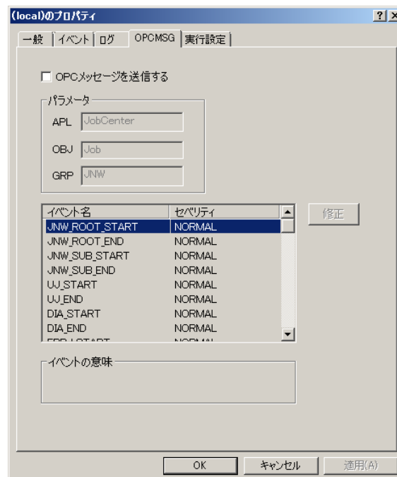
図12.8 OPCMSGタブの画面例
