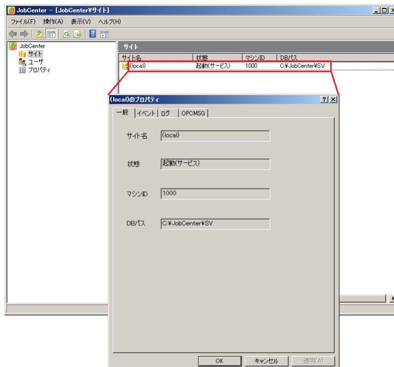
図12.4 サイトのプロパティ画面例
