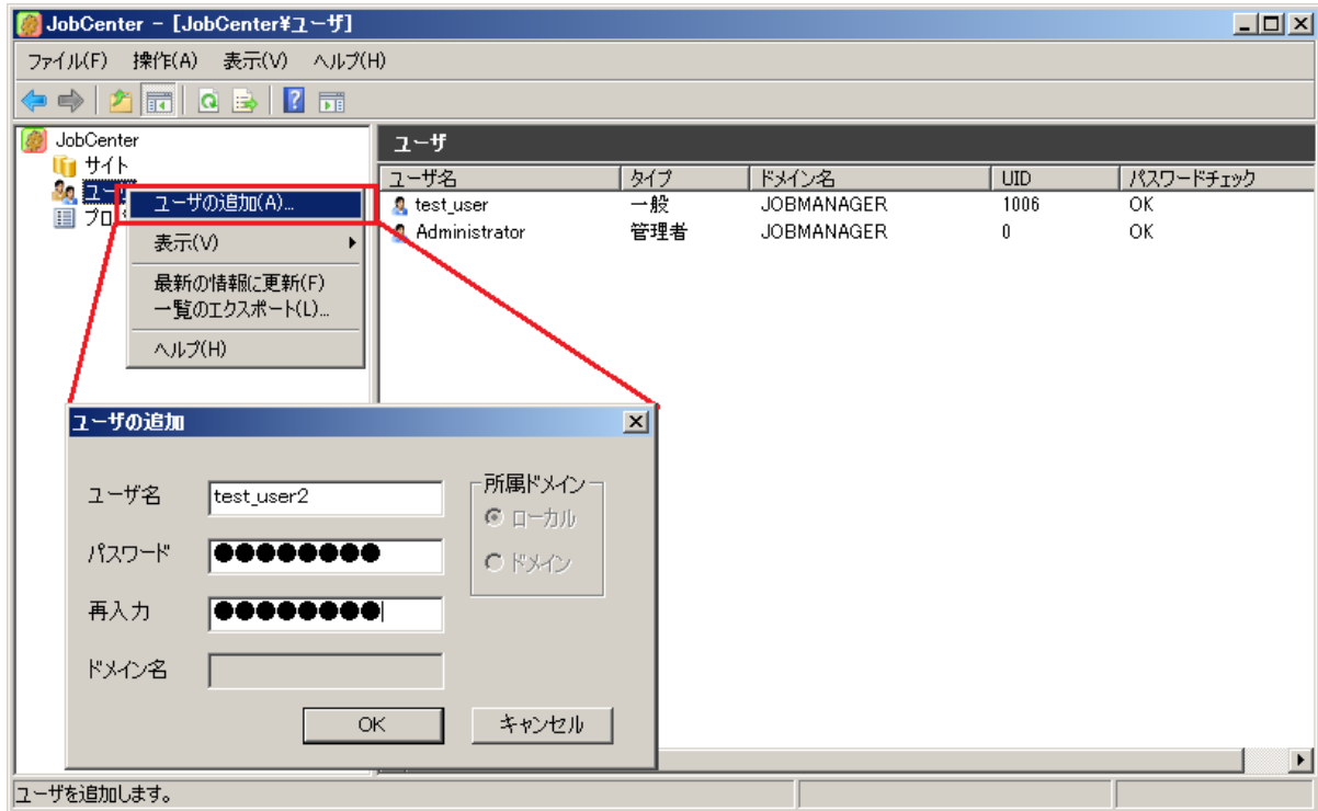
図12.17 ユーザの追加画面例
