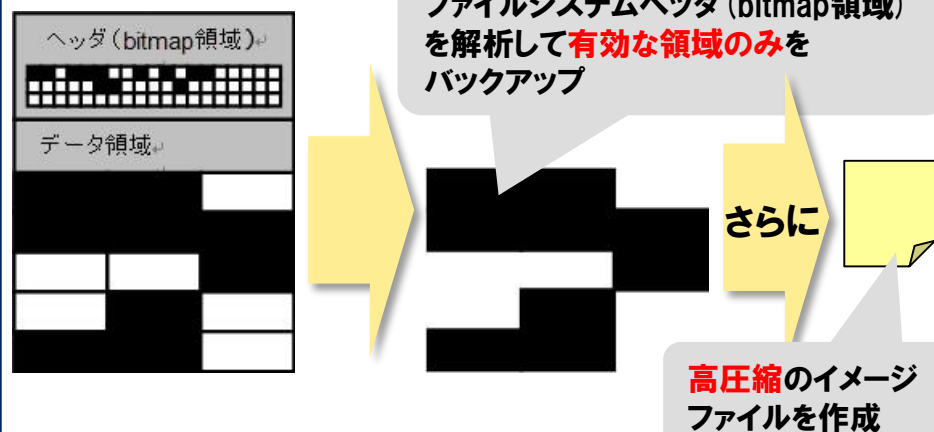
【有効セクタバックアップのイメージ図】
