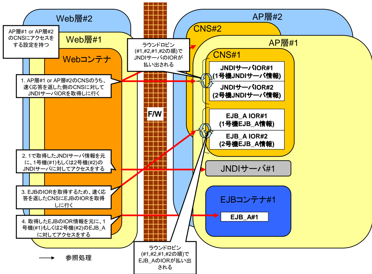
図 2.10.7 キャッシュ名前サーバ(正常稼動)
