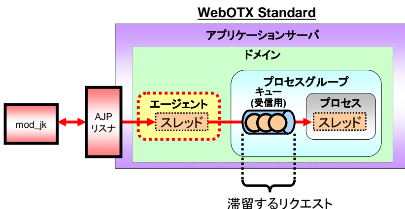
図 2.2.10.プロセスグループ構成
