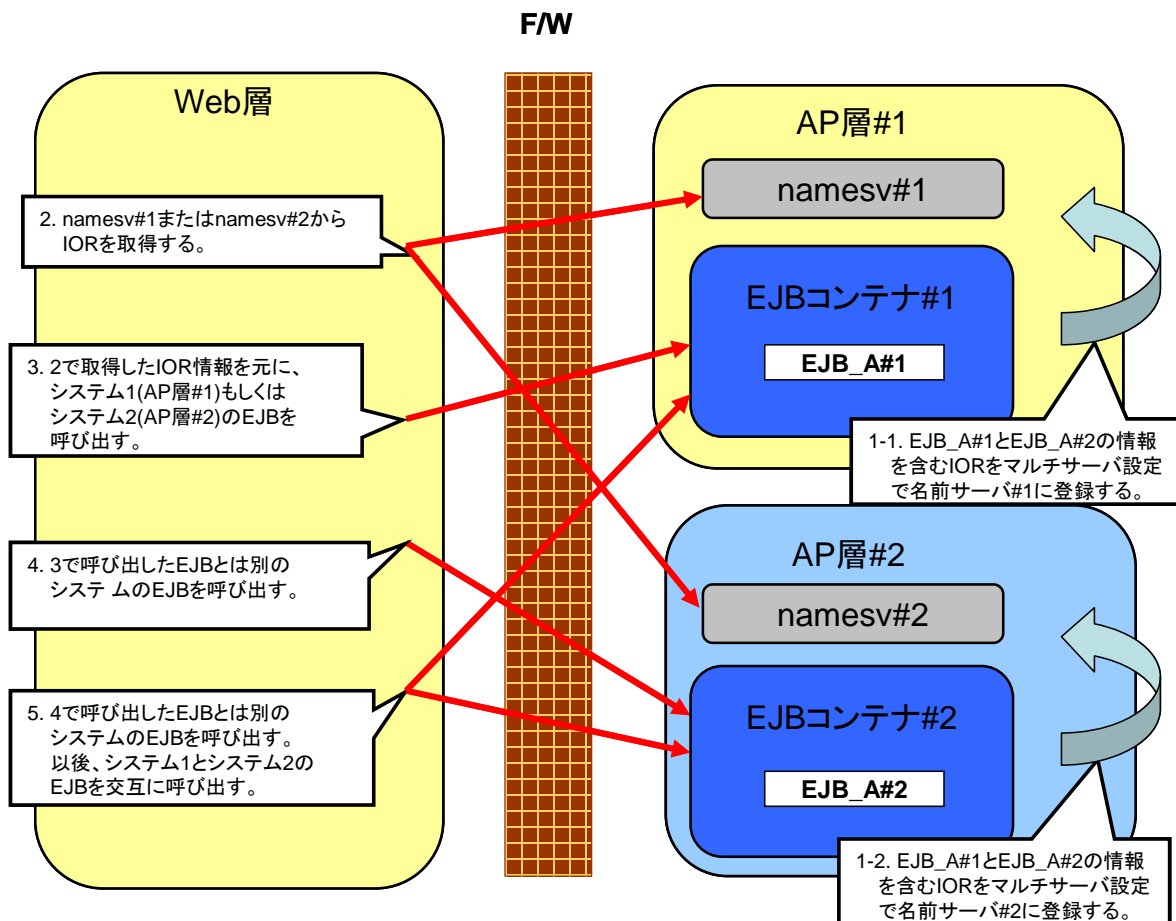
図 2.10.3 マルチサーババウンドロビン負荷分散運用(通常動作時)
