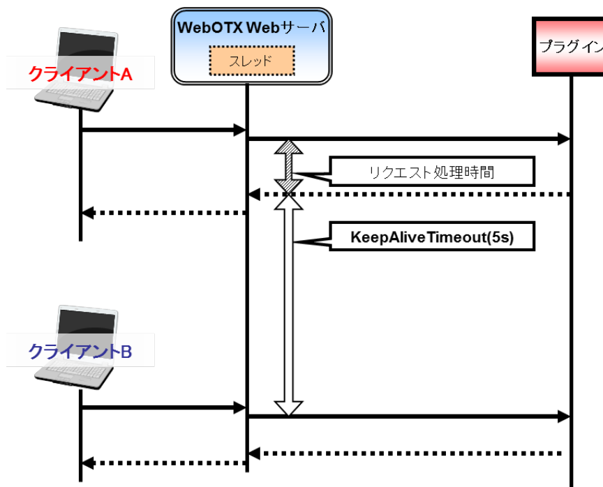
図 2.3.4.キープアライブタイムアウト
