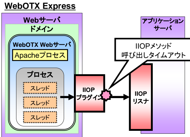
図 2.3.5.Web サーバとアプリケーションの通信経路
