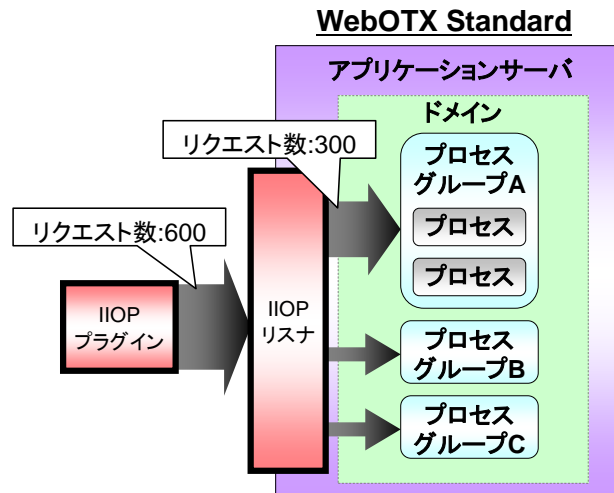
図 2.2.12.リクエスト経路
