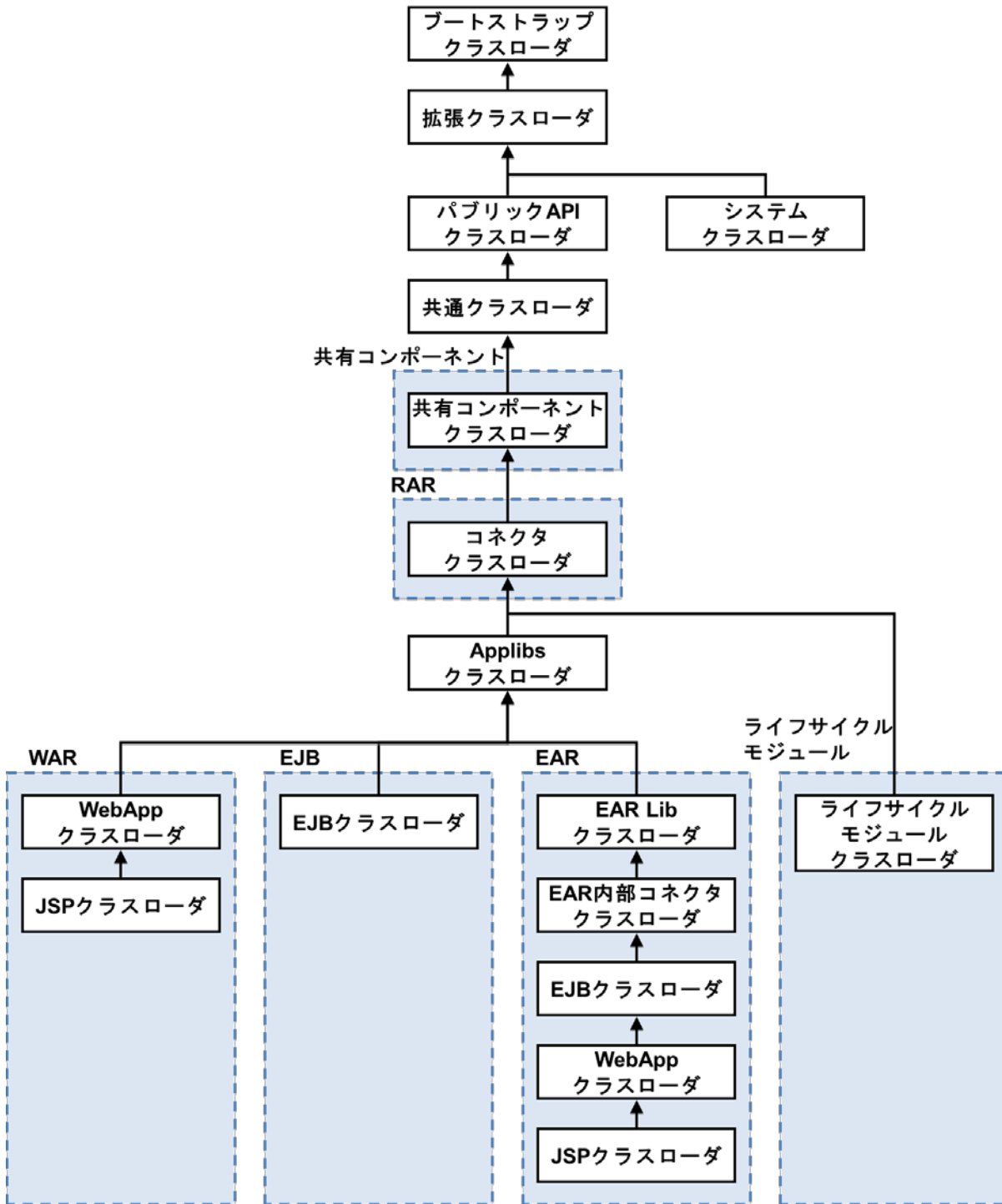
図 2.9.1.クラスローダ階層構造
