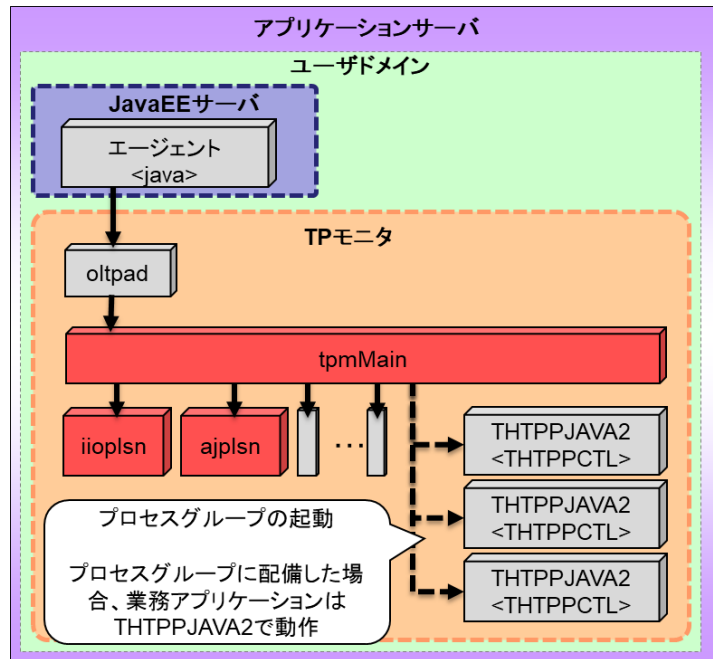
図 2.8.2.TP モニタ内監視プロセス
