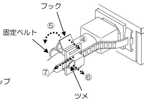
取り外すとき
