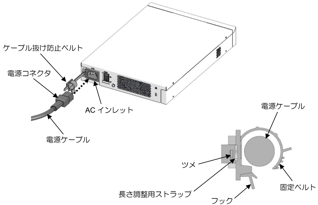
ケーブル抜け防止ベルト(断面図)
