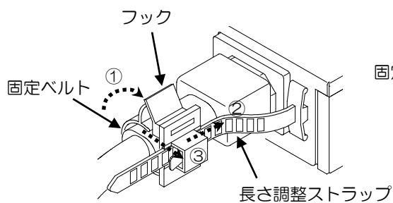
締め付けるとき
