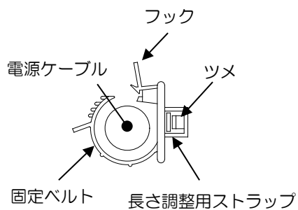
ケーブル抜け防止ベルト(断面図)
