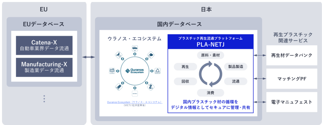
図 50：各データスペースの位置づけ
