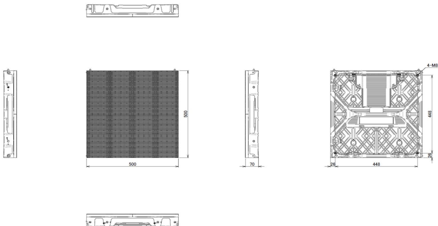
寸法図 (単位:mm)
