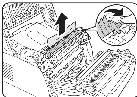
定着ユニットでの紙づまり → 75 ページ
