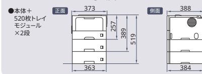
MultiWriter 4M350 寸法図 (単位:mm)
