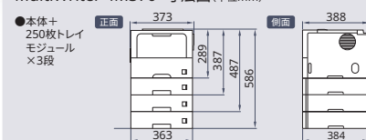
MultiWriter 4M350 寸法図 (単位:mm)
