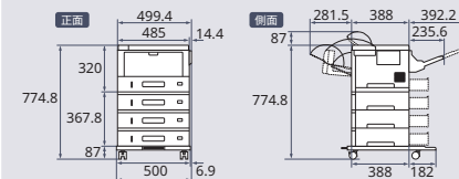
MultiWriter 3M570 寸法図(単位:mm)
