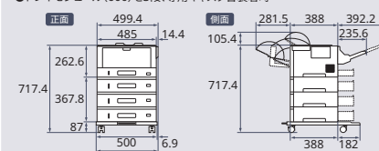
MultiWriter 3M550/3M530 寸法図(単位:mm)
