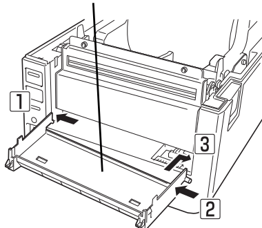
フロントカバー（カッター）
