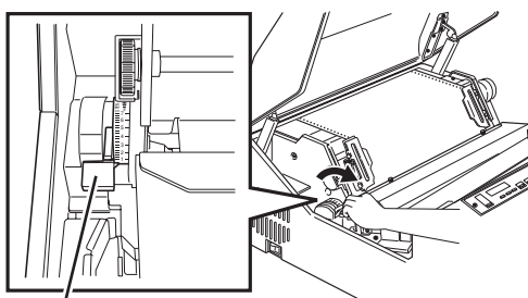
用紙厚セットレバー
