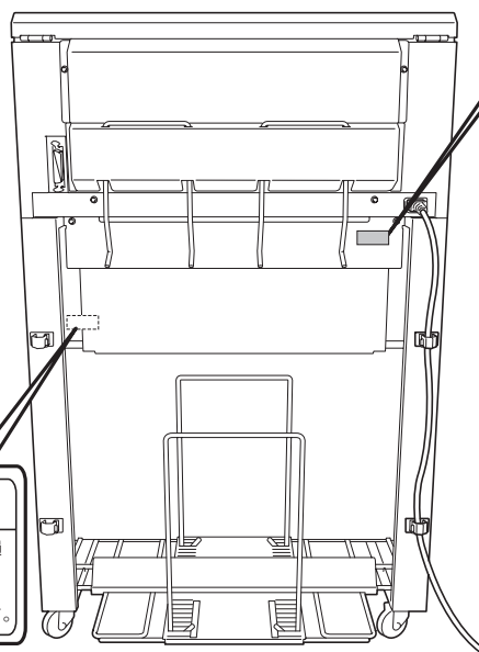
プリンタ背面
