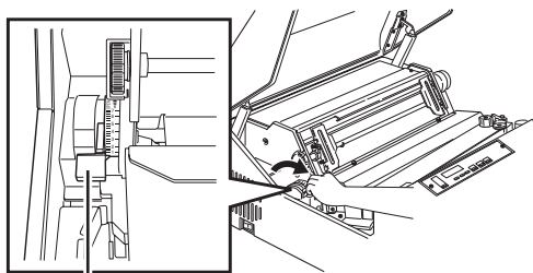
用紙厚セットレバー
