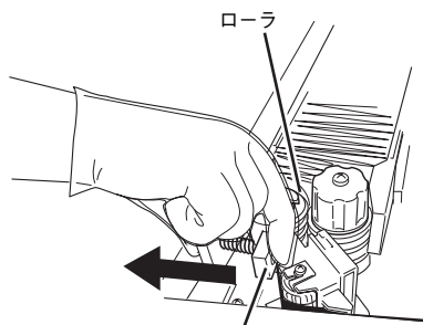
ローラオープンレバー
