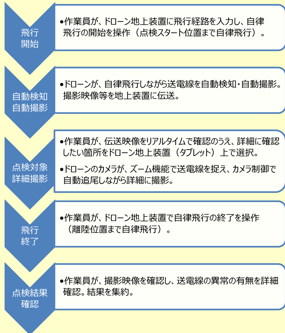
【図2】ドローンによる「送電線自動追尾点検」手順 (概要)
