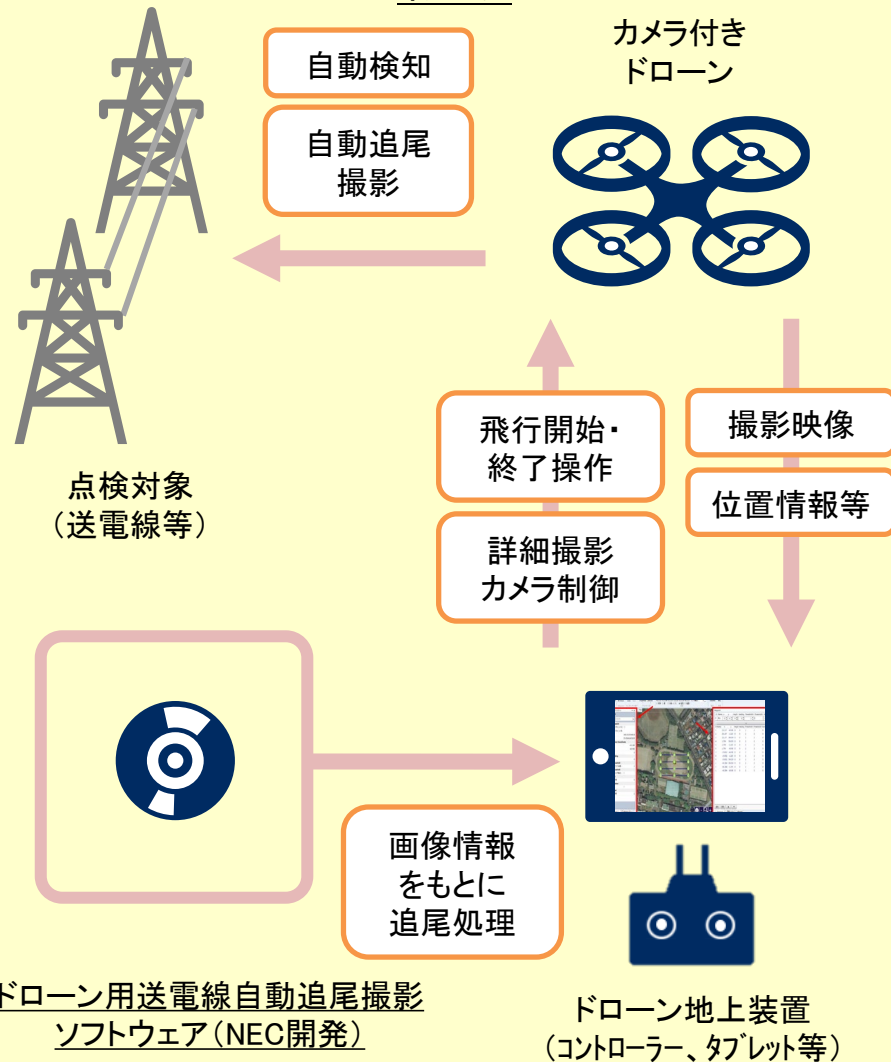
【図1】ドローンによる「送電線自動追尾点検」イメージ
