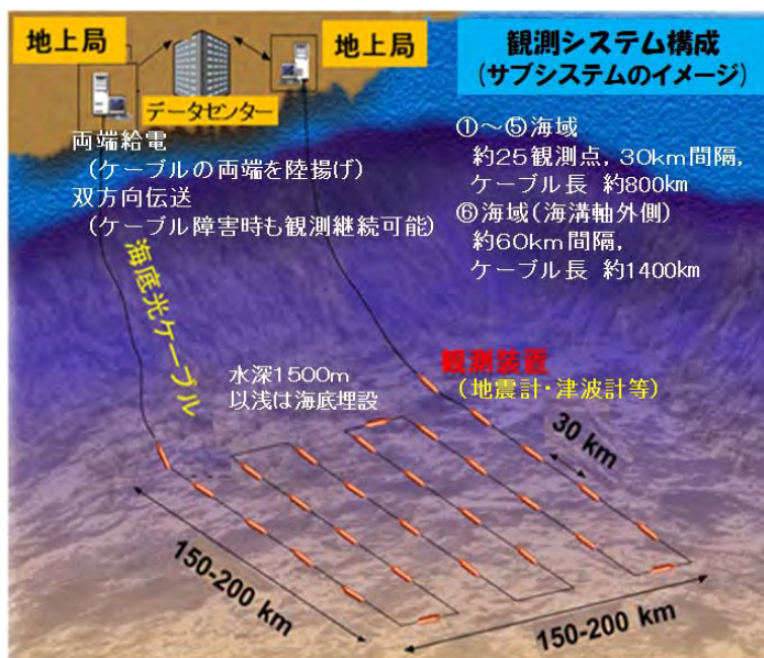
図2 観測システム(サブシステム)の構成。房総沖のシステムでは、南房総市と鹿嶋市に地上局が建設される。
