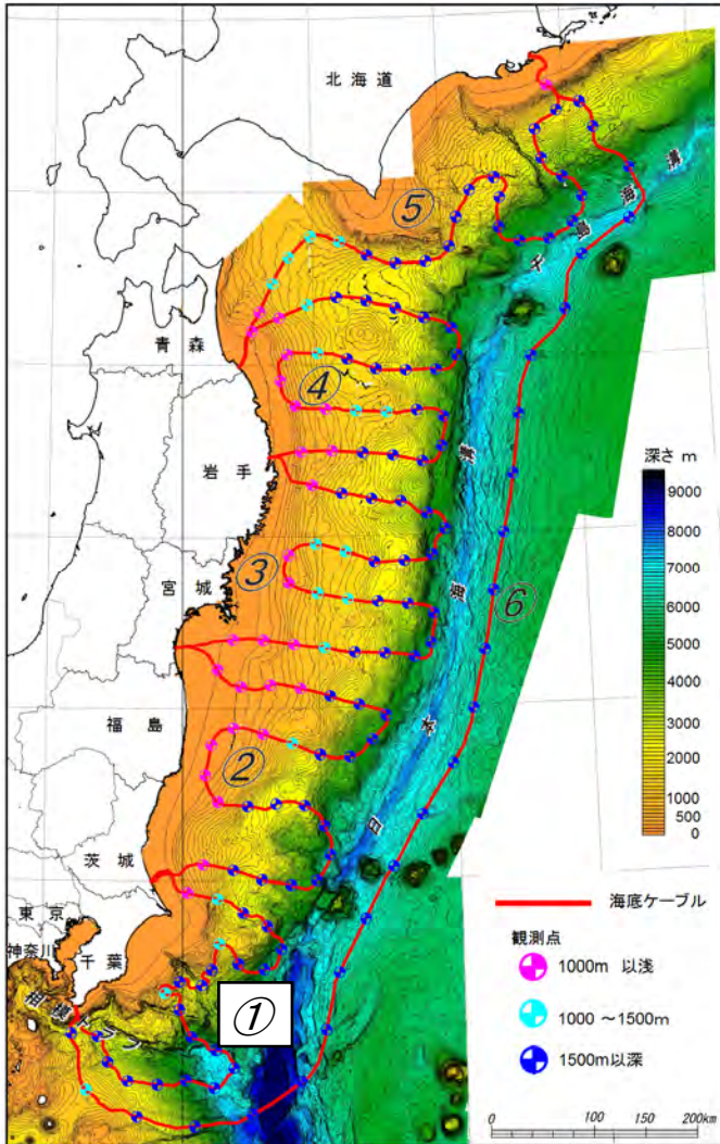
図1 日本海溝海底地震津波観測網の整備計画。今回、房総沖のサブシステム①のケーブル敷設を行う。
