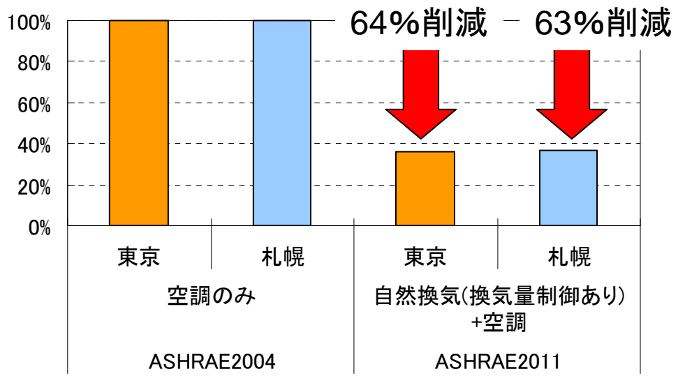
年間における空調エネルギーの消費量の比較（東京、札幌）
