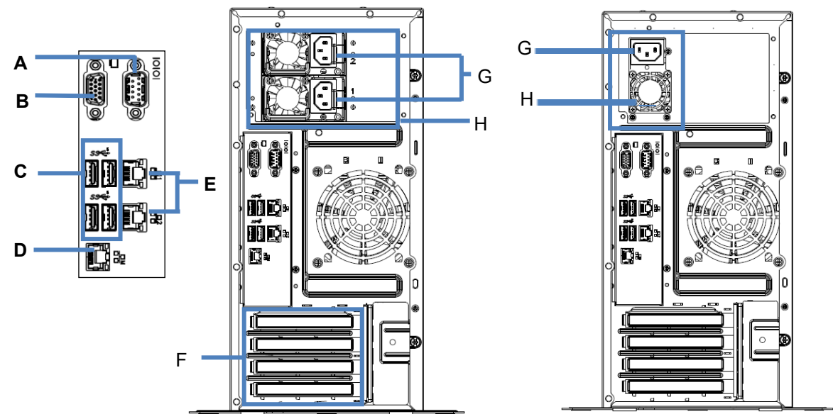
非冗長電源ユニット(N8181-177)搭載時
