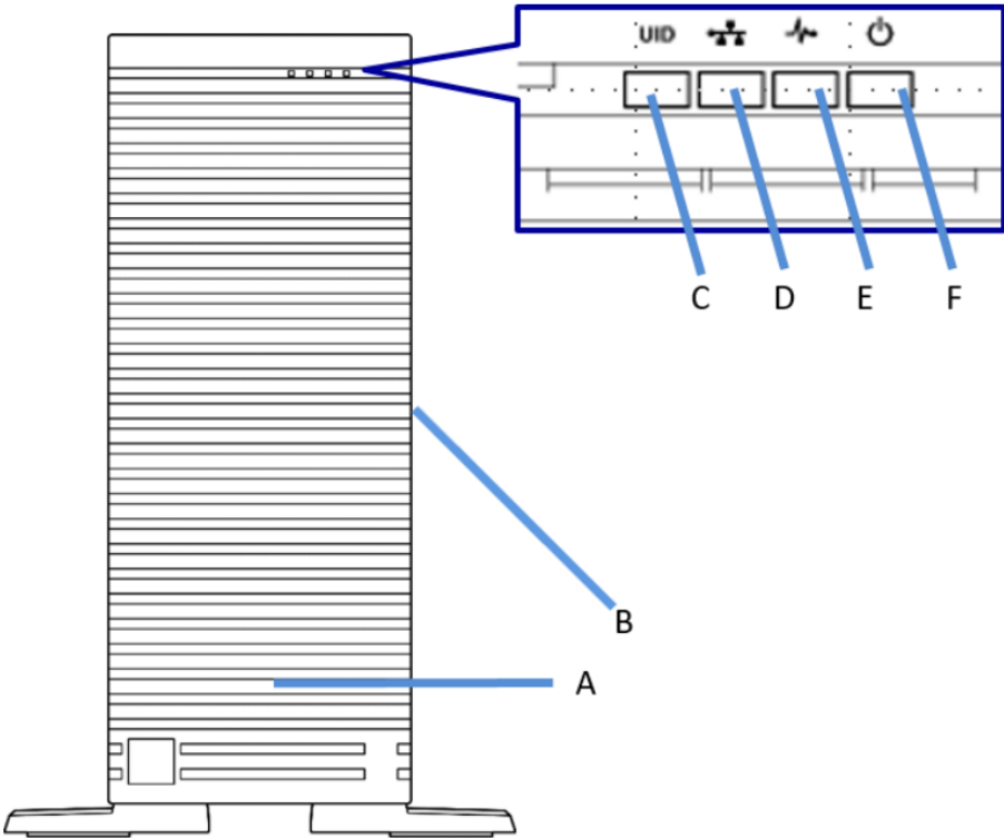
正面図 フロントベゼルを閉じた状態
