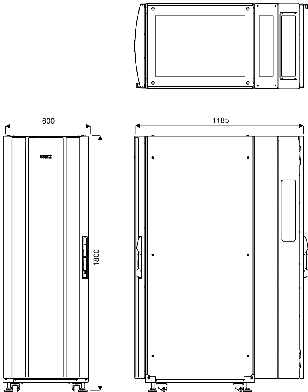
37U 三面図 (基本タイプ+奥行延長キット取り付け時)
