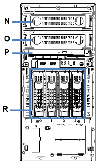
3.5 型 HDD ケージ(N8154-140)実装時
