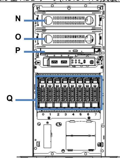
2.5 型 HDD ケージ(N8154-170)実装時
