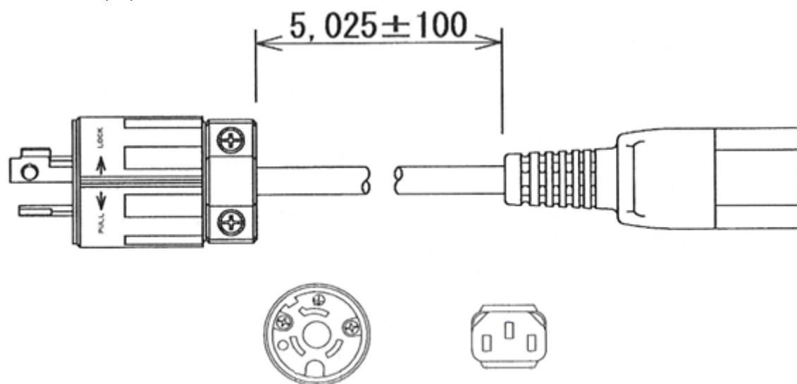
電源設備側 【プラグ形状 : NEMA L6-15P】
