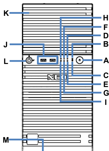
フロントベゼルを開いた状態 2.5 型 HDD ケージ(N8154-170)実装時
