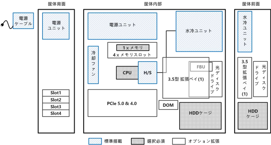
拡張スロット対応図
