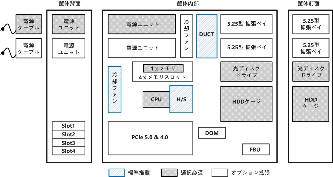
拡張スロット対応図
