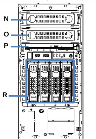
フロントベゼルを開いた状態 3.5 型 HDD ケージ(N8154-140)実装時
