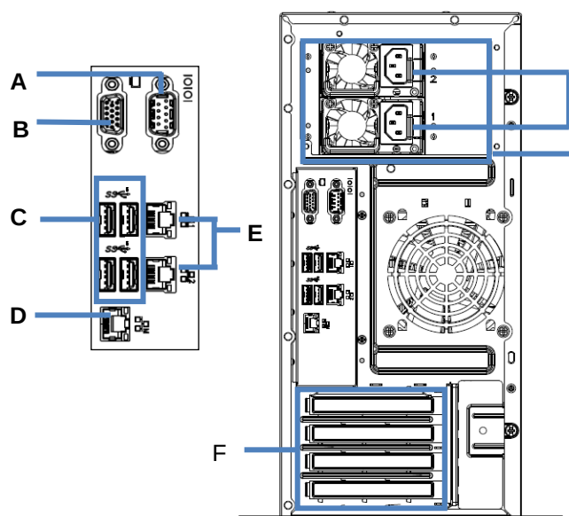
冗長電源ユニット(N8181-183/-184)搭載時
