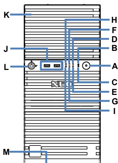
フロントベゼルを開いた状態 3.5 型 HDD ケージ(N8154-140)実装時
